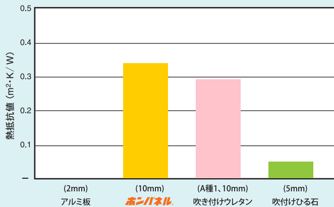
各種材料の熱抵抗 ※数値が大きいほど熱を通さない
