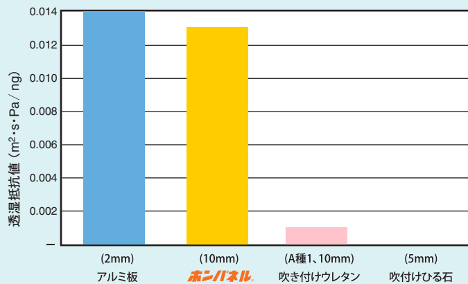
各種材料の透湿抵抗 ※数値が大きいほど湿気を通さない
