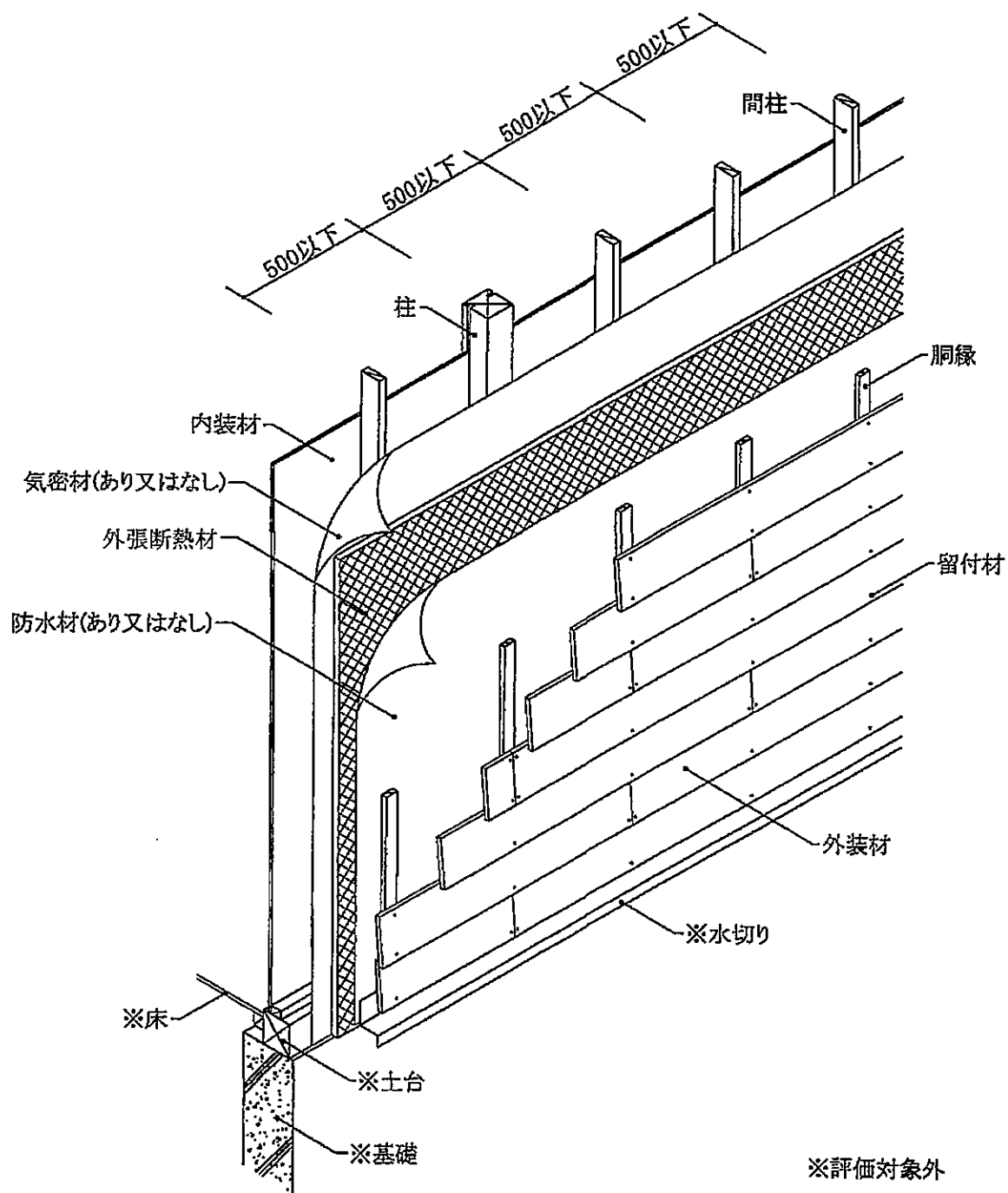
透視図
