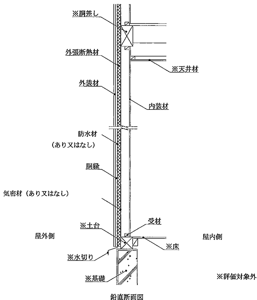
図24 施工図
