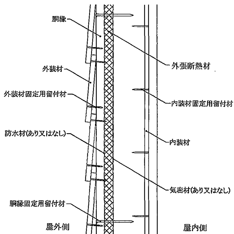
鉛直断面図
