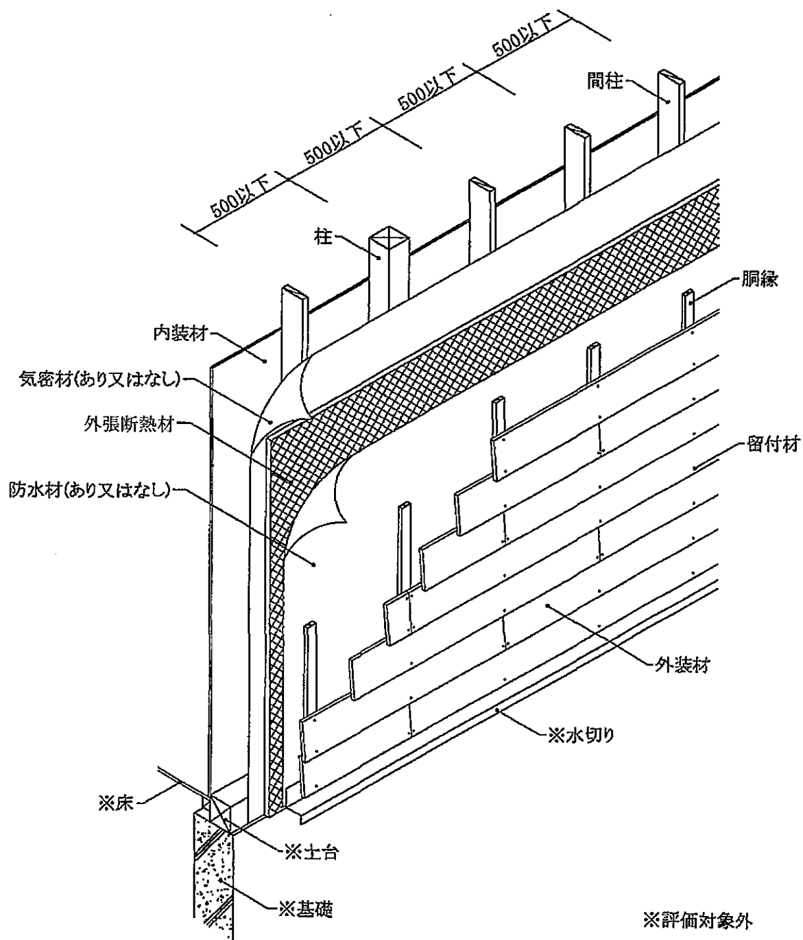
透視図
