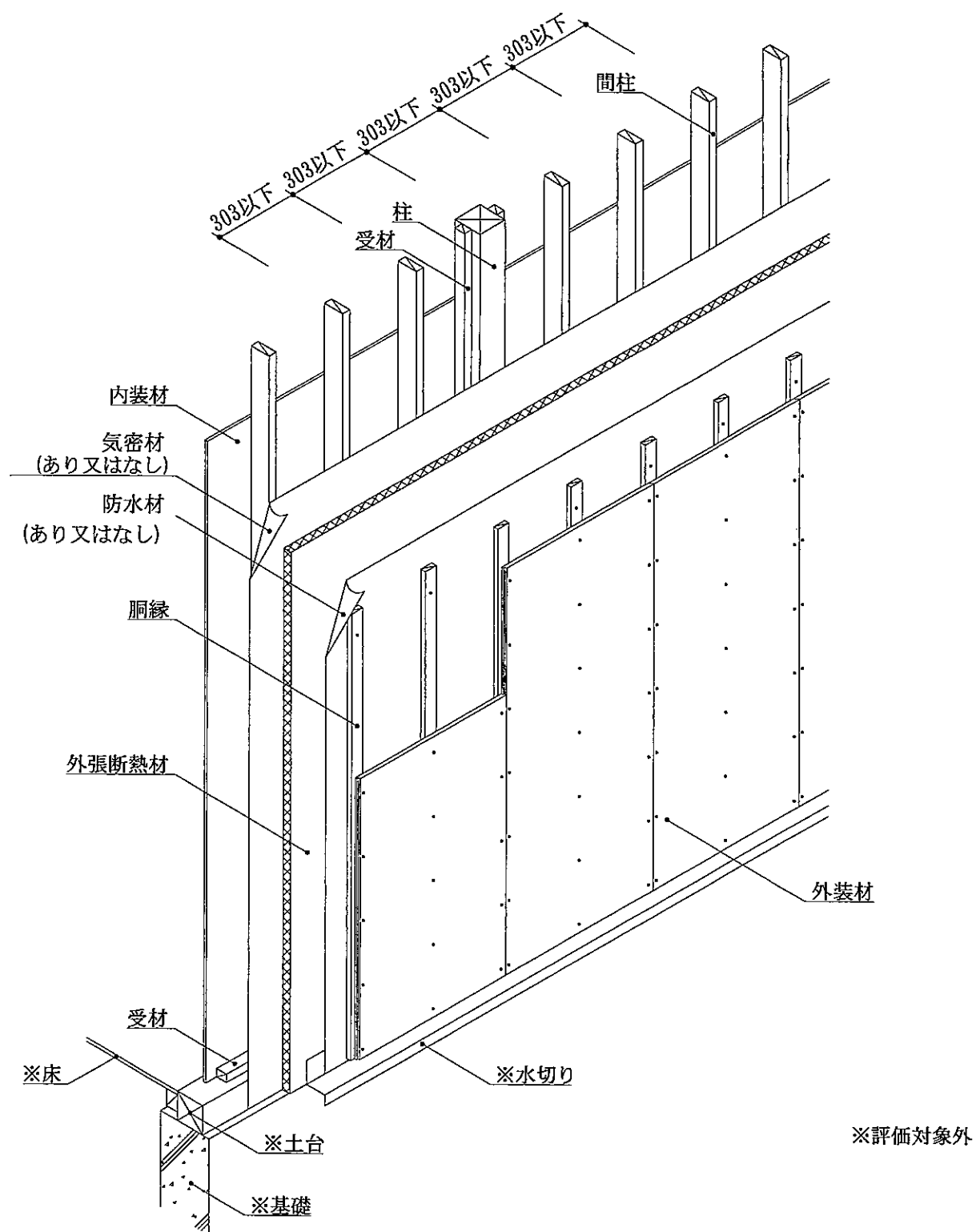
図11 構造説明図
