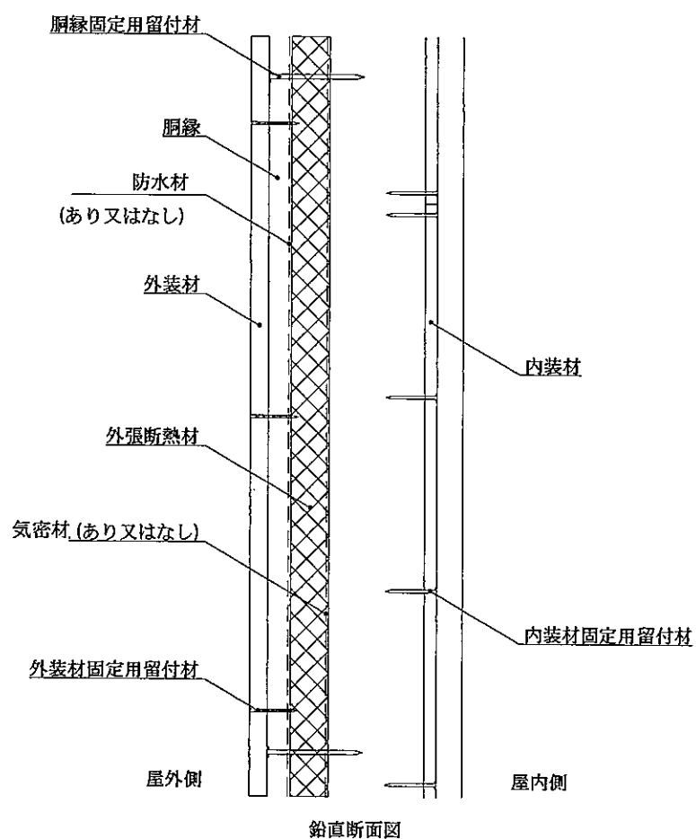
図6 構造説明図
