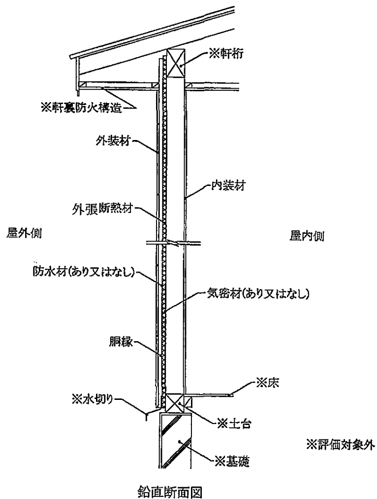
図28 施工図 (外装材横張・大壁造／充てん断熱材なし・構造用面材なし・下張材なし)
