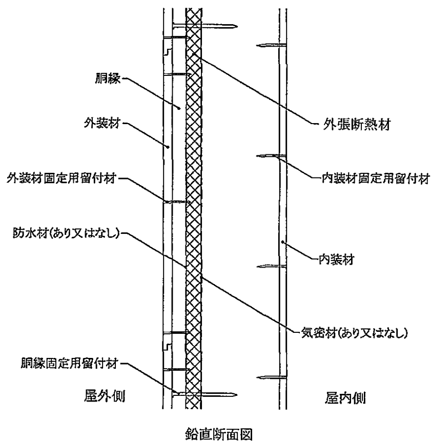
図14 構造説明図
