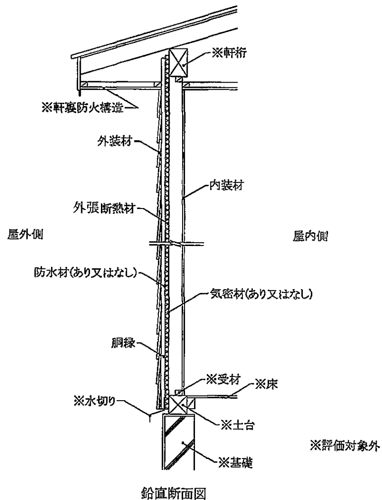
図23 施工図 (外装材横張・欠き込み真壁造／充てん断熱材なし・構造用面材なし・下張材なし)
