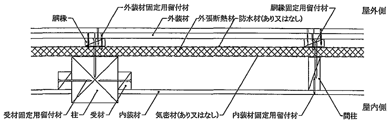
水平断面図
