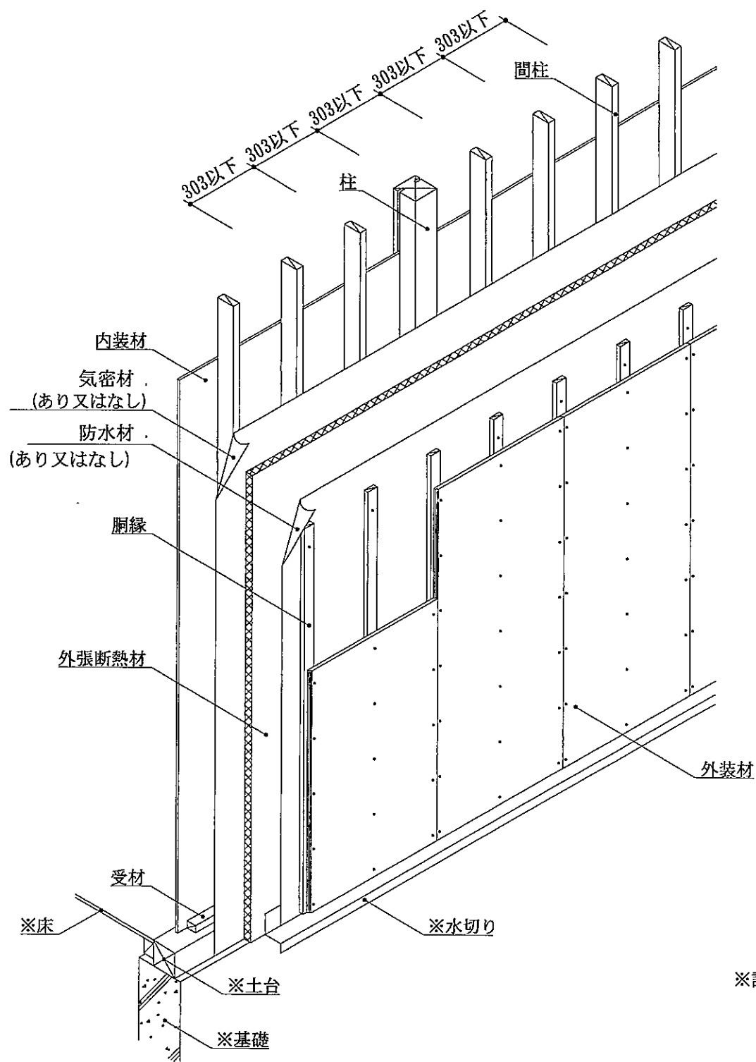
図5 構造説明図 (外装材縦張・欠き込み真壁造／充てん断熱材なし・構造用面材なし・下張材なし)
