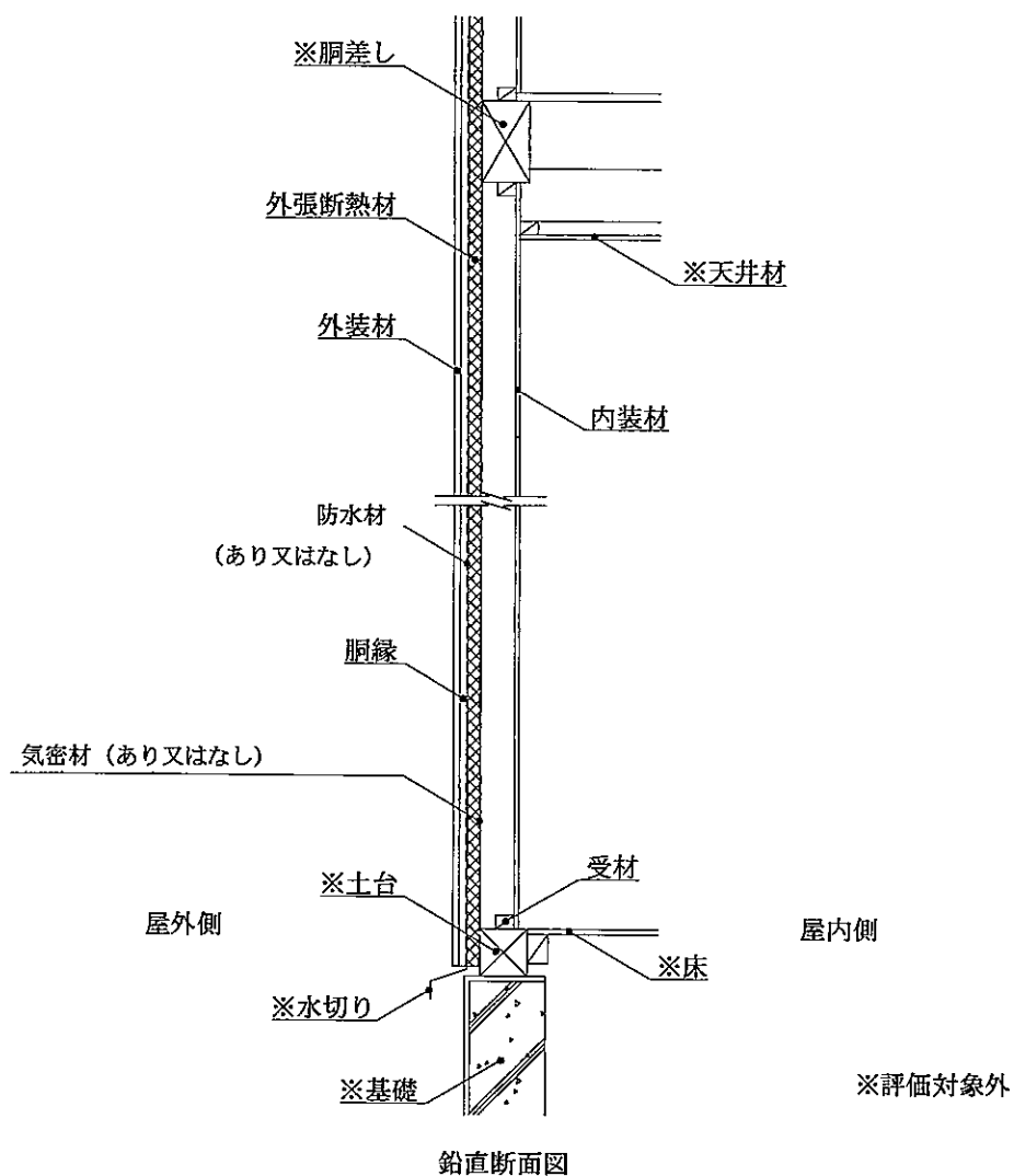
図27 施工図
