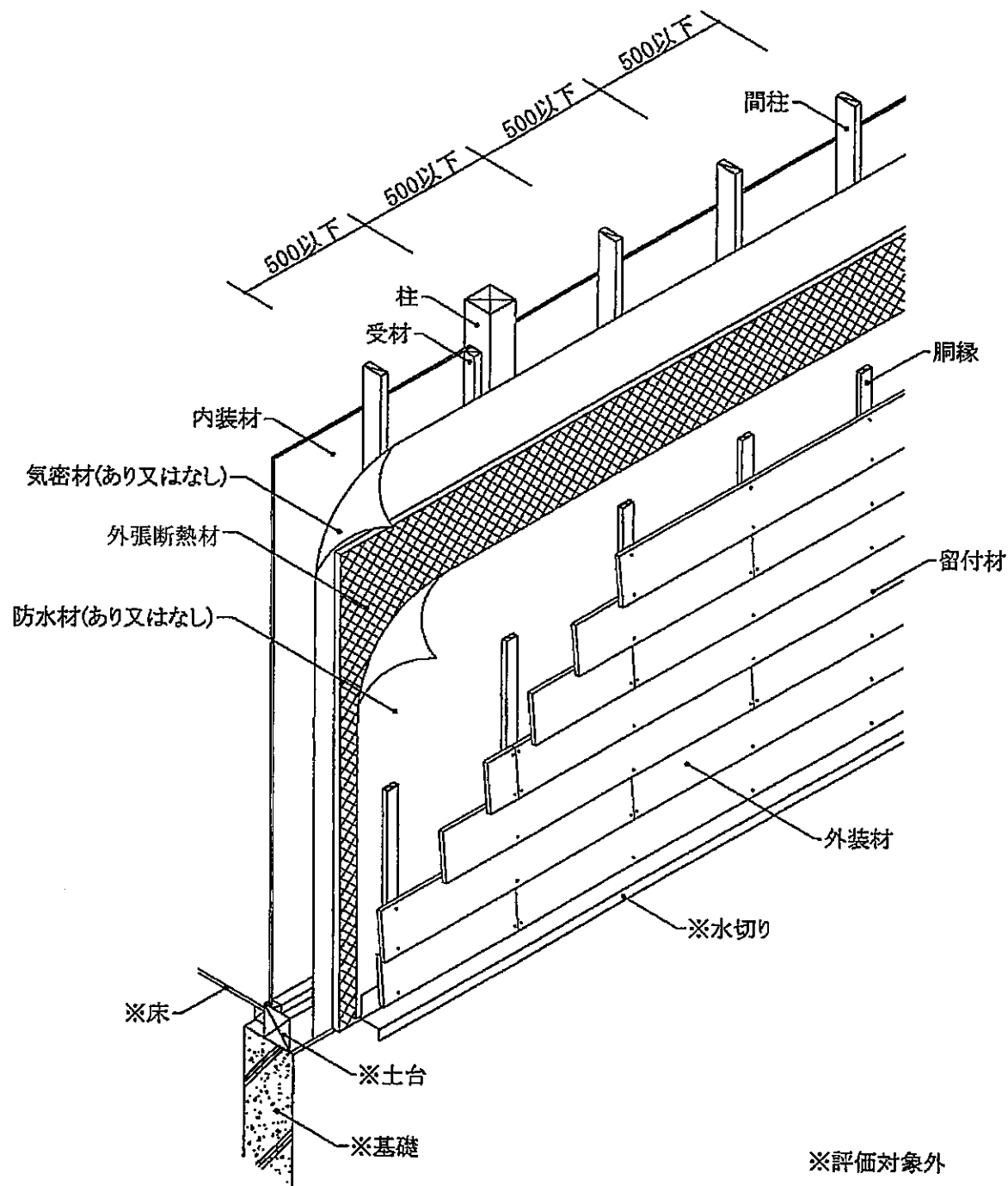
透視図
