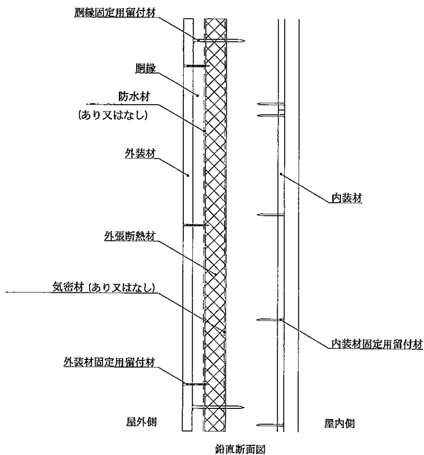
図12 構造説明図 (外装材横張・受材真壁造／充てん断熱材なし・構造用面材なし・下張材なし)
