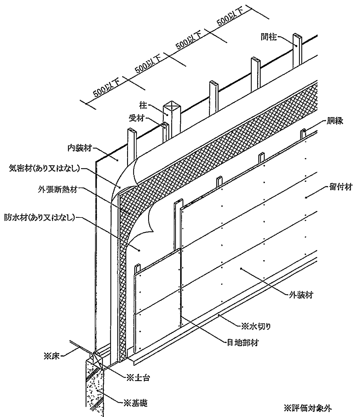
透視図
