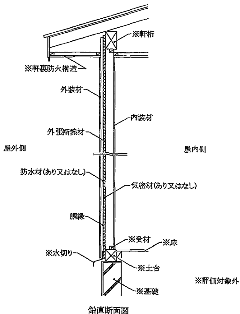
図25 施工図 (外装材横張・受材真壁造／充てん断熱材なし・構造用面材なし・下張材なし)
