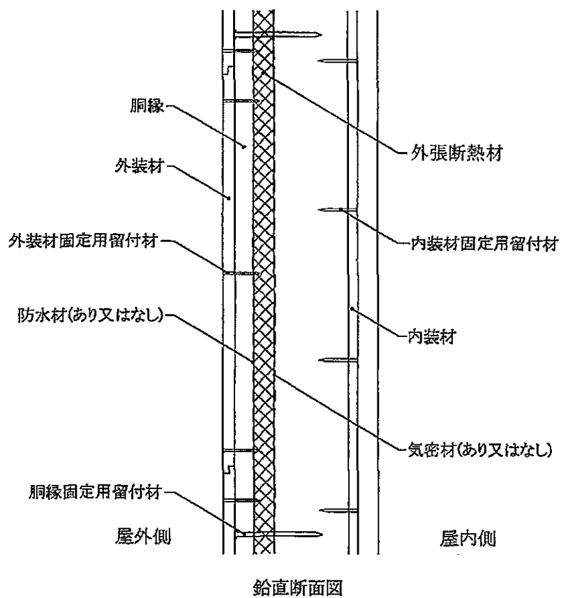
図2 構造説明図 (外装材横張・欠き込み真壁造／充てん断熱材なし・構造用面材なし・下張材なし)
