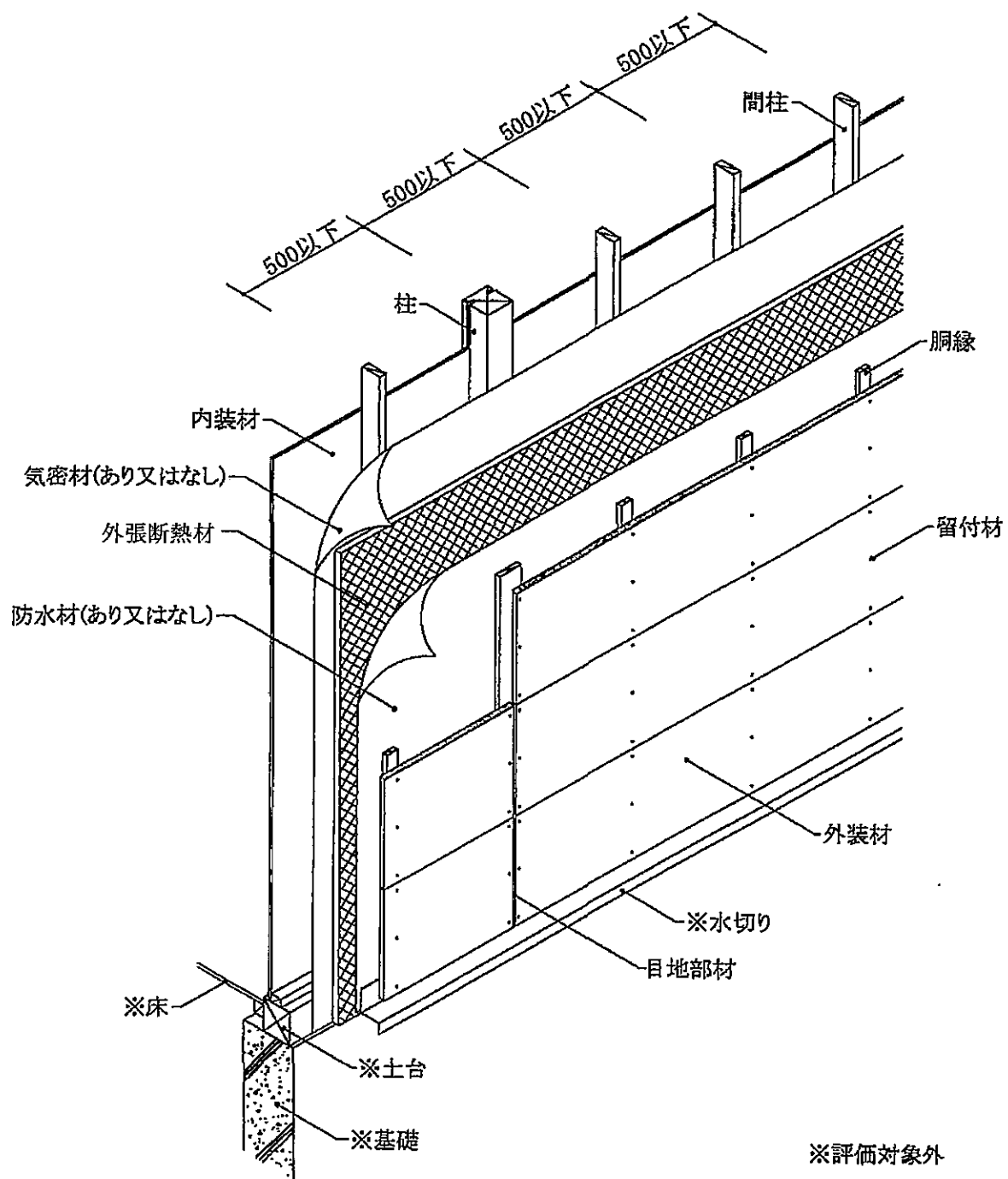
透視図
