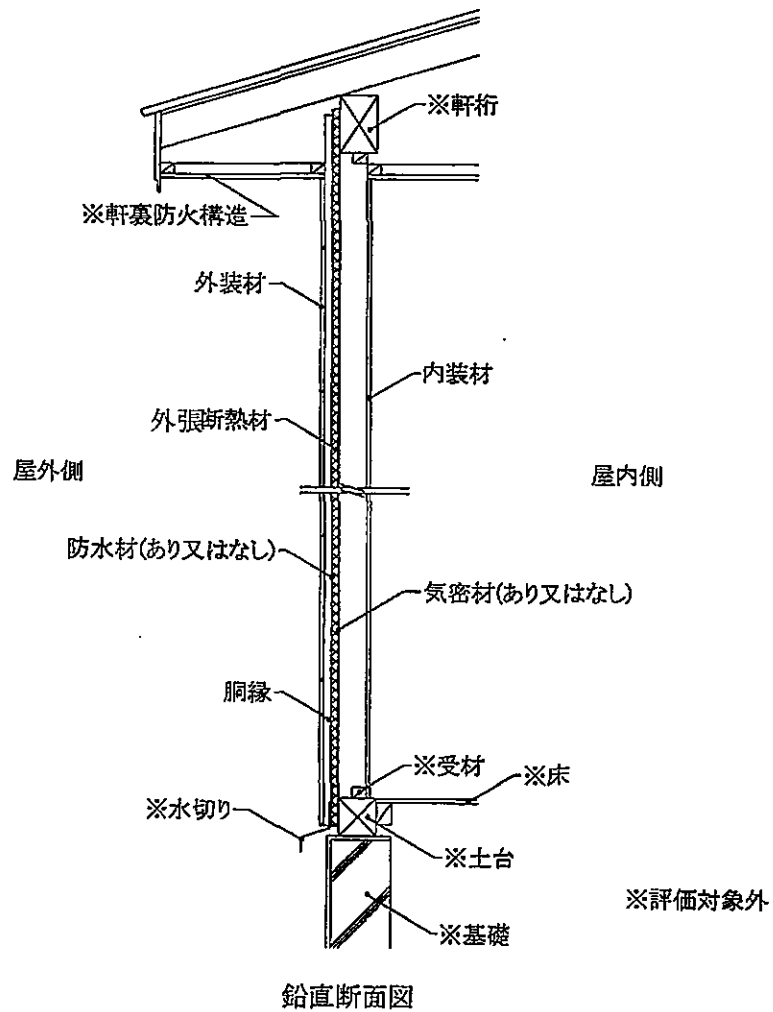
図22 施工図 (外装材横張・欠き込み真壁造／充てん断熱材なし・構造用面材なし・下張材なし)
