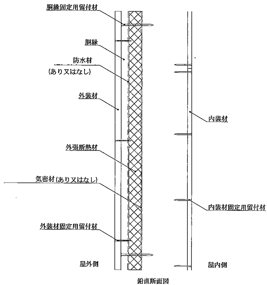
図18 構造説明図 (外装材横張・大壁造／充てん断熱材なし・構造用面材なし・下張材なし)
