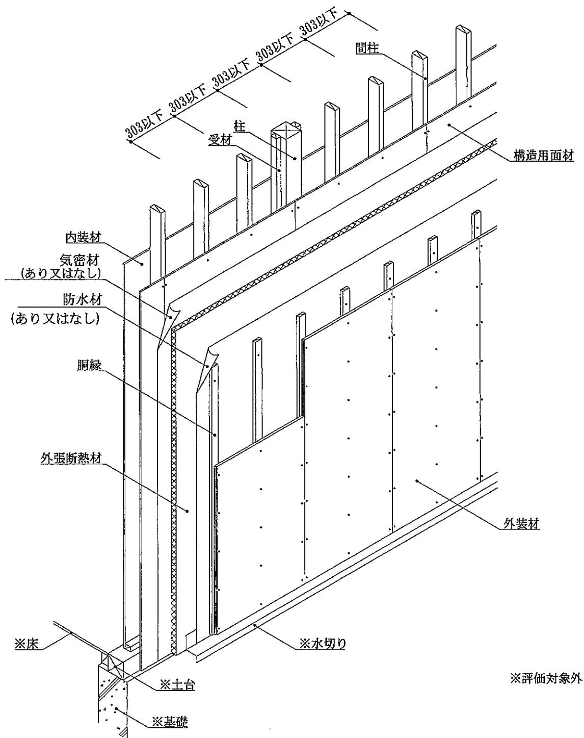
図11 構造説明図
