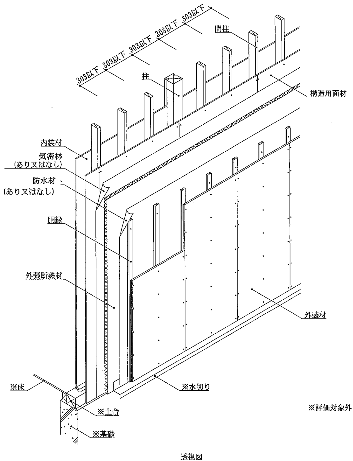
図5 構造説明図
