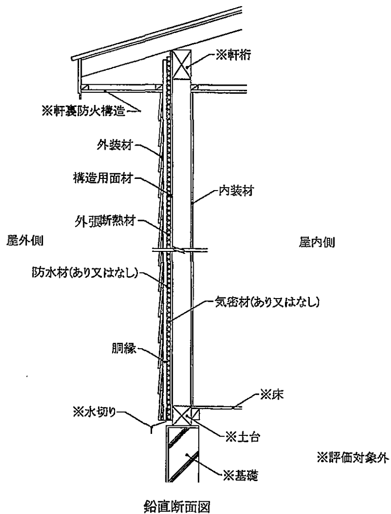
図29 施工図 (外装材横張・大壁造／充てん断熱材なし・構造用面材あり・下張材なし)
