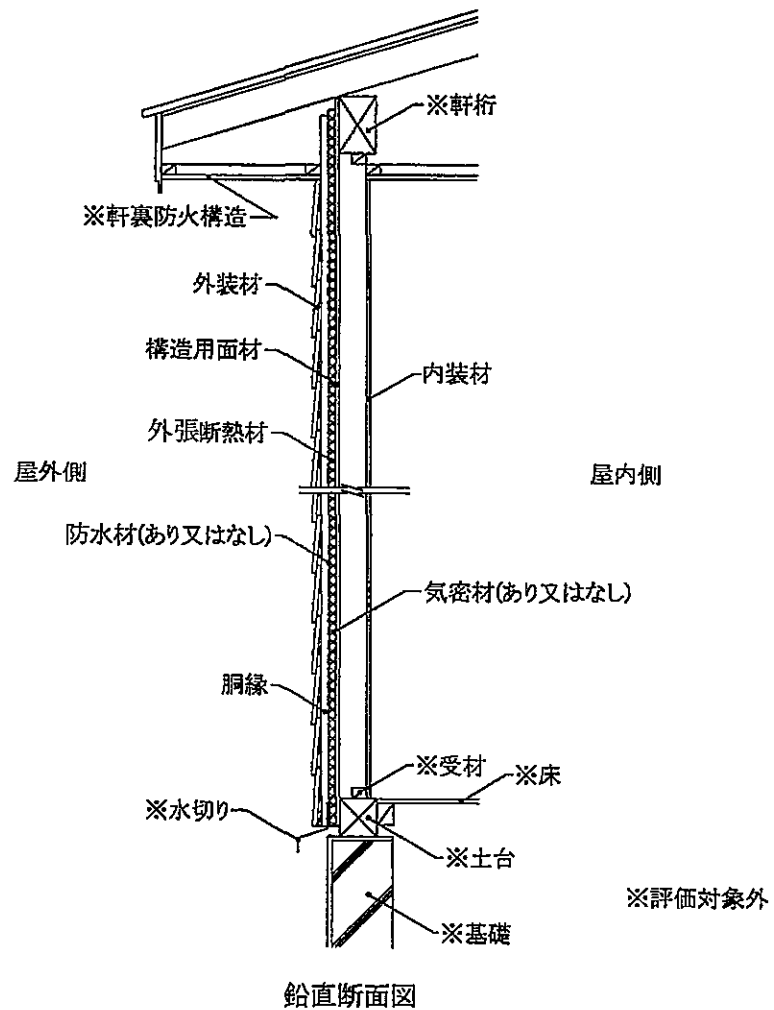
図26 施工図 (外装材横張・受材真壁造／充てん断熱材なし・構造用面材あり・下張材なし)
