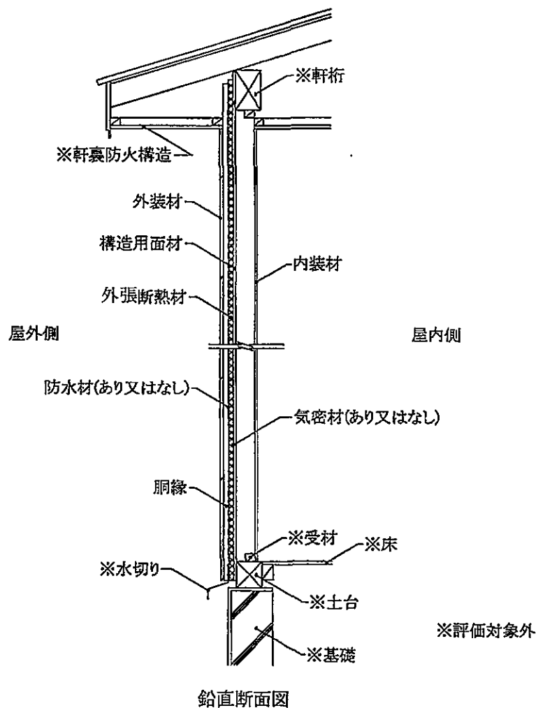
図22 施工図 (外装材横張・欠き込み真壁造／充てん断熱材なし・構造用面材あり・下張材なし)
