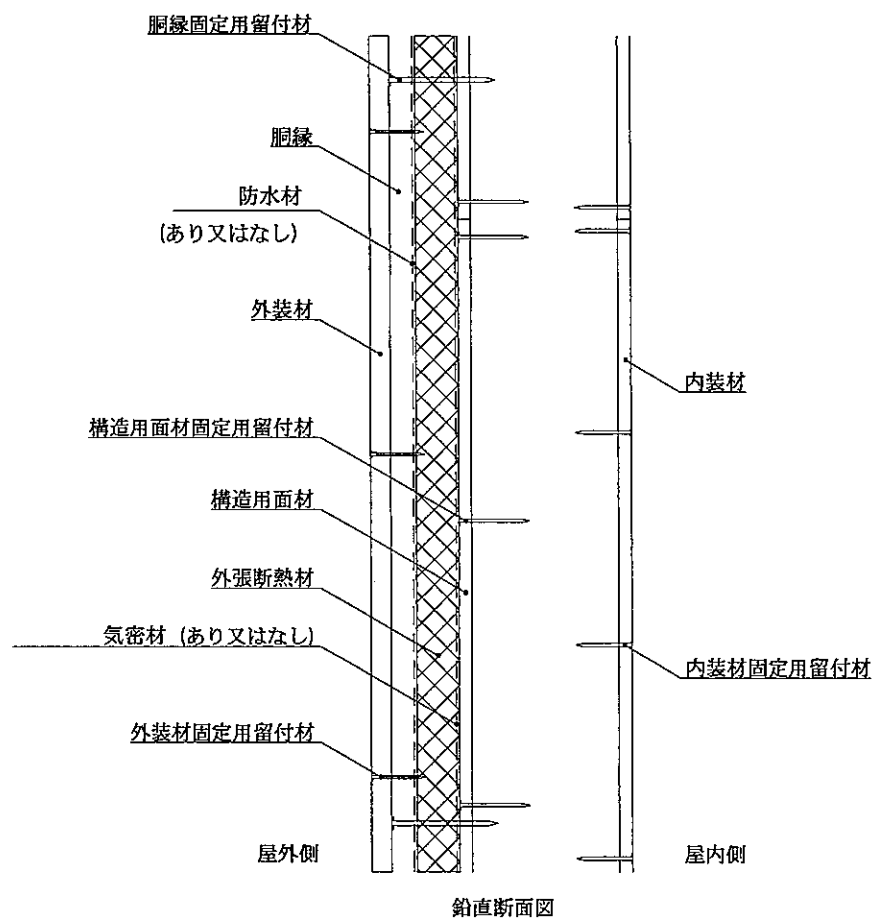
図18 構造説明図 (外装材縦張・大壁造／充てん断熱材なし・構造用面材あり・下張材なし)
