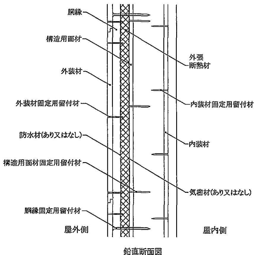
図2 構造説明図 (外装材横張・欠き込み真壁造／充てん断熱材なし・構造用面材あり・下張材なし)
