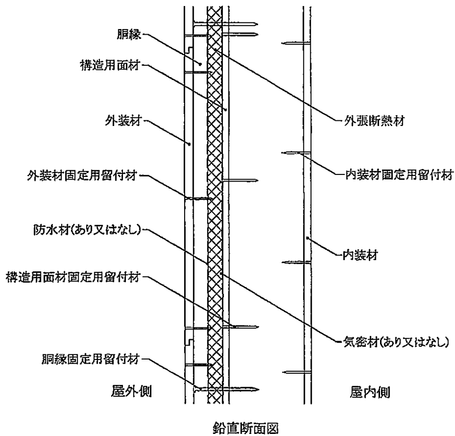
図14 構造説明図 (外装材横張・大壁造／充てん断熱材なし・構造用面材あり・下張材なし)
