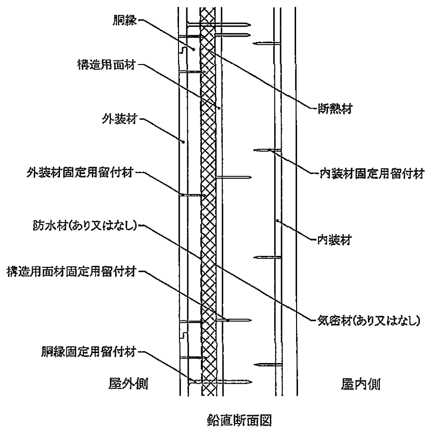
図8 構造説明図 (外装材横張・受材真壁造／充てん断熱材なし・構造用面材あり・下張材なし)
