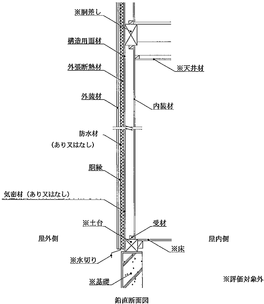
図24 施工図 (外装材縦張・欠き込み真壁造／充てん断熱材なし・構造用面材あり・下張材なし)
