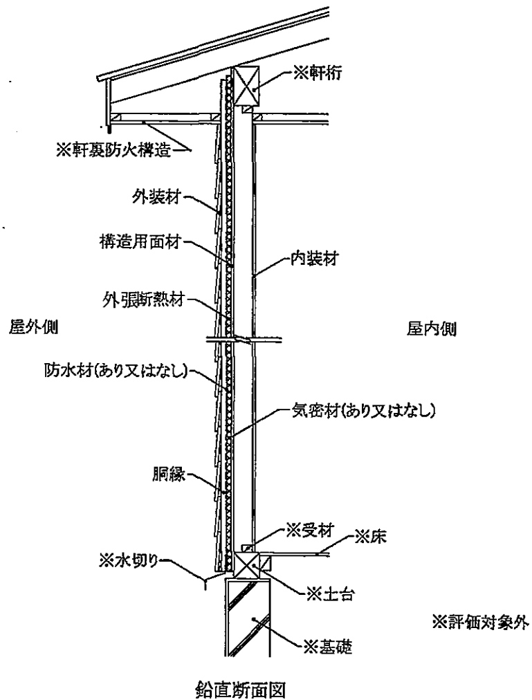
図23 施工図 (外装材横張・欠き込み真壁造／充てん断熱材なし・構造用面材あり・下張材なし)
