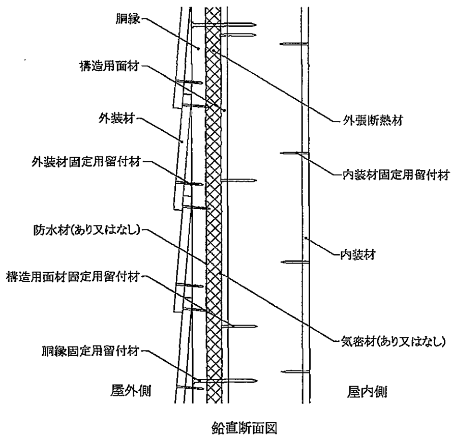
図16 構造説明図 (外装材横張・大壁造／充てん断熱材なし・構造用面材あり・下張材なし)
