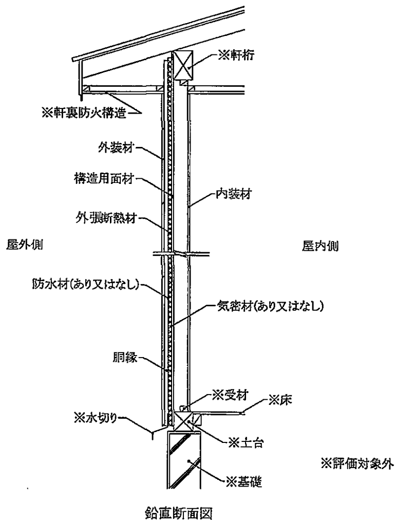
図25 施工図 (外装材横張・受材真壁造／充てん断熱材なし・構造用面材あり・下張材なし)
