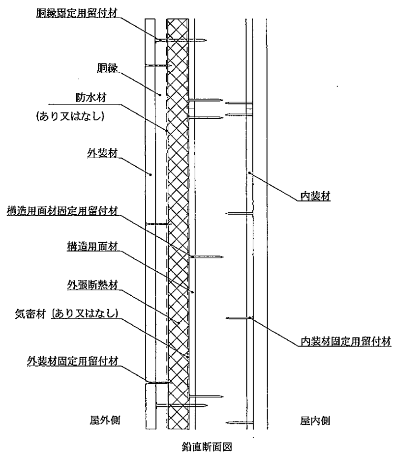
図6 構造説明図
