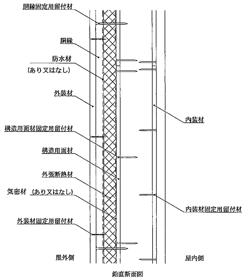
図12 構造説明図 (外装材縦張・受材真壁造／充てん断熱材なし・構造用面材あり・下張材なし)
