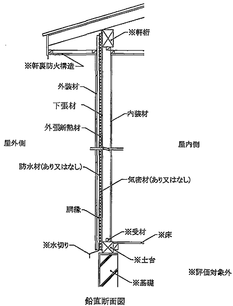
図25 施工図 (外装材横張・受材真壁造／充てん断熱材なし・構造用面材なし・下張材あり)
