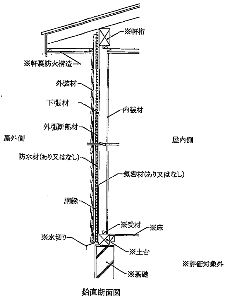
図23 施工図 (外装材横張・欠き込み真壁造／充てん断熱材なし・構造用面材なし・下張材あり)
