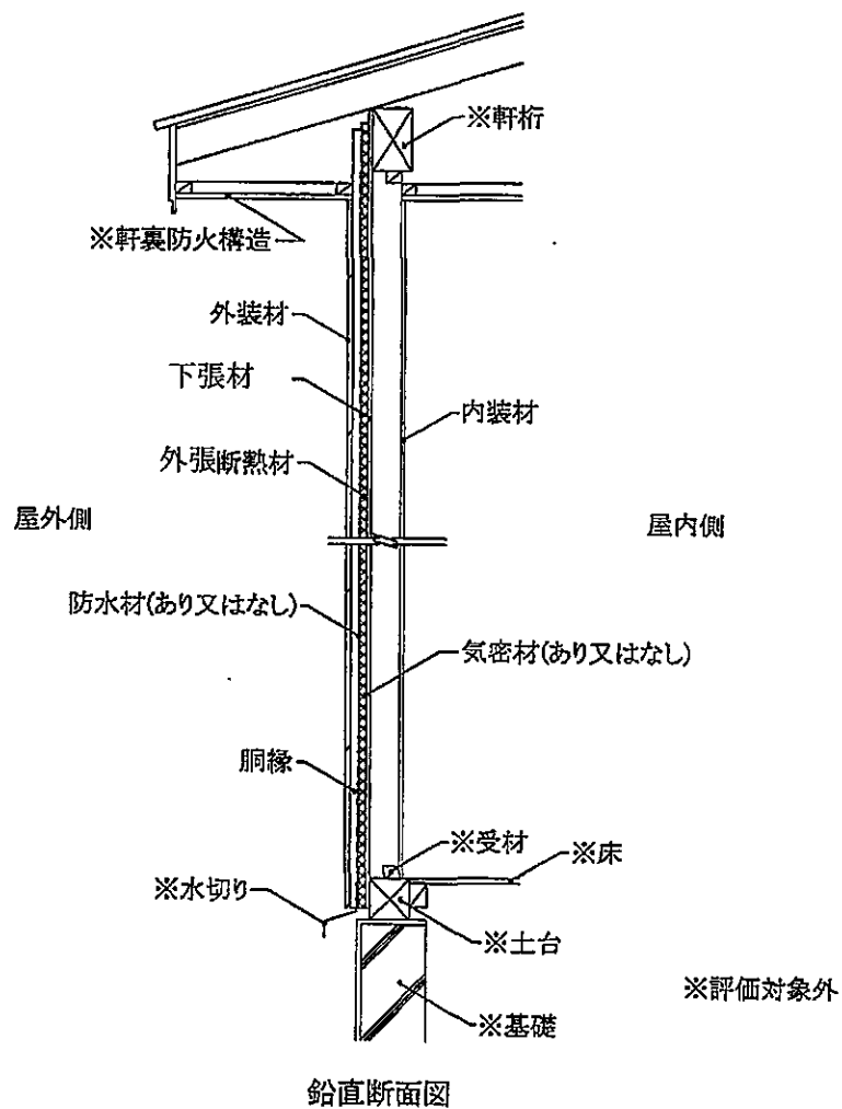
図22 施工図 (外装材横張・欠き込み真壁造／充てん断熱材なし・構造用面材なし・下張材あり)
