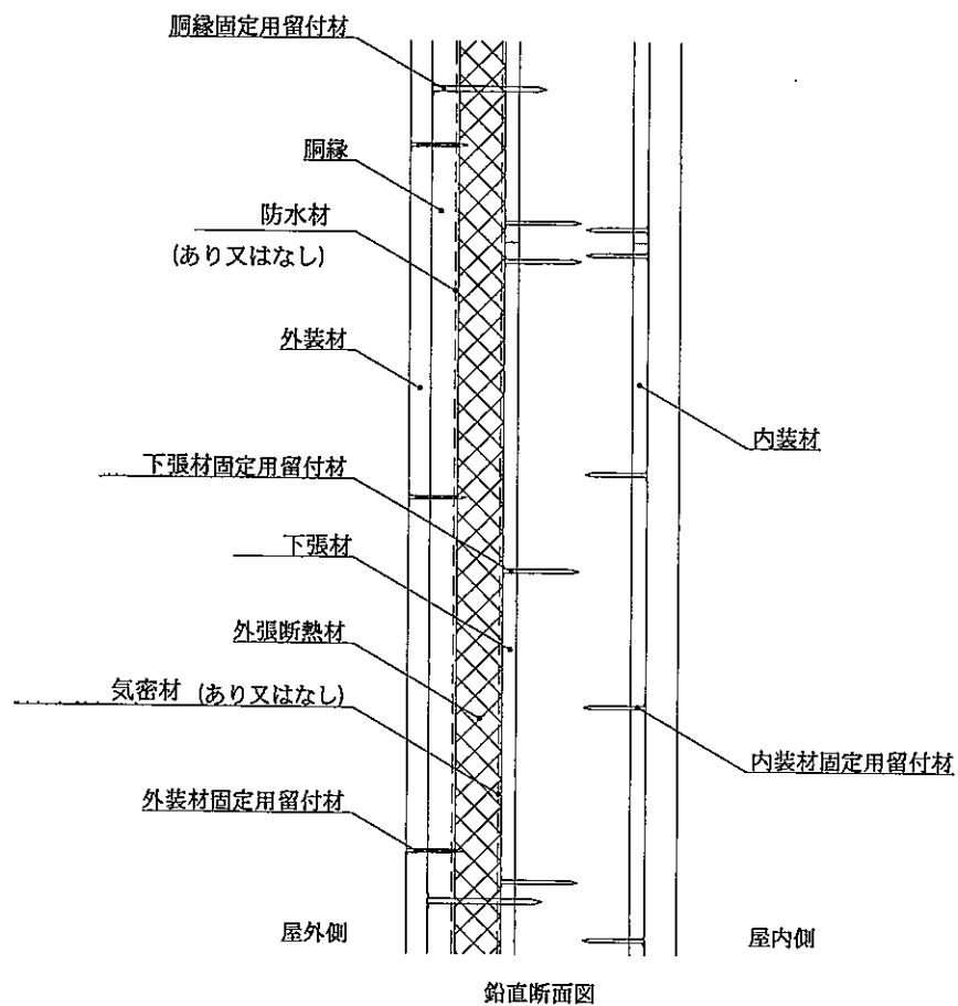
図12 構造説明図 (外装材縦張・受材真壁造／充てん断熱材なし・構造用面材なし・下張材あり)
