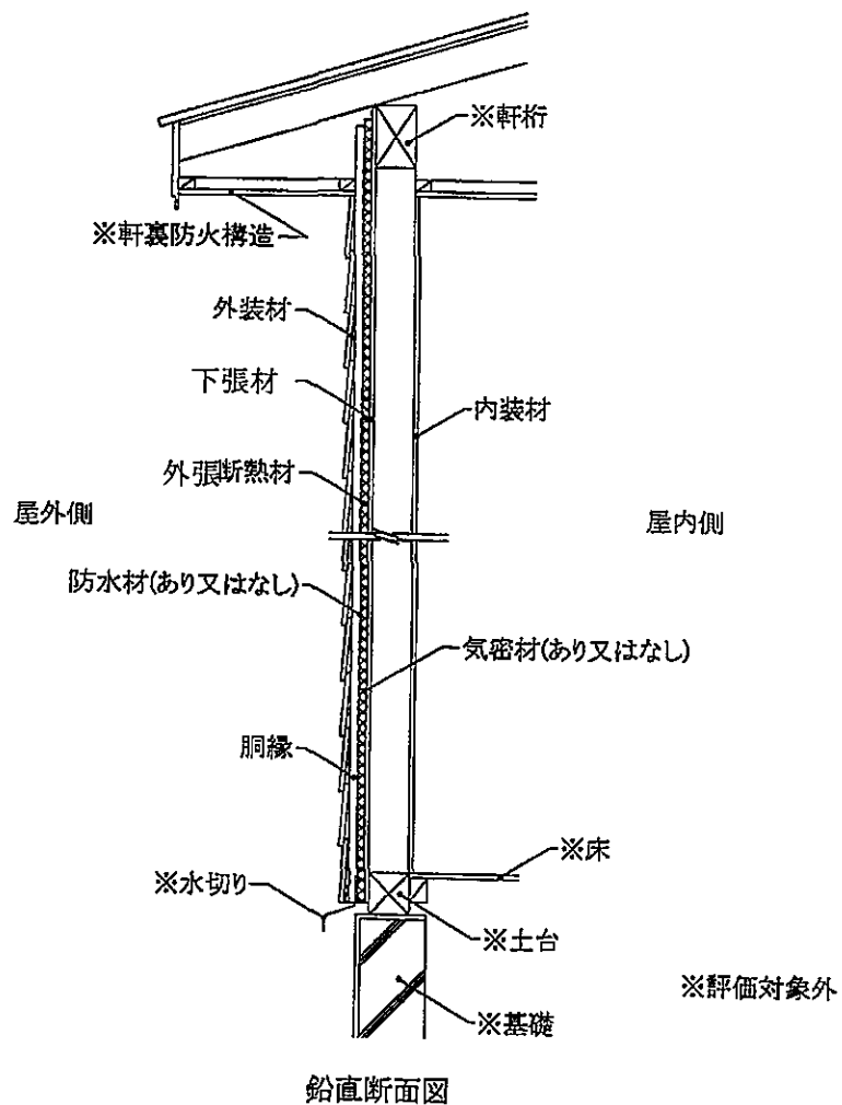
図29 施工図 (外装材横張・大壁造／充てん断熱材なし・構造用面材なし・下張材あり)
