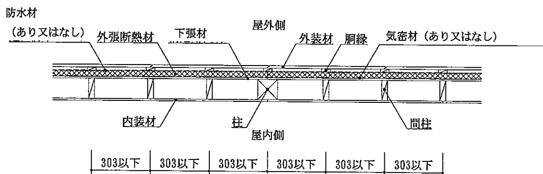
水平断面図 (大壁造・構造用面材あり・充てん断熱材なし仕様)
