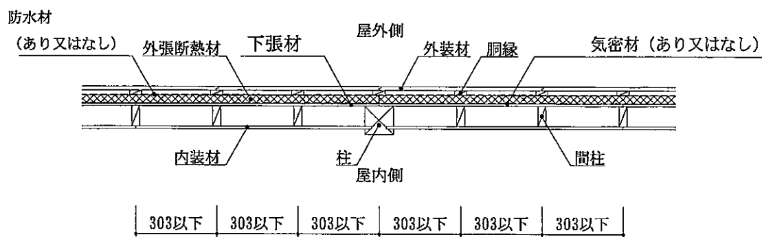
水平断面図 (欠き込み真壁造・構造用面材あり・充てん断熱材なし仕様)
