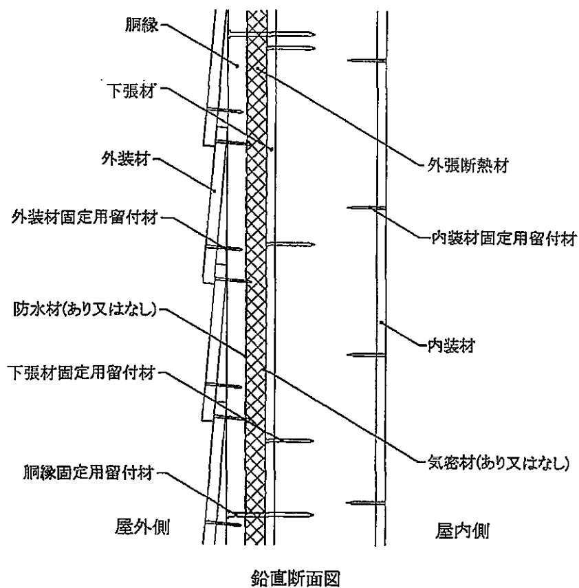
図16 構造説明図 (外装材横張・大壁造／充てん断熱材なし・構造用面材なし・下張材あり)
