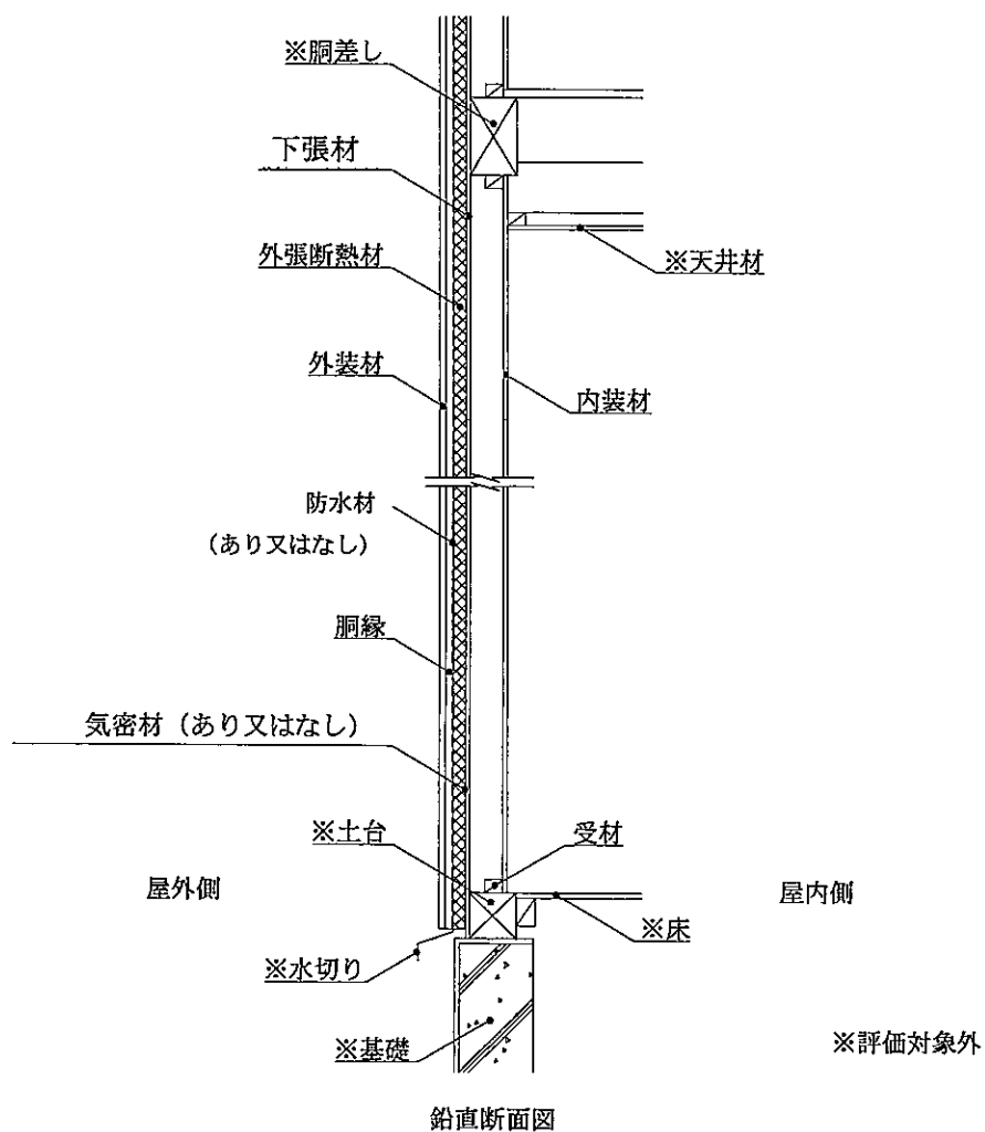
図24 施工図
