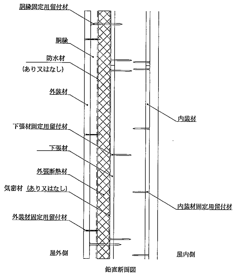
図6 構造説明図 (外装材横張・欠き込み真壁造／充てん断熱材なし・構造用面材なし・下張材あり)
