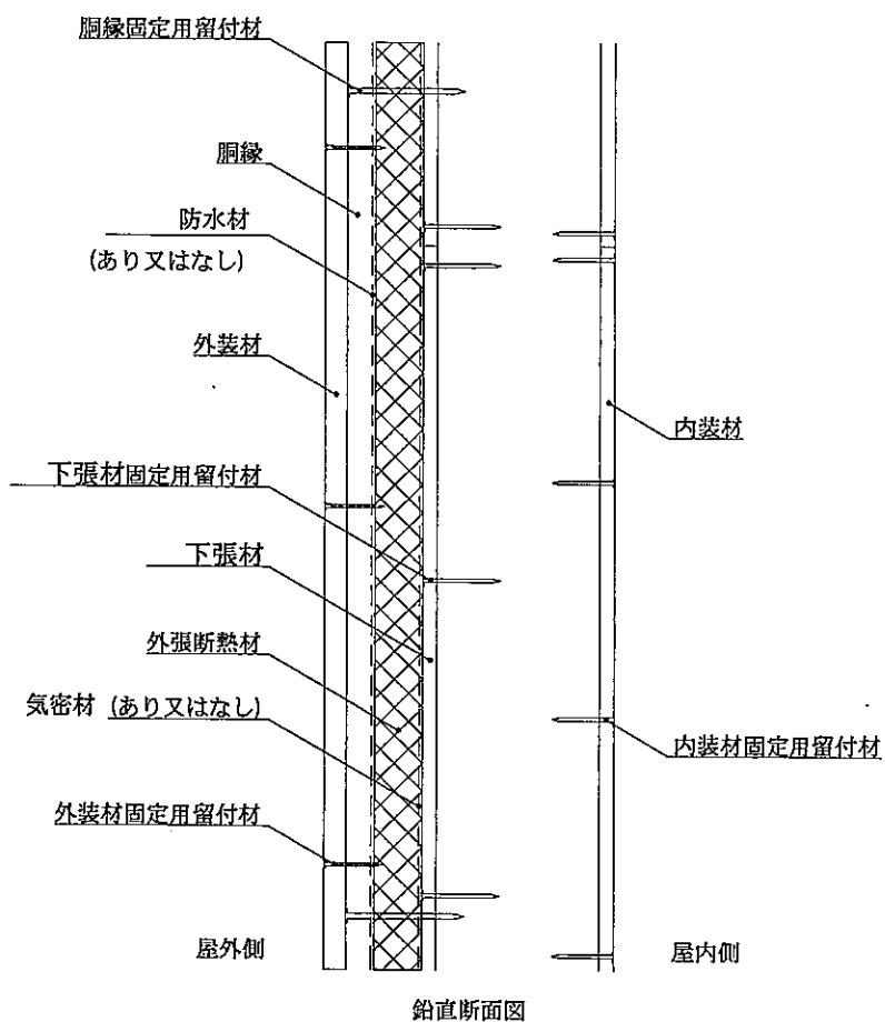
図18 構造説明図 (外装材縦張・大壁造／充てん断熱材なし・構造用面材なし・下張材あり)
