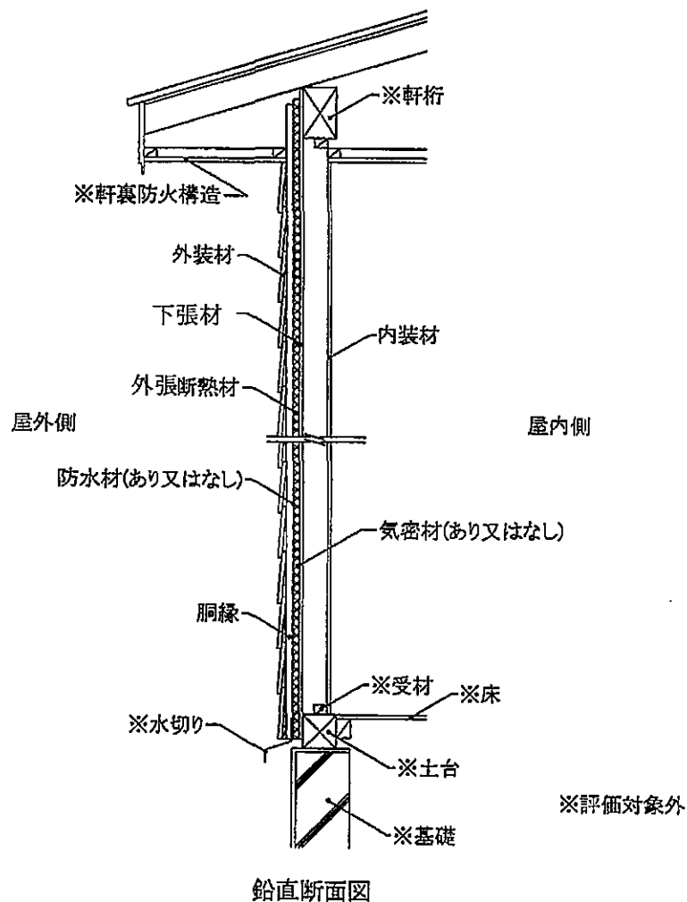
図26 施工図 (外装材横張・受材真壁造／充てん断熱材なし・構造用面材なし・下張材あり)
