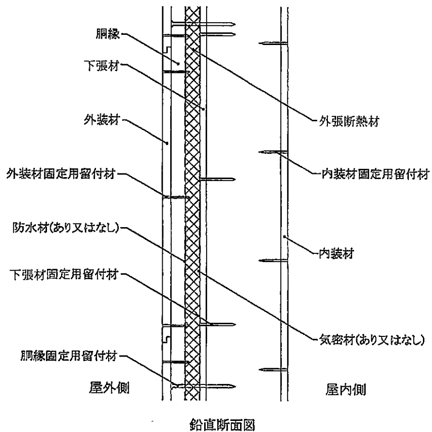
図14 構造説明図 (外装材横張・大壁造／充てん断熱材なし・構造用面材なし・下張材あり)
