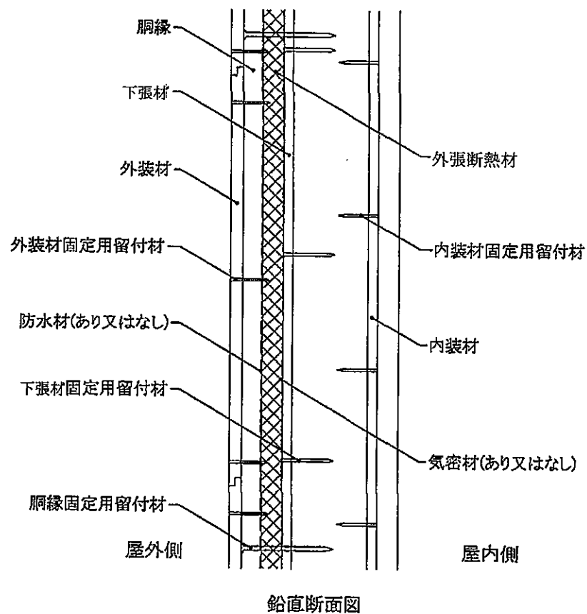
図8 構造説明図 (外装材横張・受材真壁造／充てん断熱材なし・構造用面材なし・下張材あり)
