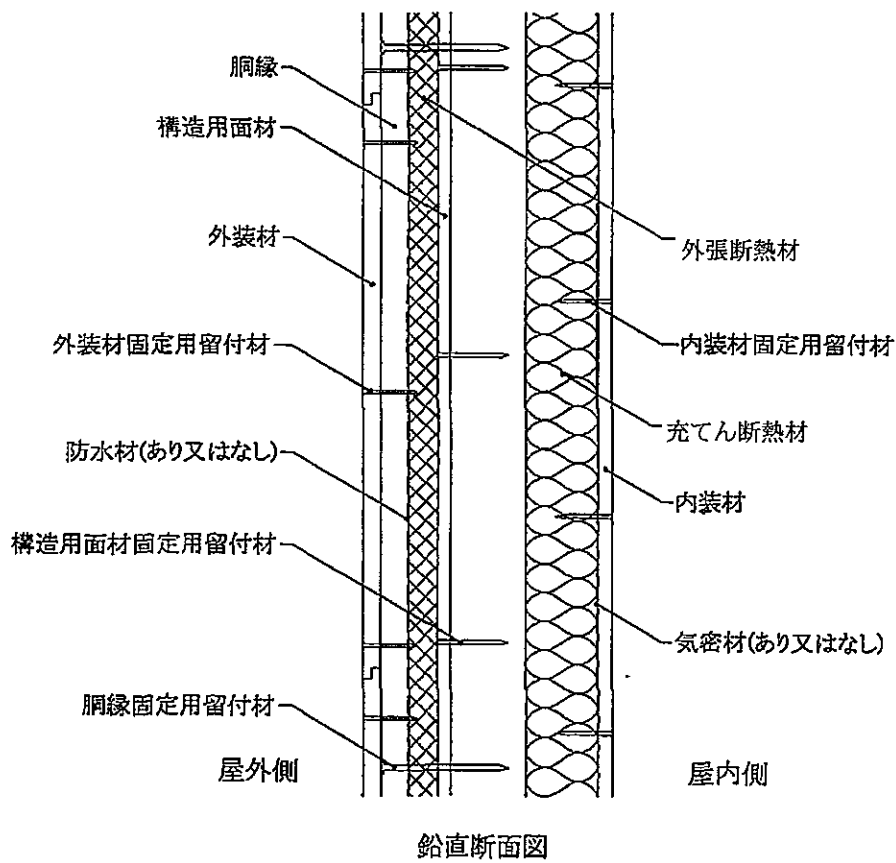
図14 構造説明図 (外装材横張・大壁造／充てん断熱材あり・構造用面材あり・下張材なし)
