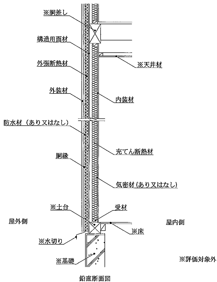
図27 施工図
