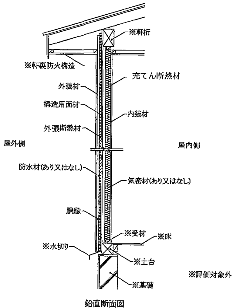
図25 施工図 (外装材横張・受材真壁造／充てん断熱材あり・構造用面材あり・下張材なし)
