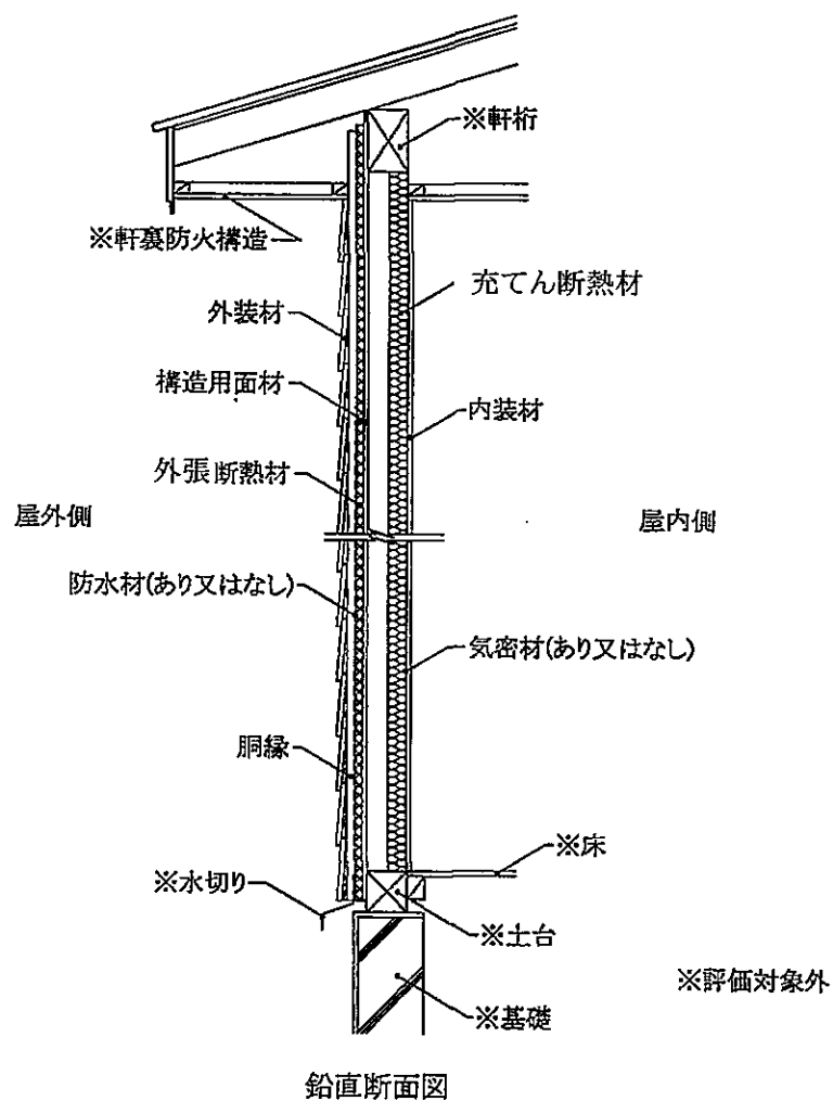
図29 施工図 (外装材横張・大壁造／充てん断熱材あり・構造用面材あり・下張材なし)
