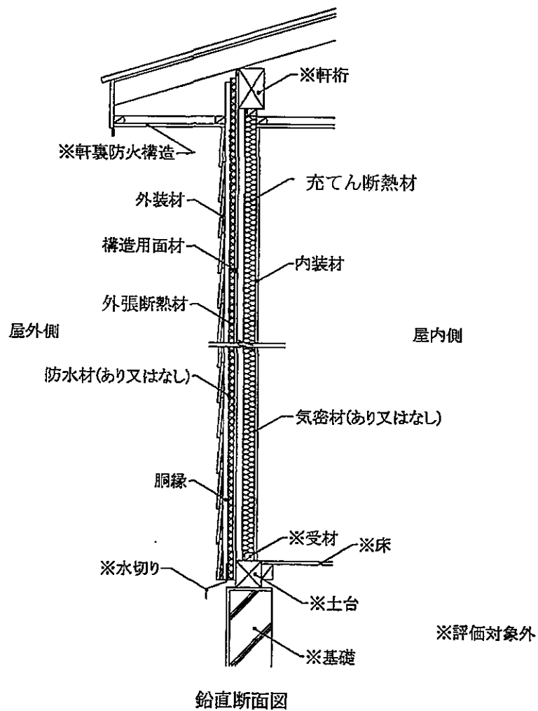
図23 施工図 (外装材横張・欠き込み真壁造／充てん断熱材あり・構造用面材あり・下張材なし)
