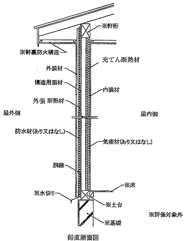
図28 施工図 (外装材横張・大壁造／充てん断熱材あり・構造用面材あり・下張材なし)
