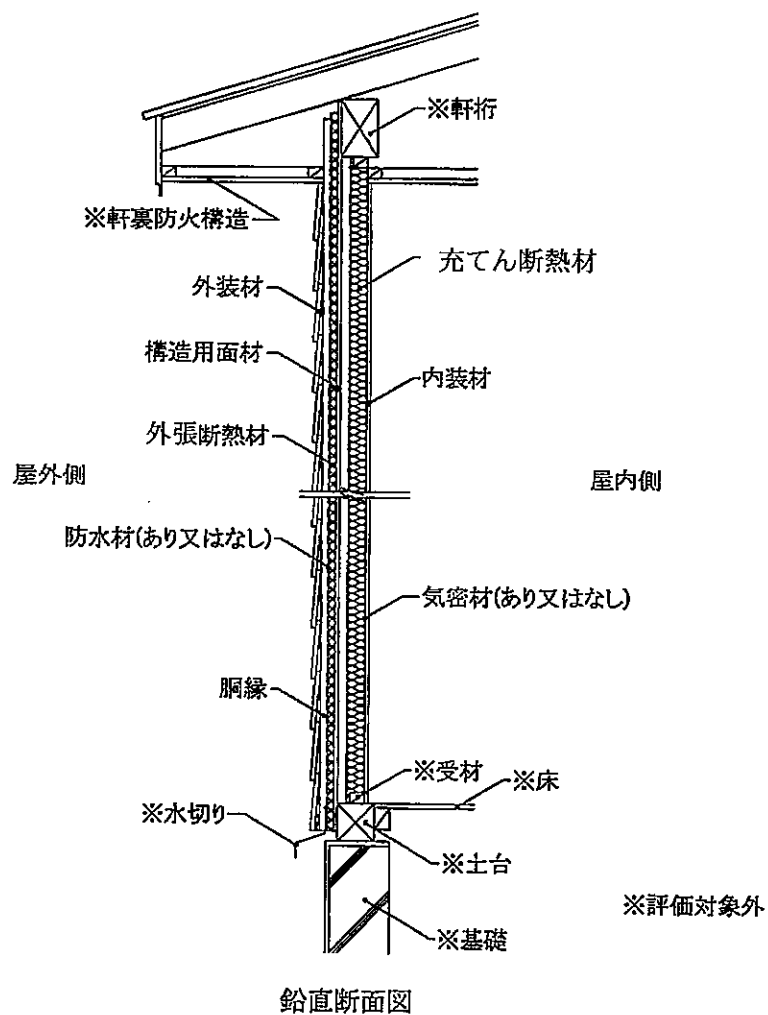
図26 施工図 (外装材横張・受材真壁造／充てん断熱材あり・構造用面材あり・下張材なし)
