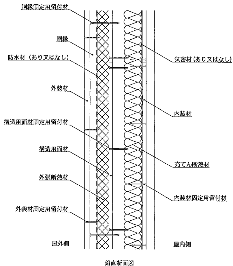
図12 構造説明図 (外装材横張・受材真壁造／充てん断熱材あり・構造用面材あり・下張材なし)
