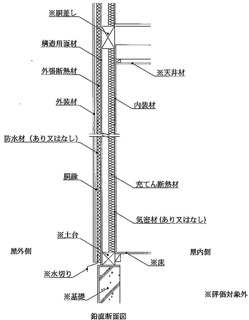
図30 施工図 (外装材横張・大壁造／充てん断熱材あり・構造用面材あり・下張材なし)
