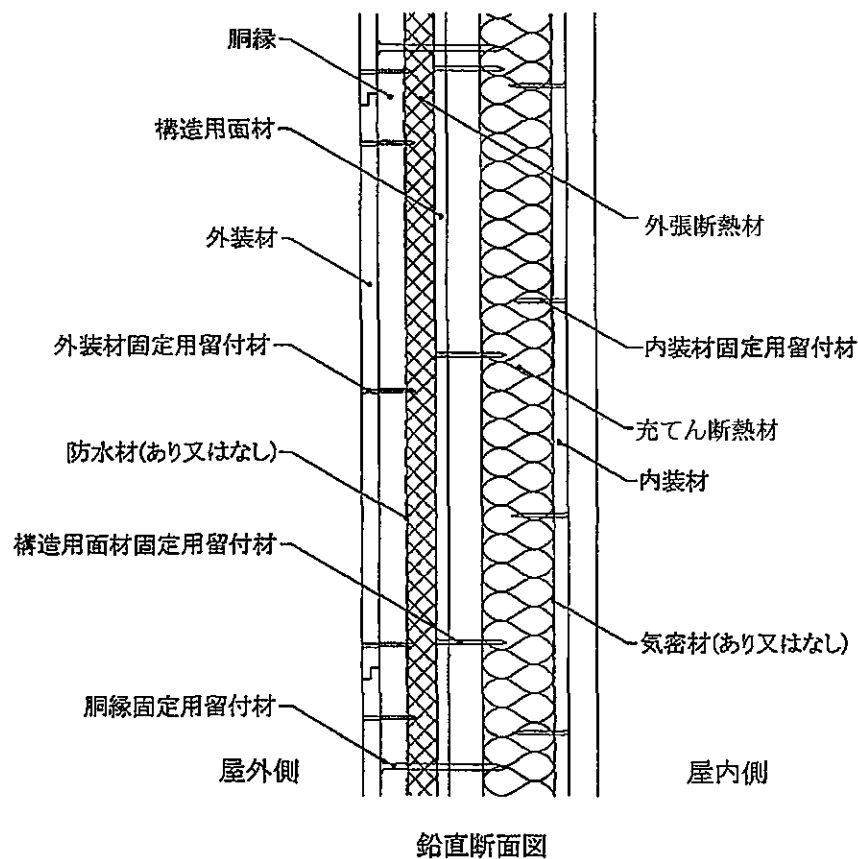
図8 構造説明図 (外装材横張・受材真壁造／充てん断熱材あり・構造用面材あり・下張材なし)
