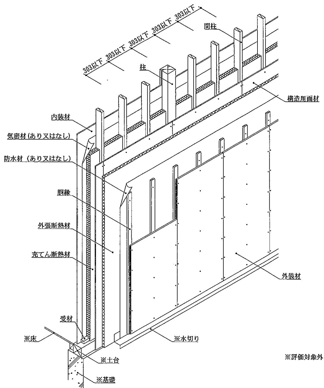
透視図
