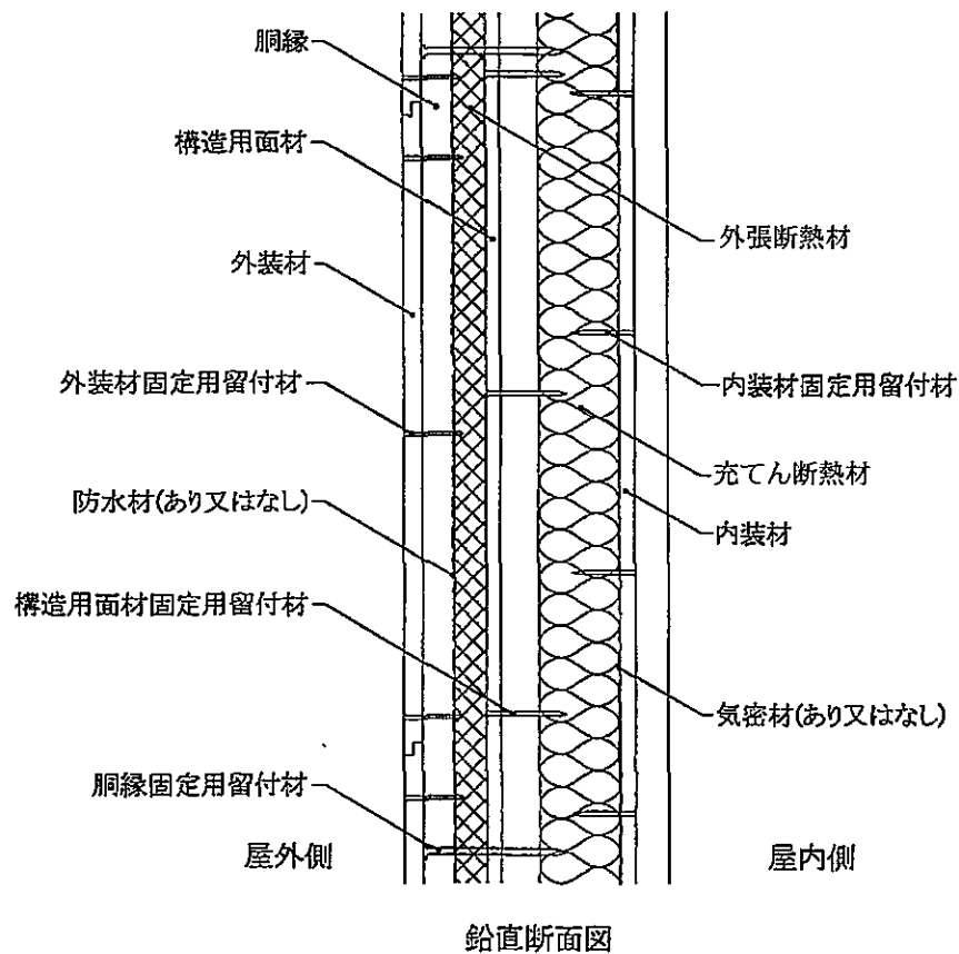
図2 構造説明図 (外装材横張・欠き込み真壁造／充てん断熱材あり・構造用面材あり・下張材なし)
