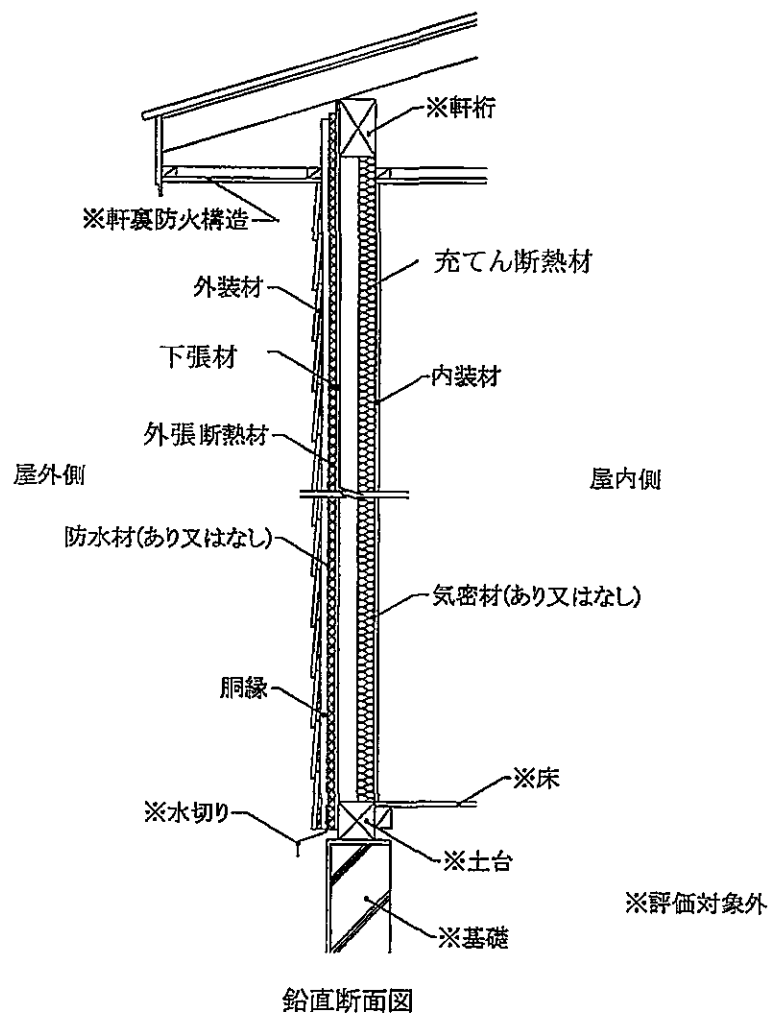
図29 施工図 (外装材横張・大壁造／充てん断熱材あり・構造用面材なし・下張材あり)
