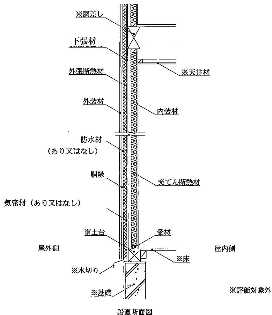
図24 施工図
