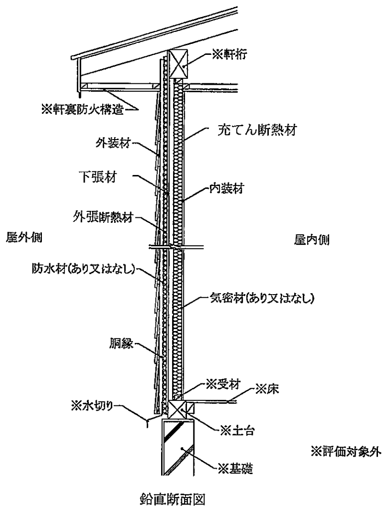
図26 施工図 (外装材横張・受材真壁造／充てん断熱材あり・構造用面材なし・下張材あり)
