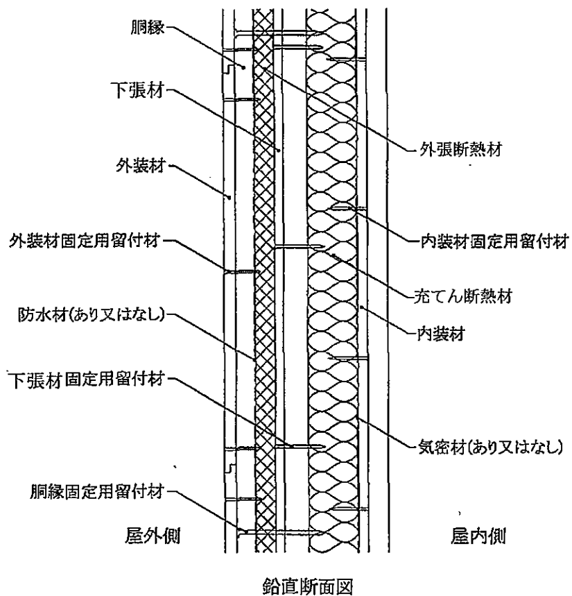
図2 構造説明図 (外装材横張・欠き込み真壁造／充てん断熱材あり・構造用面材なし・下張材あり)
