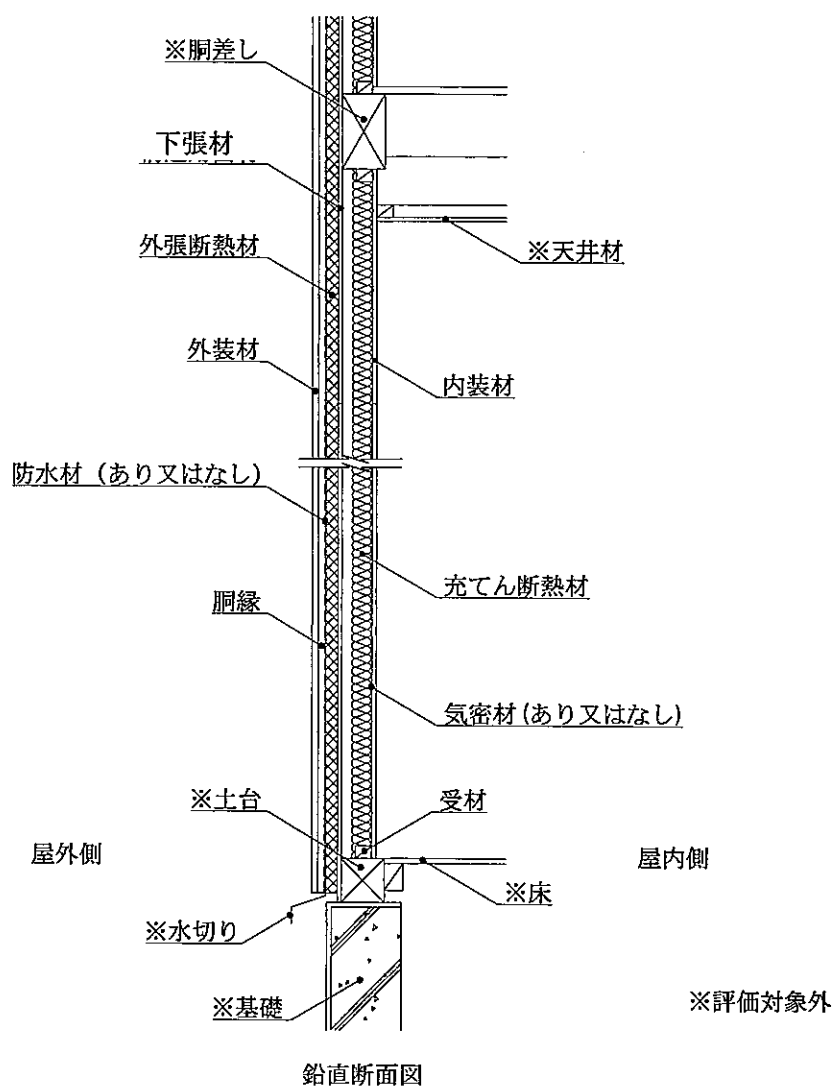
図27 施工図 (外装材縦張・受材真壁造／充てん断熱材あり・構造用面材なし・下張材あり)
