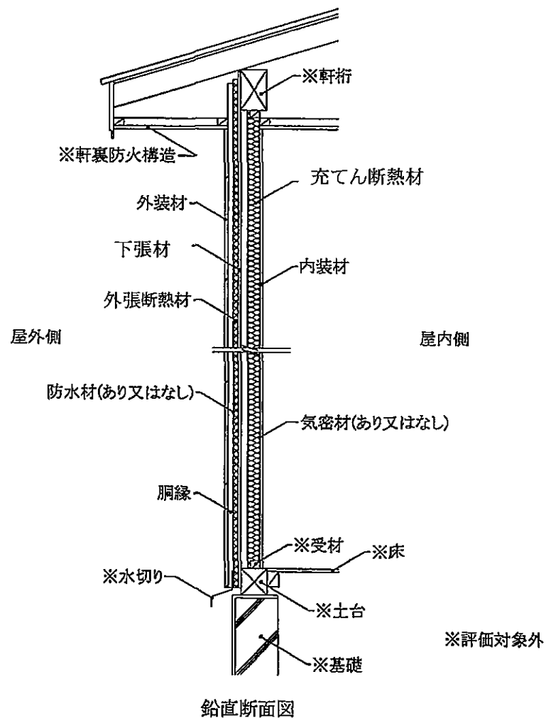
図22 施工図
