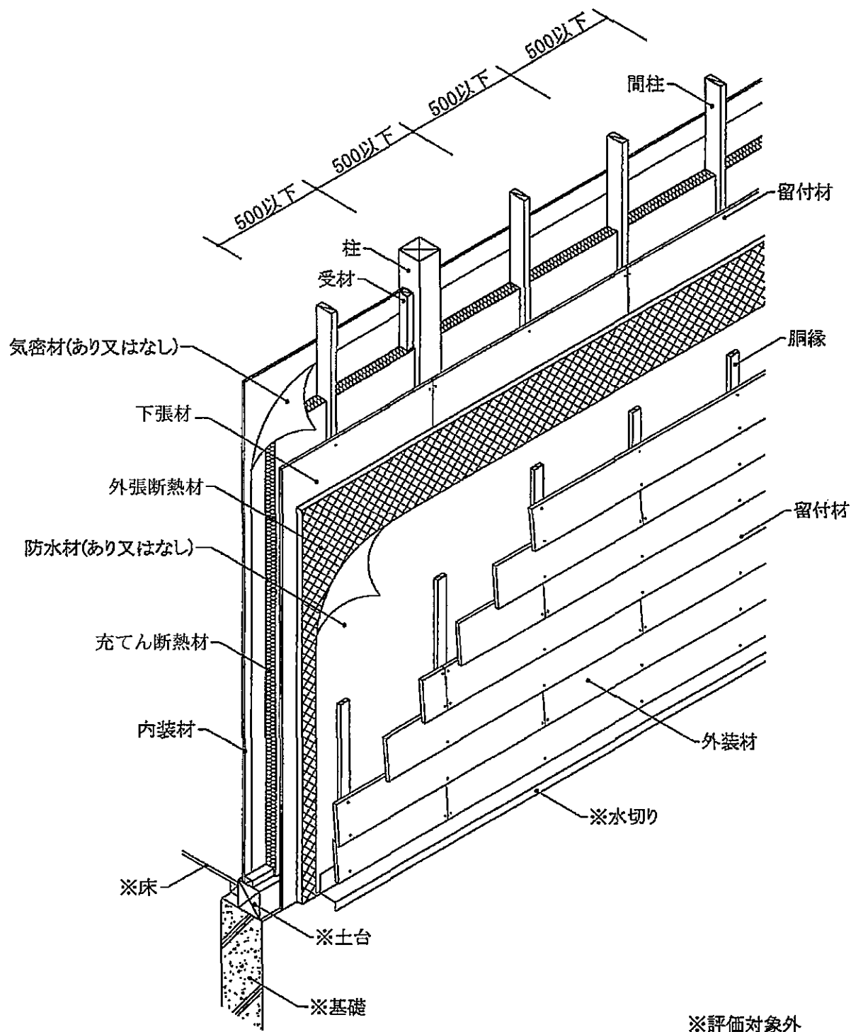
透視図
