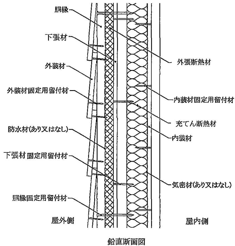
図4 構造説明図 (外装材横張・欠き込み真壁造／充てん断熱材あり・構造用面材なし・下張材あり)
