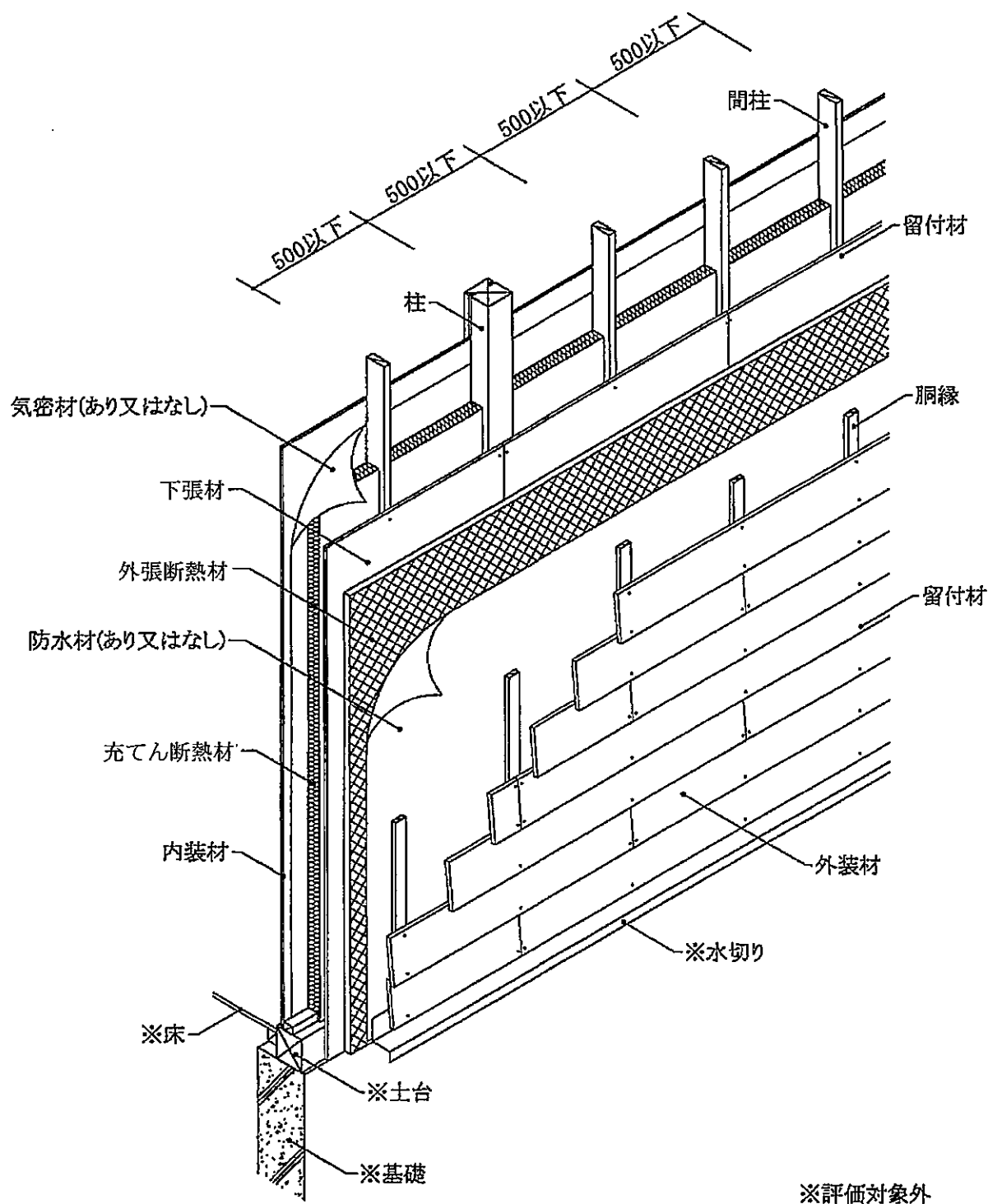
透視図
