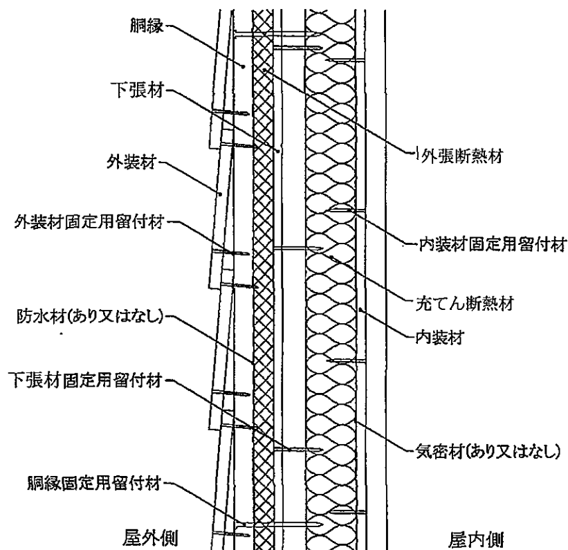
鉛直断面図
