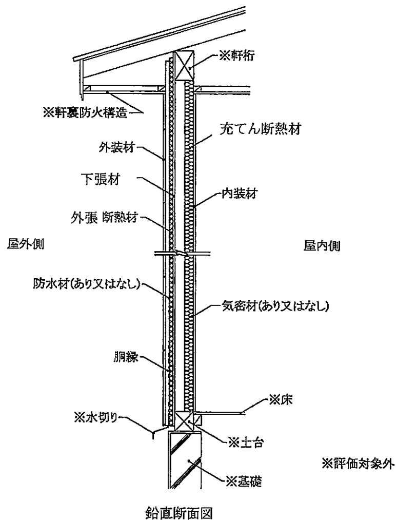
図28 施工図 (外装材横張・大壁造／充てん断熱材あり・構造用面材なし・下張材あり)
