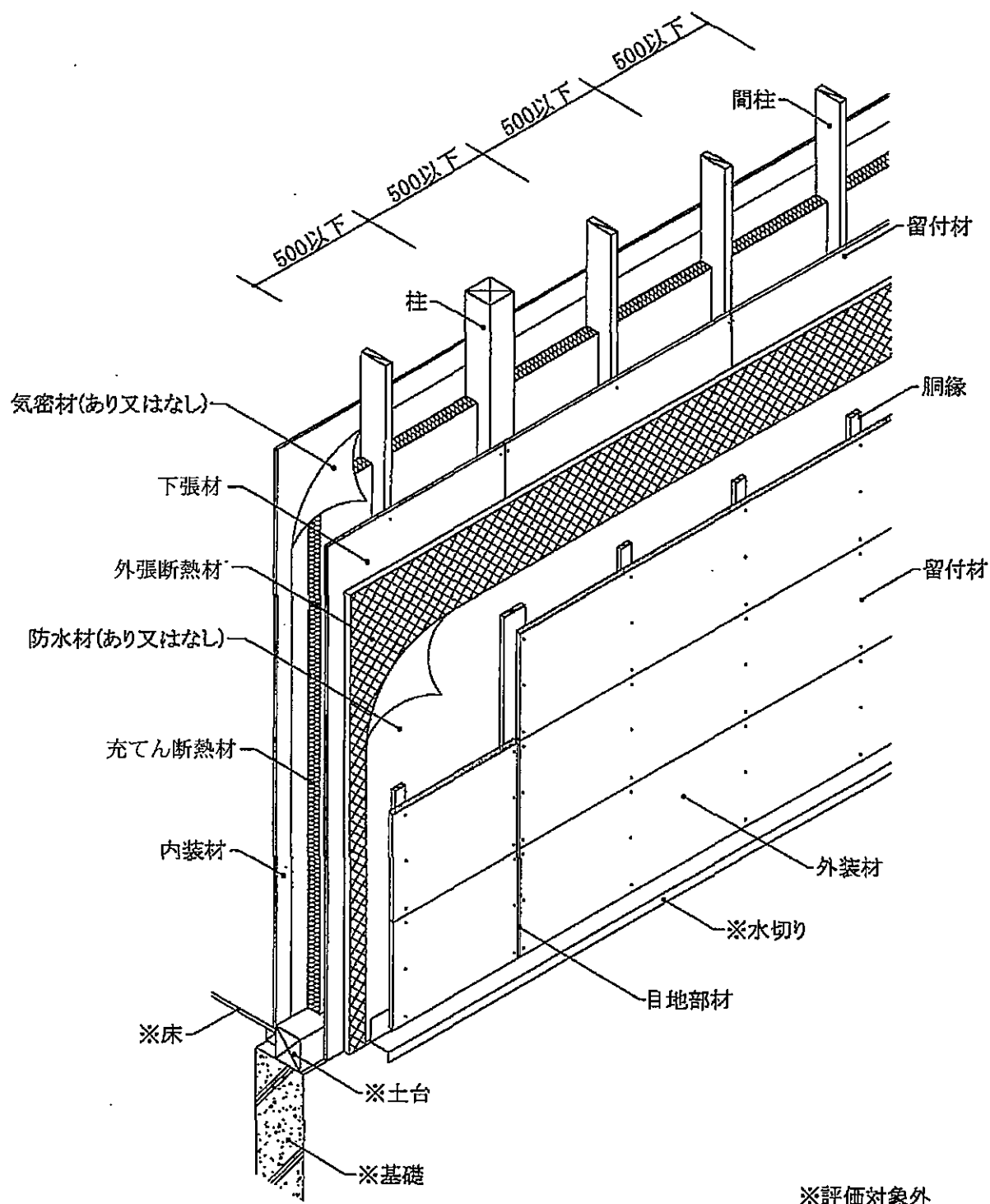
透視図
