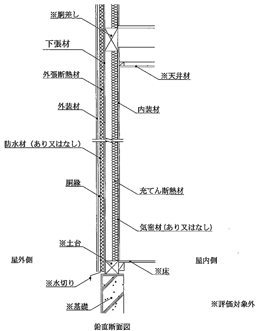
図30 施工図 (外装材横張・大壁造／充てん断熱材あり・構造用面材なし・下張材あり)
