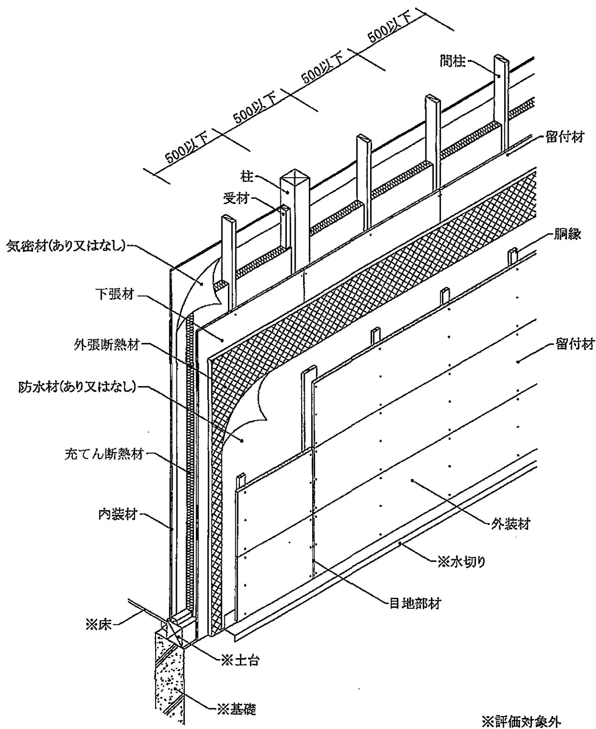
透視図
