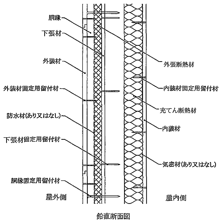
図14 構造説明図 (外装材横張・大壁造／充てん断熱材あり・構造用面材なし・下張材あり)
