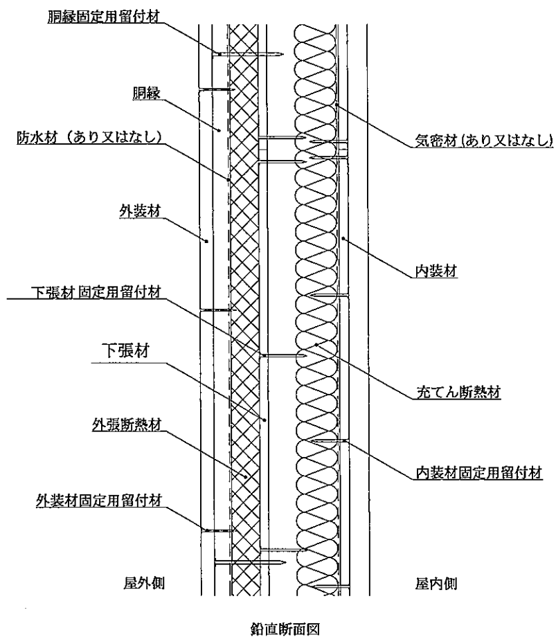
図12 構造説明図 (外装材横張・受材真壁造／充てん断熱材あり・構造用面材なし・下張材あり)
