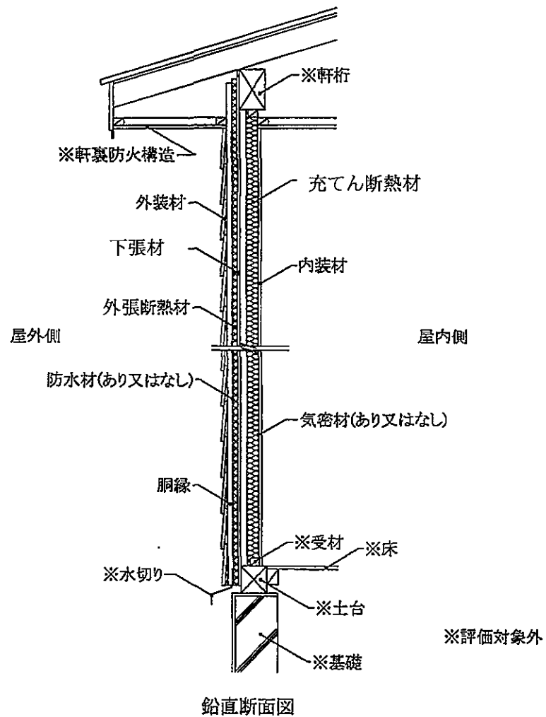
図23 施工図 (外装材横張・欠き込み真壁造／充てん断熱材あり・構造用面材なし・下張材あり)
