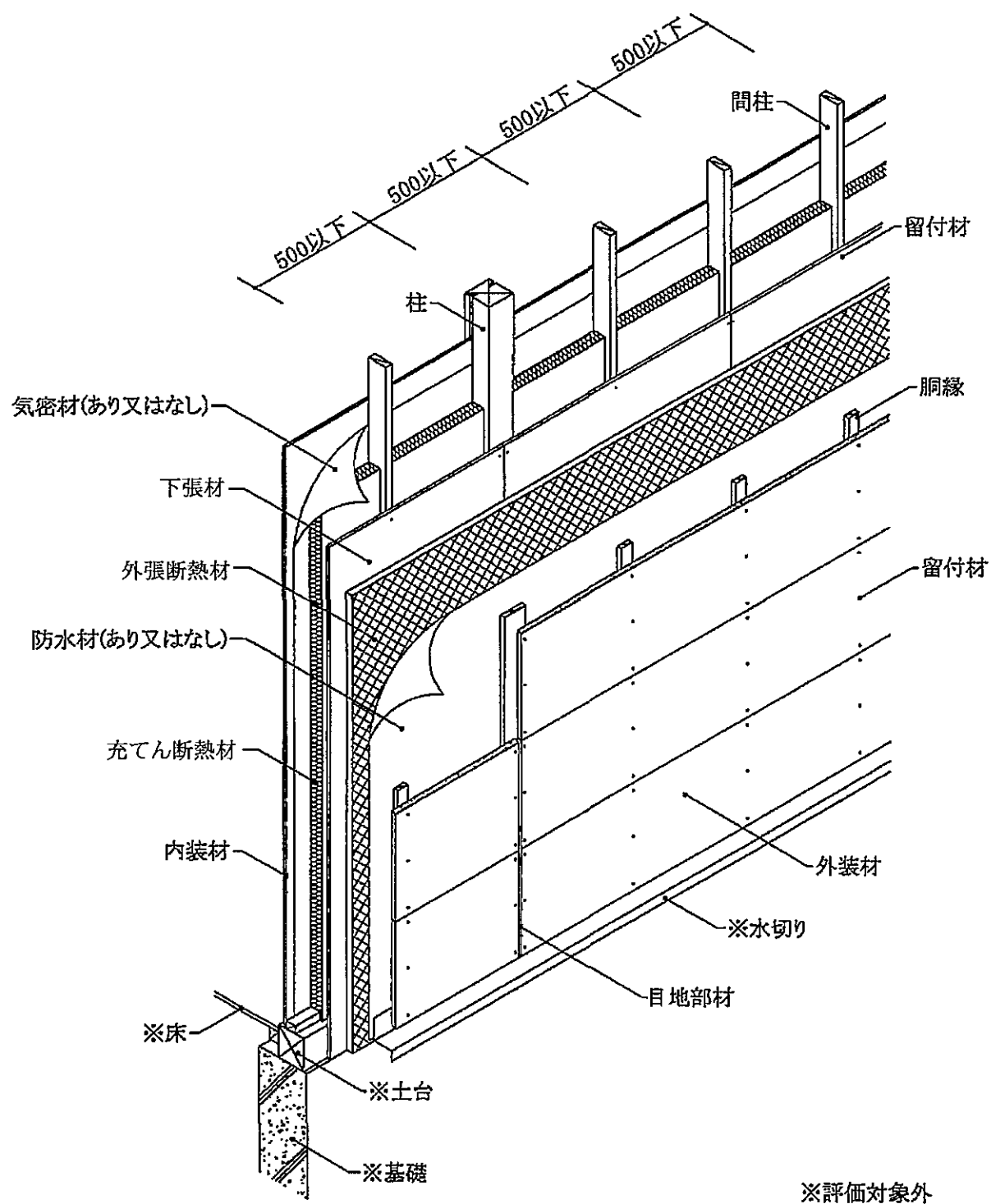
透視図
