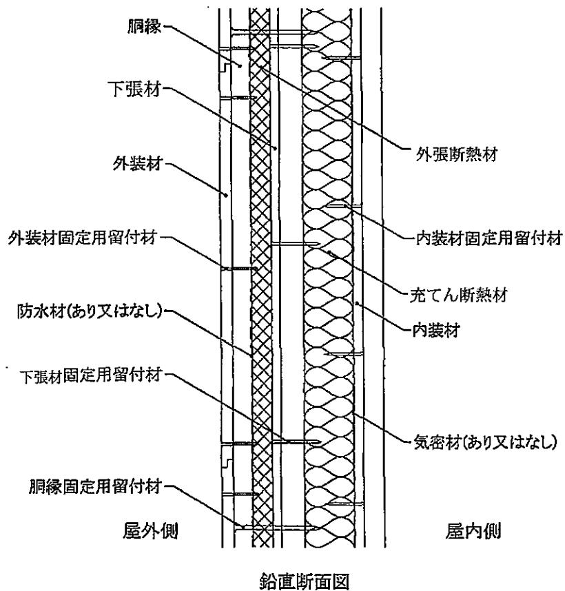
図8 構造説明図 (外装材横張・受材真壁造／充てん断熱材あり・構造用面材なし・下張材あり)
