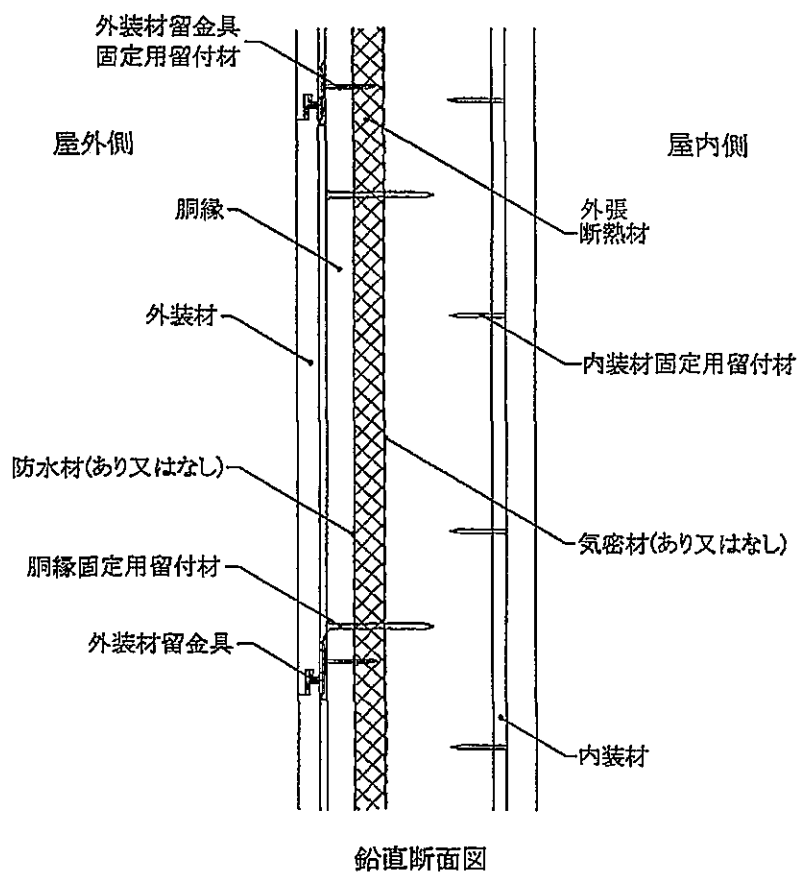
図2 構造説明図 (欠き込み真壁造／充てん断熱材なし・構造用面材なし・下張材なし)
