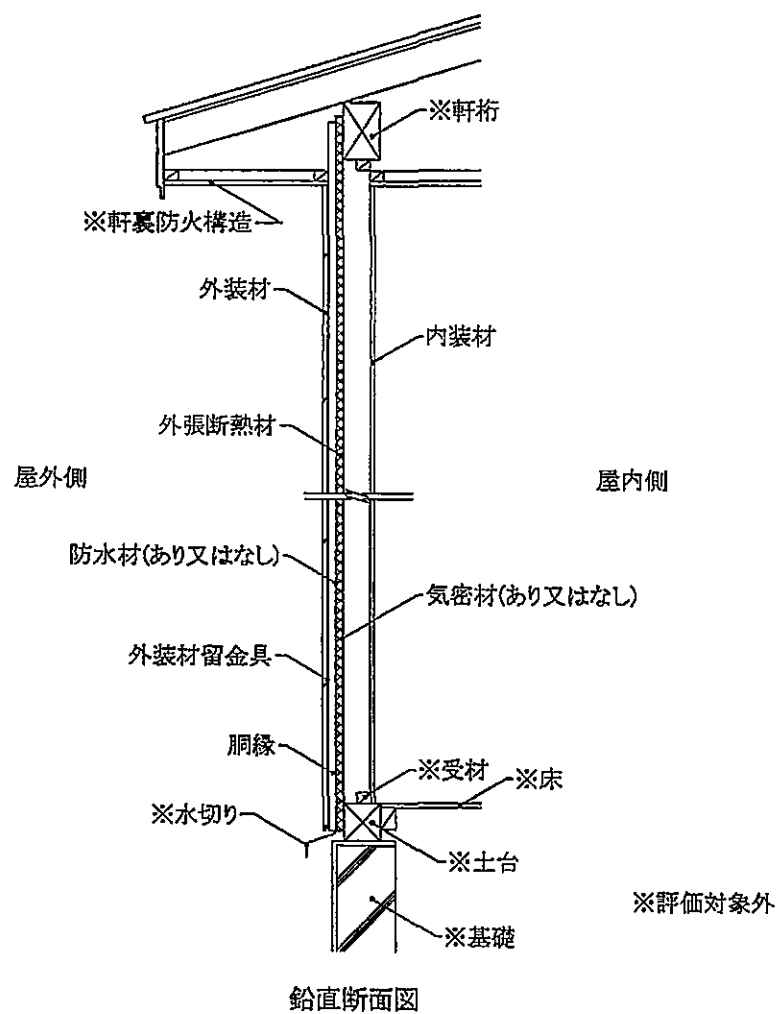
図12 構造説明図 (受材真壁造／充てん断熱材なし・構造用面材なし・下張材なし)
