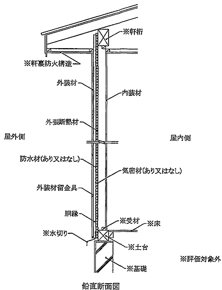
図11 構造説明図 (欠き込み真壁造／充てん断熱材なし・構造用面材なし・下張材なし)
