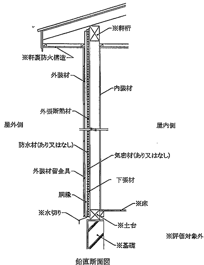
図13 構造説明図 (大壁造／充てん断熱材なし・構造用面材なし・下張材あり)
