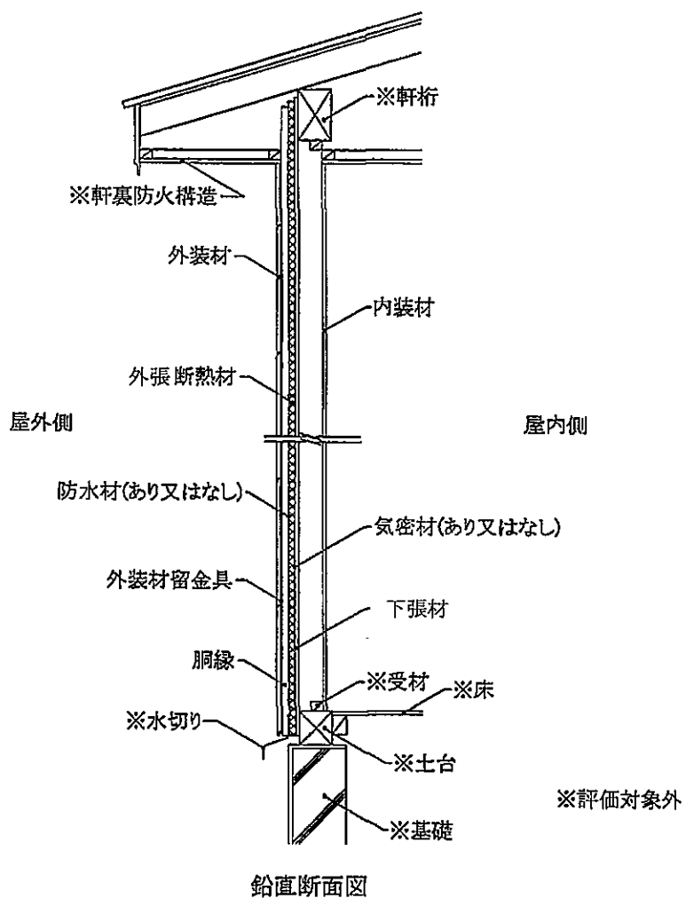
図12 構造説明図 (受材真壁造／充てん断熱材なし・構造用面材なし・下張材あり)
