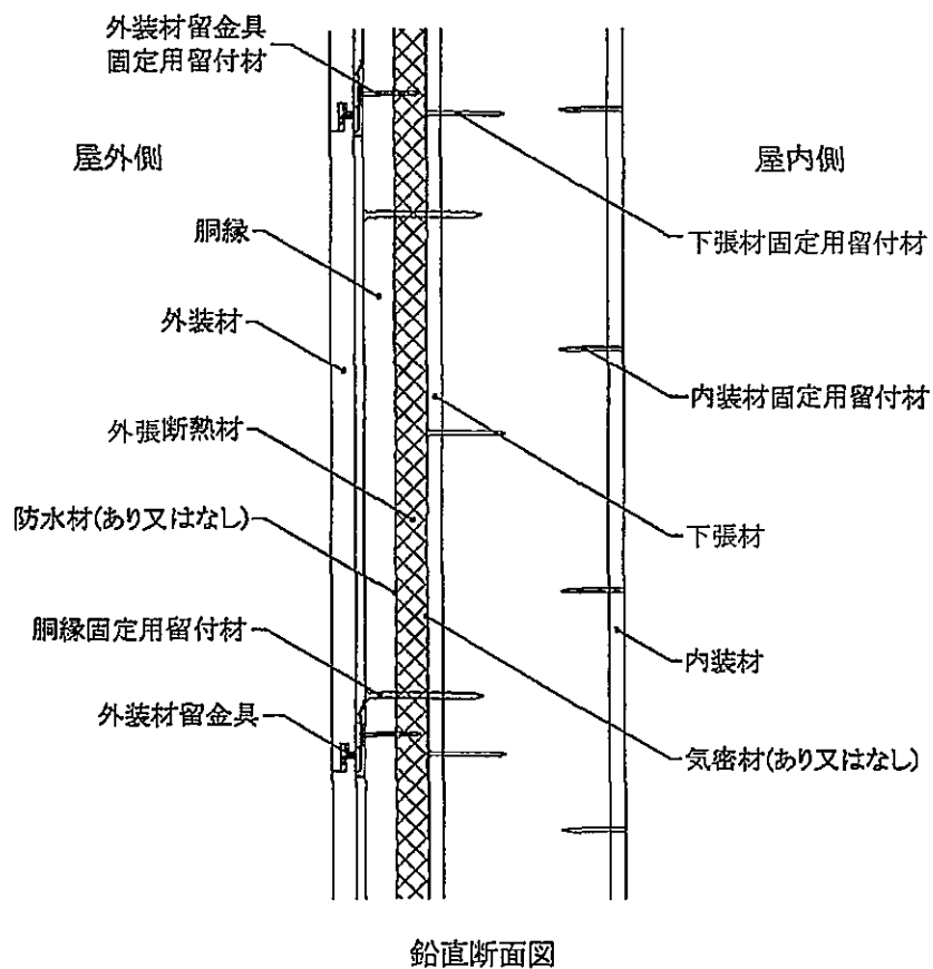
図6 構造説明図 (大壁造／充てん断熱材なし・構造用面材なし・下張材あり)
