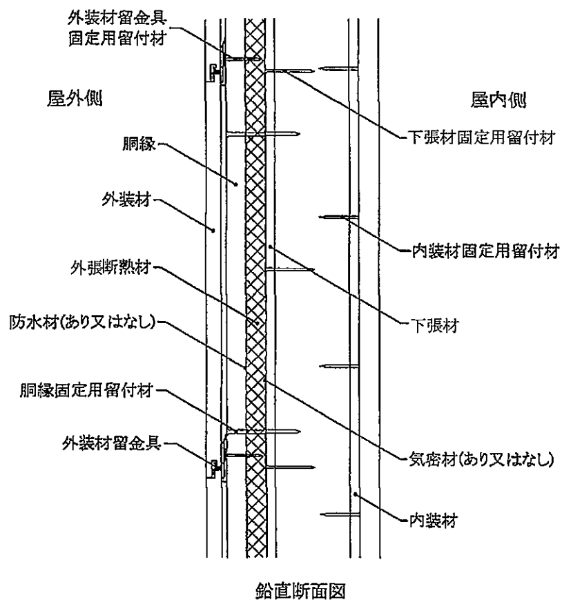
図2 構造説明図 (欠き込み真壁造／充てん断熱材なし・構造用面材なし・下張材あり)
