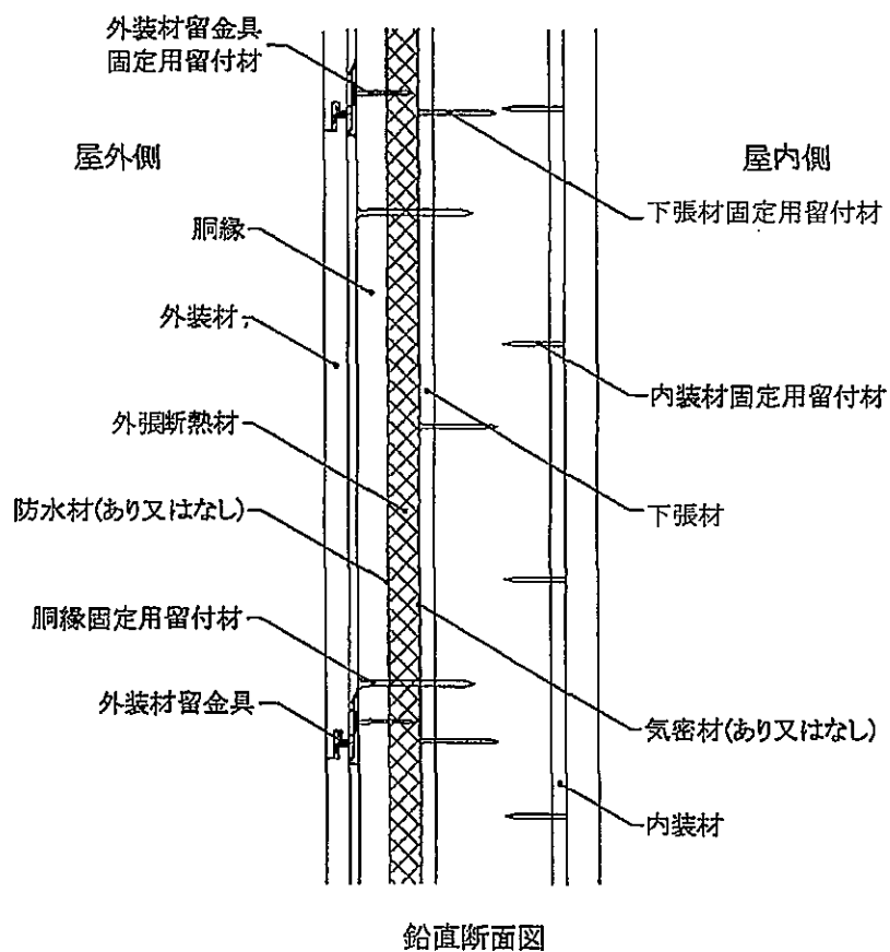
図4 構造説明図 (受材真壁造／充てん断熱材なし・構造用面材なし・下張材あり)
