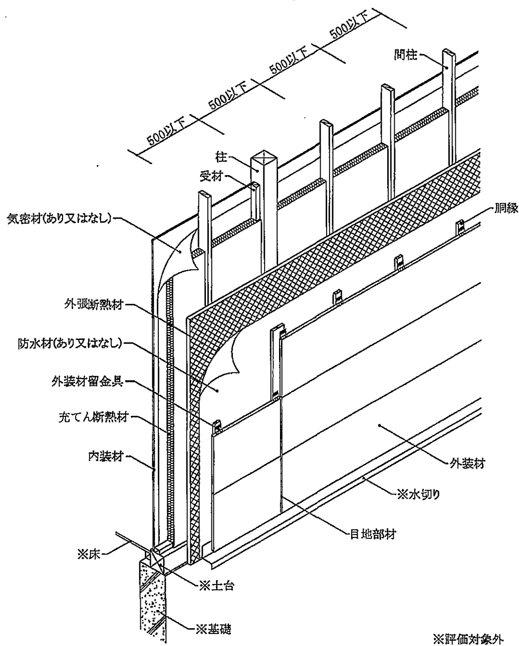
透視図
