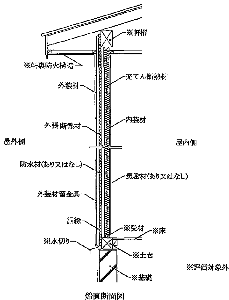
図11 構造説明図 (欠き込み真壁造/充てん断熱材あり・構造用面材なし・下張材なし)
