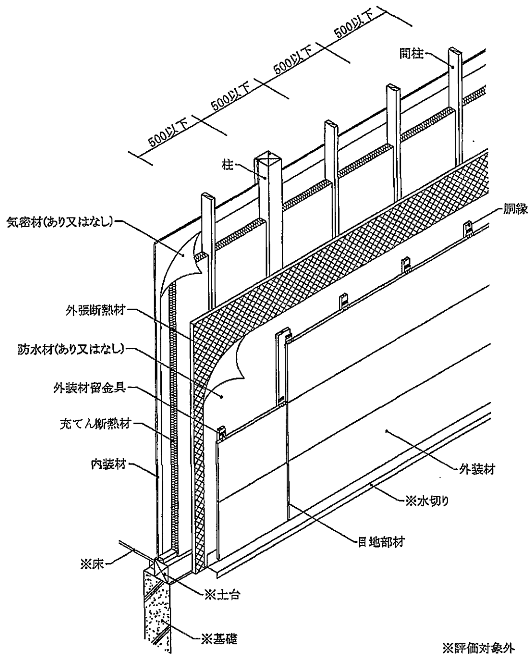
透視図
