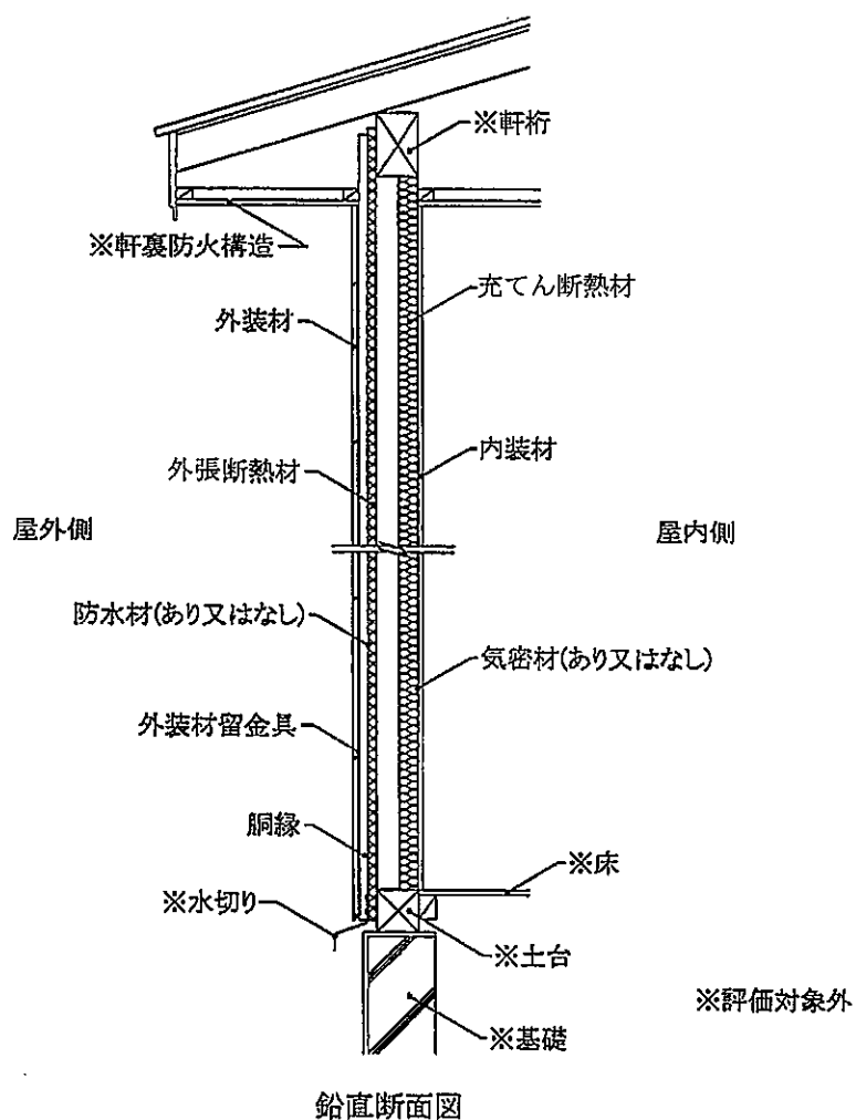
図13 構造説明図 (大壁造／充てん断熱材あり・構造用面材なし・下張材なし)
