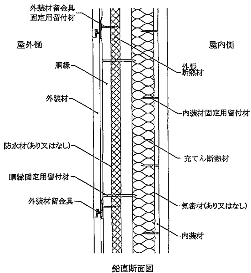
図4 構造説明図 (受材真壁造／充てん断熱材あり・構造用面材なし・下張材なし)
