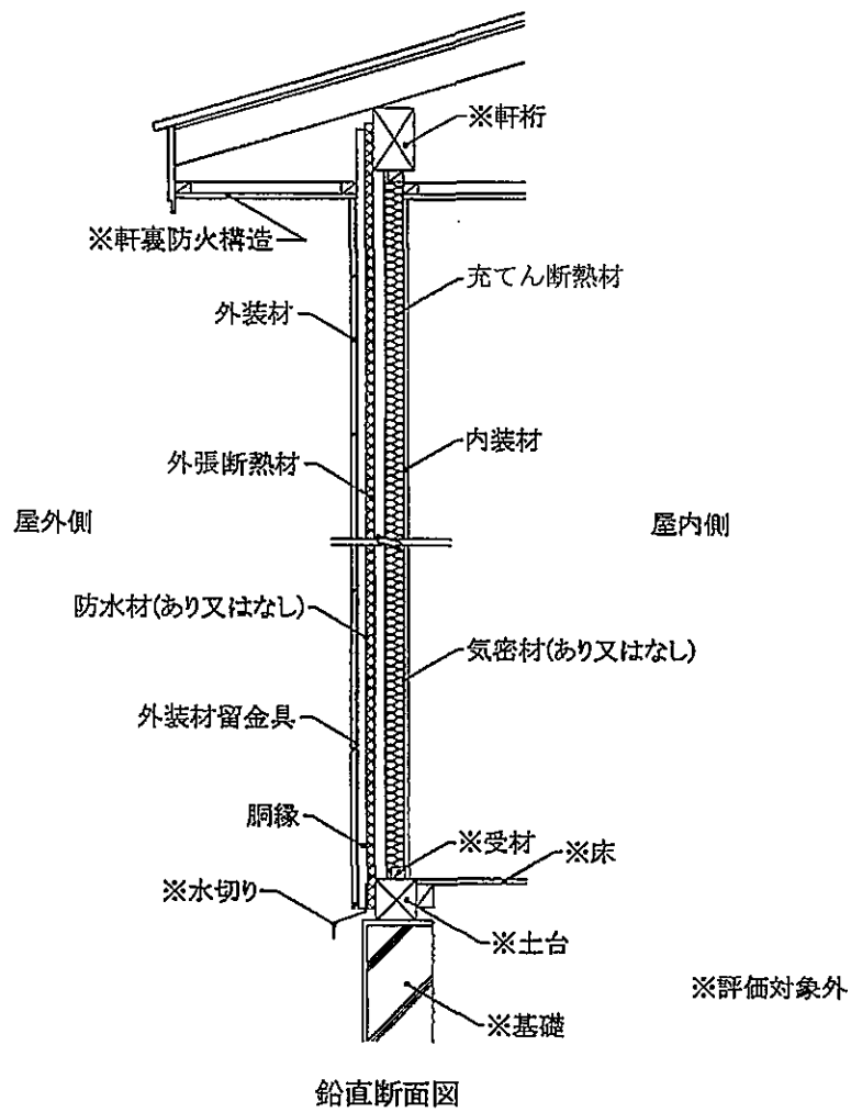
図12 構造説明図 (受材真壁造／充てん断熱材あり・構造用面材なし・下張材なし)
