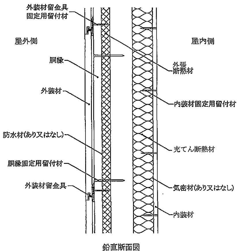
図6 構造説明図 (大壁造／充てん断熱材あり・構造用面材なし・下張材なし)
