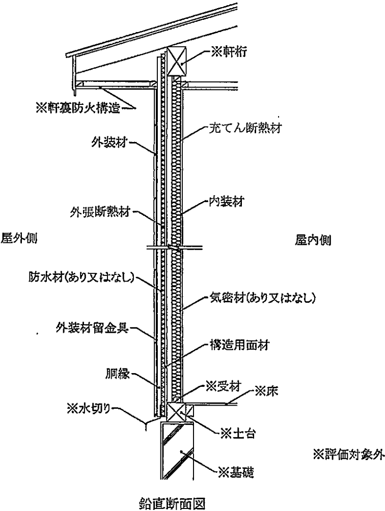
図12 構造説明図 (受材真壁造／充てん断熱材あり・構造用面材あり・下張材なし)
