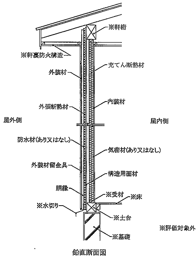
図11 構造説明図 (欠き込み真壁造／充てん断熱材あり・構造用面材あり・下張材なし)
