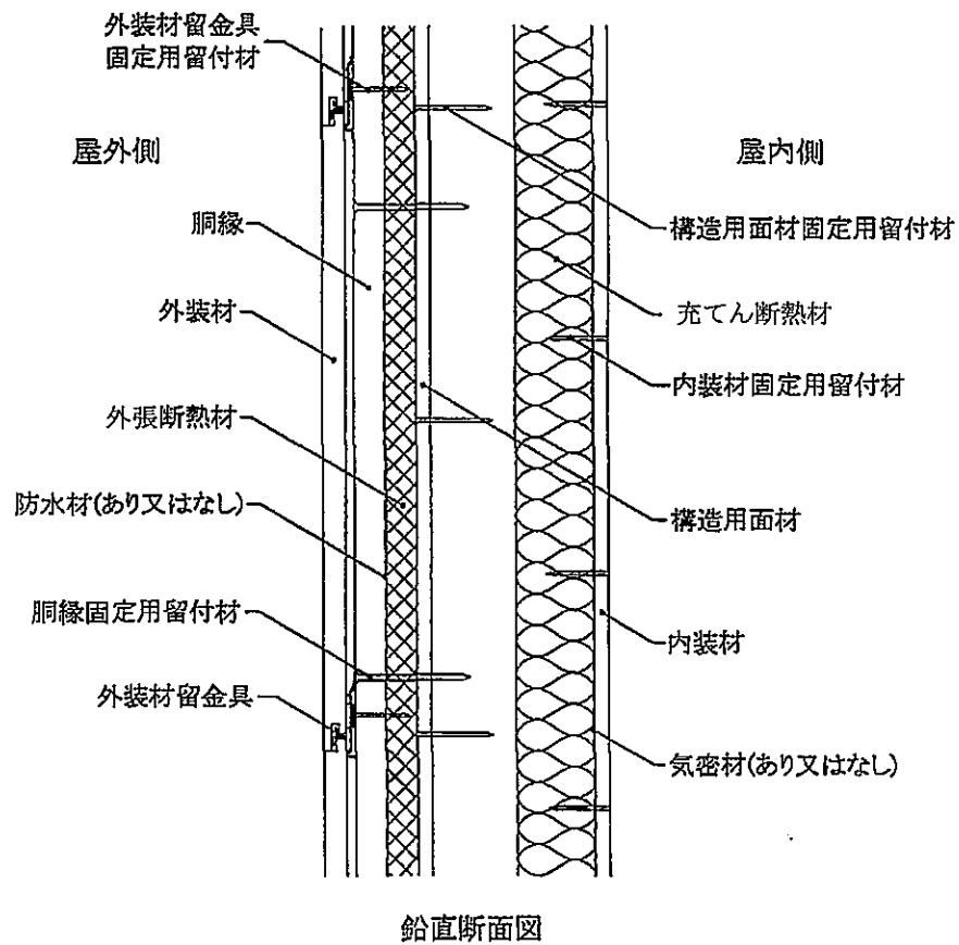
図6 構造説明図 (大壁造/充てん断熱材あり・構造用面材あり・下張材なし)
