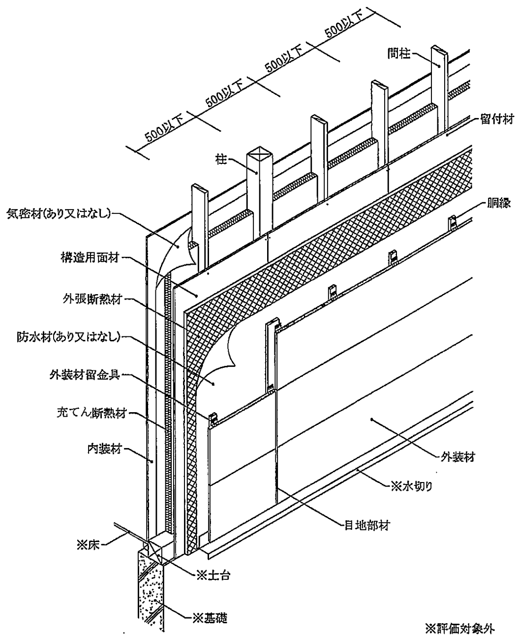
透視図
