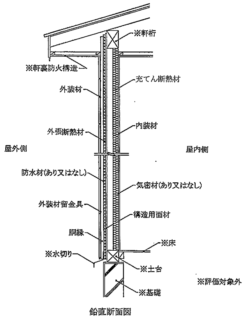
図13 構造説明図 (大壁造／充てん断熱材あり・構造用面材あり・下張材なし)
