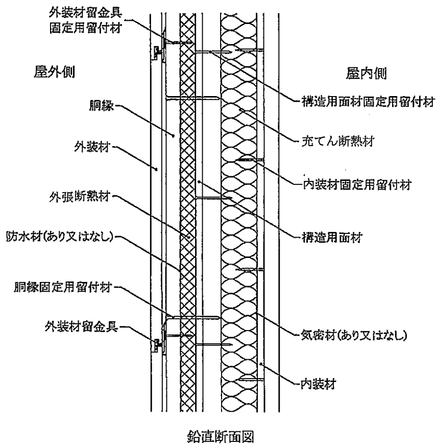
図4 構造説明図 (受材真壁造／充てん断熱材あり・構造用面材あり・下張材なし)
