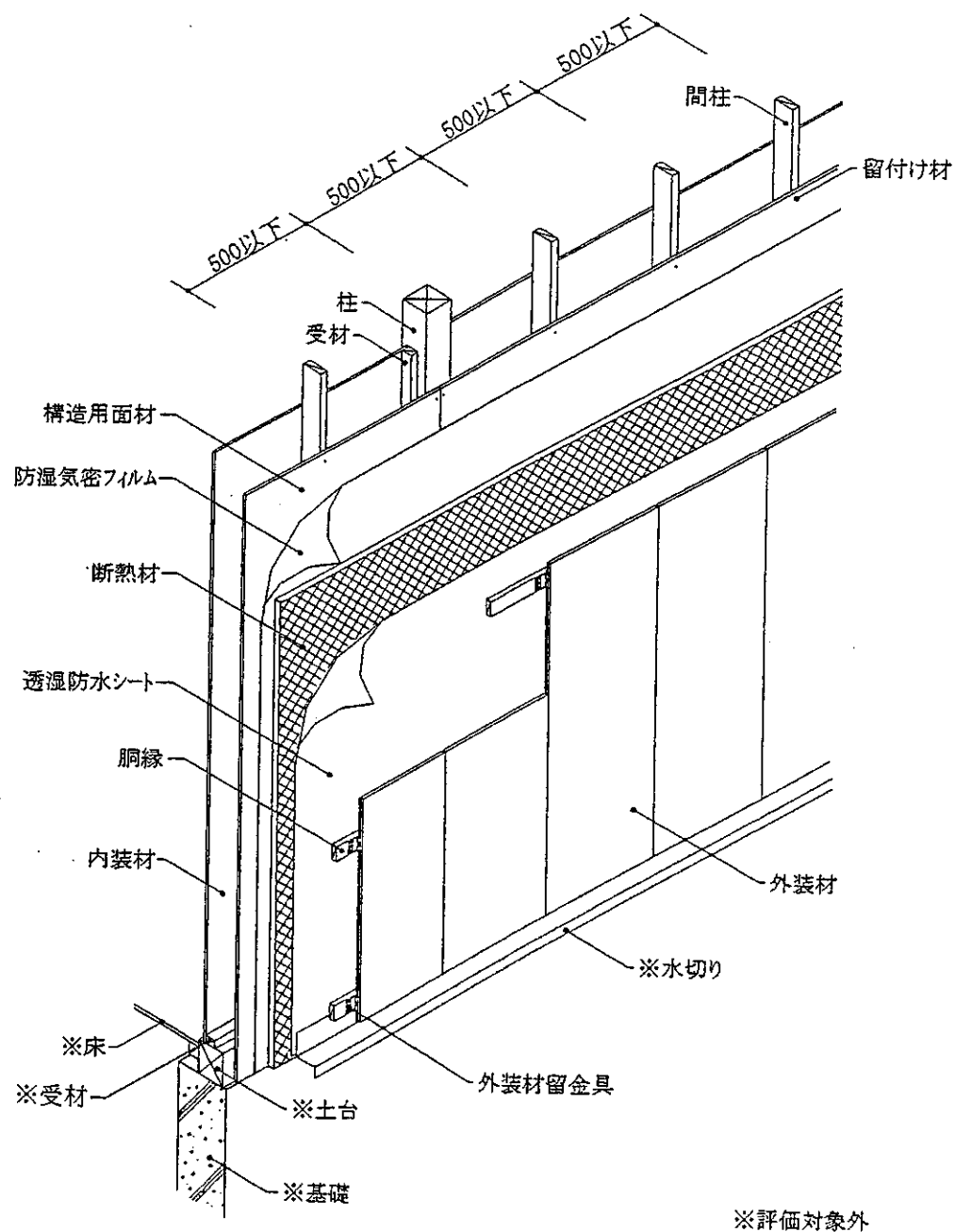
透視図
