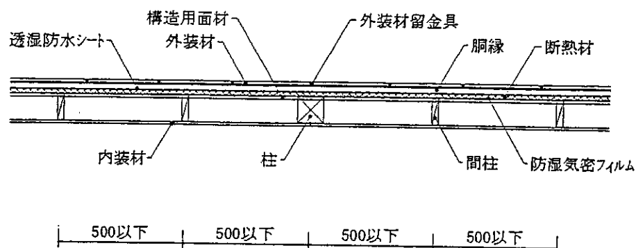
水平断面図
