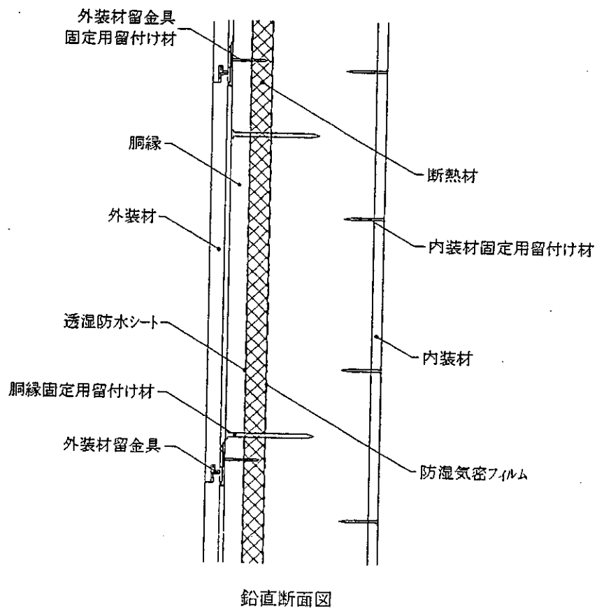
図 2 1 構造説明図
