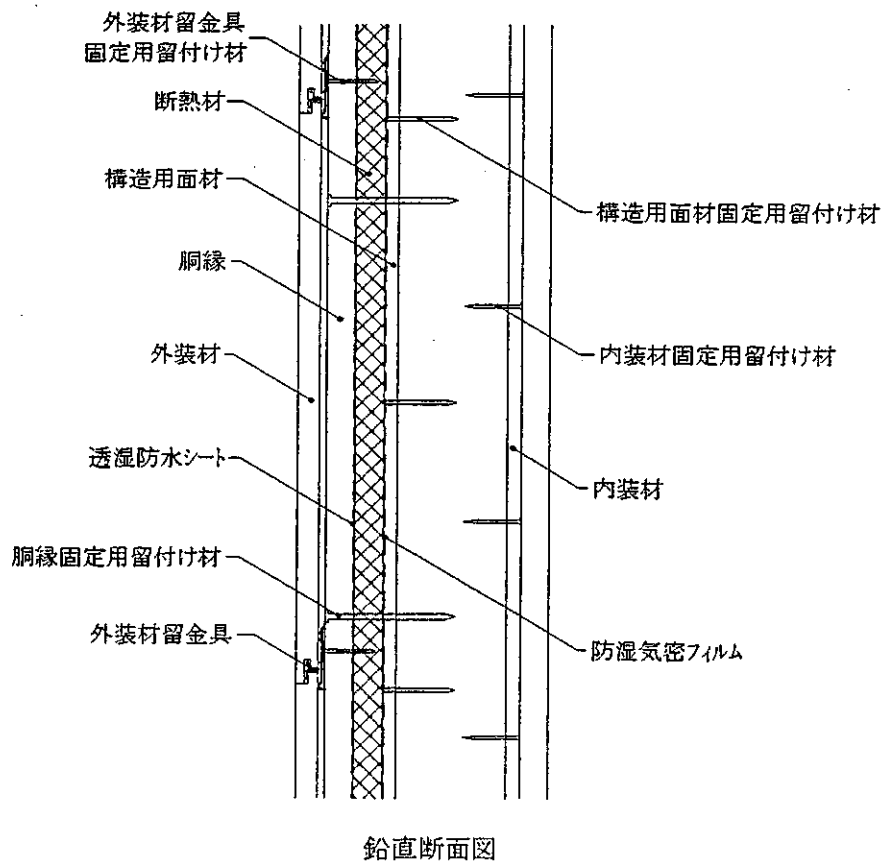
図 1 9 構造説明図
