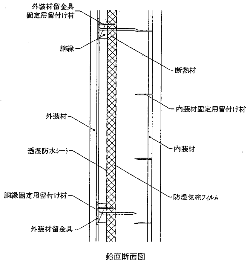
図 1 8 構造説明図
