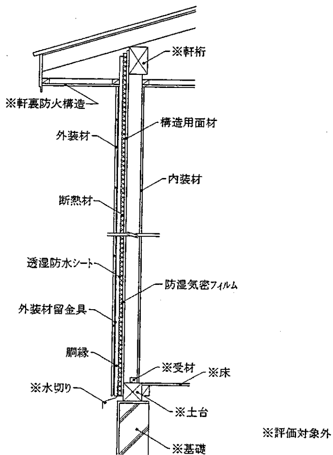
鉛直断面図
