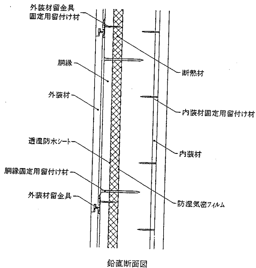
図 1 7 構造説明図
