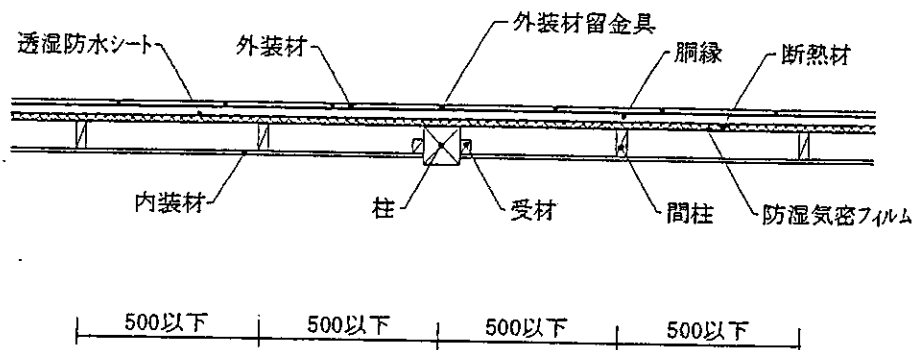
水平断面図
