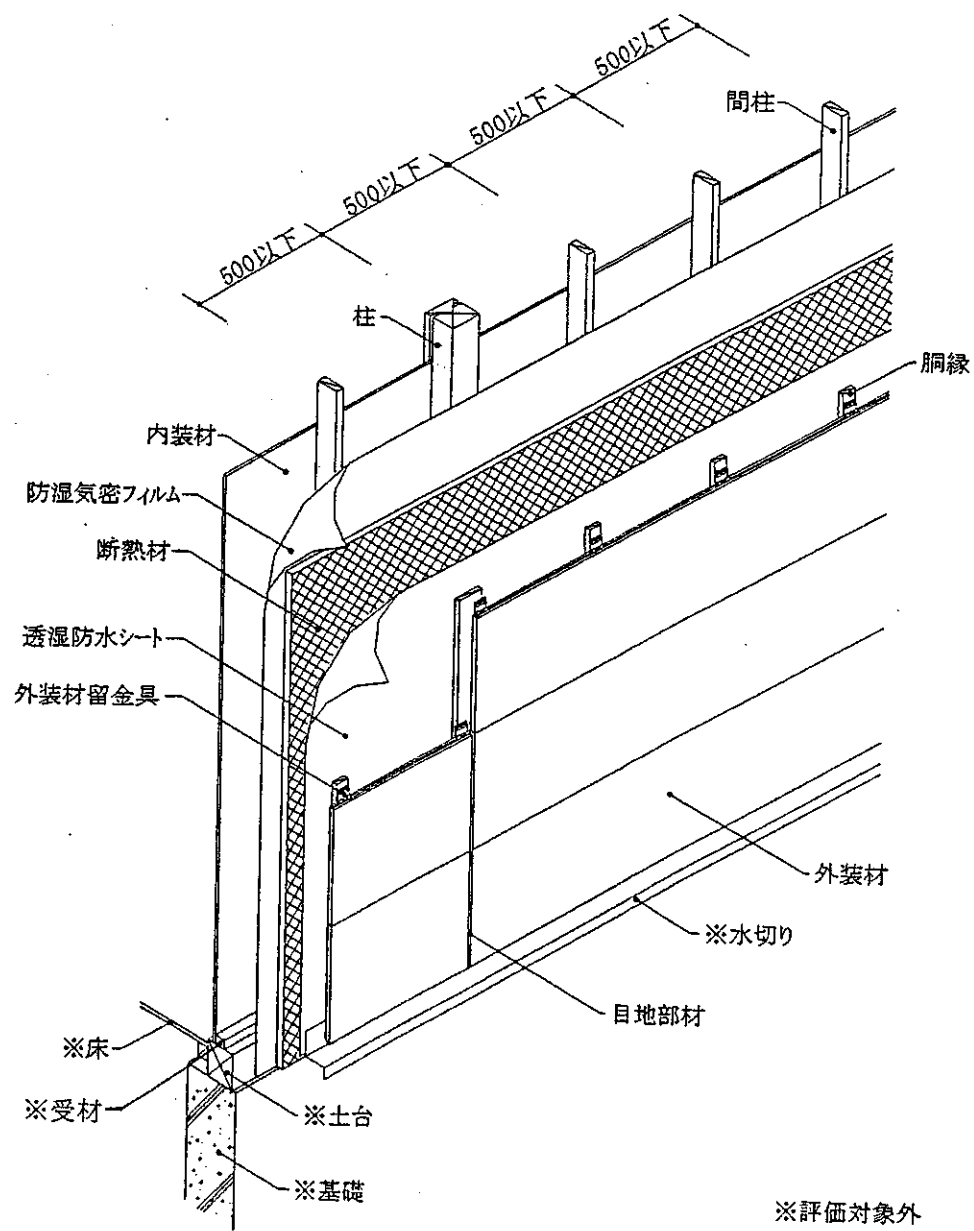
透視図
