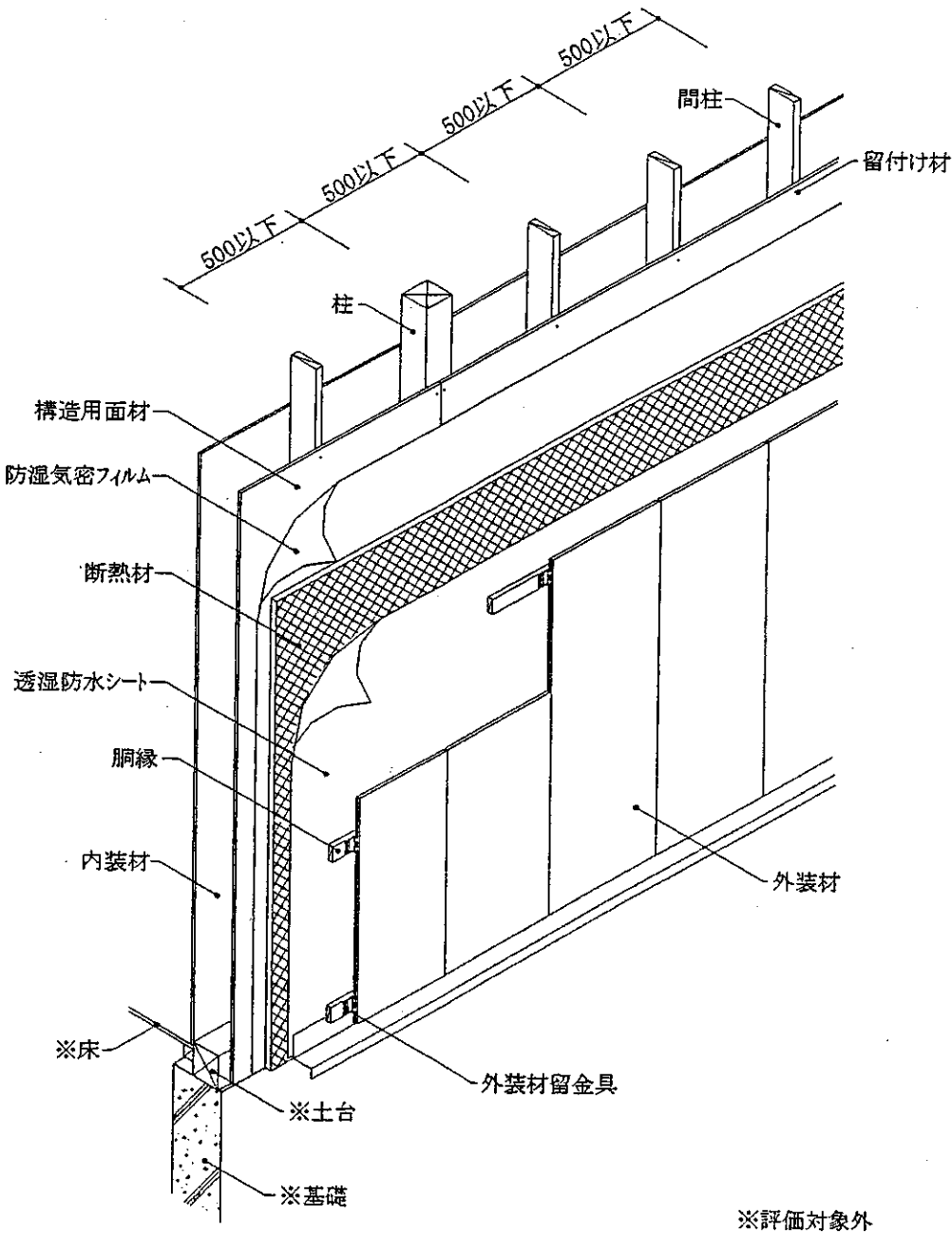
透視図
