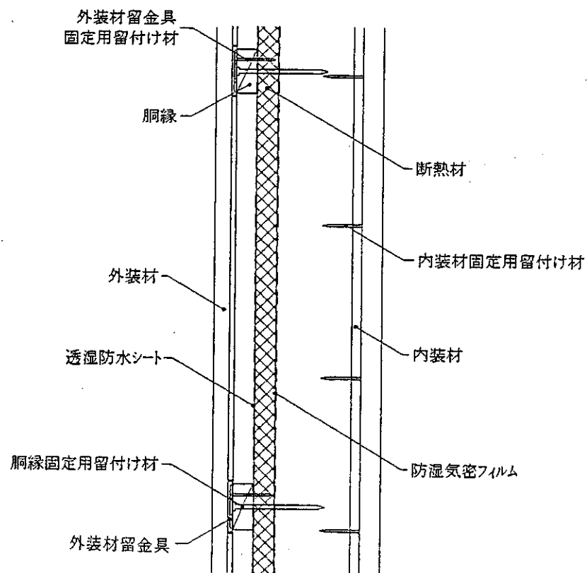
鉛直断面図
