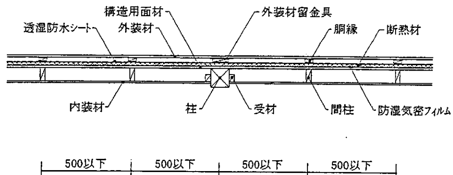
水平断面図
