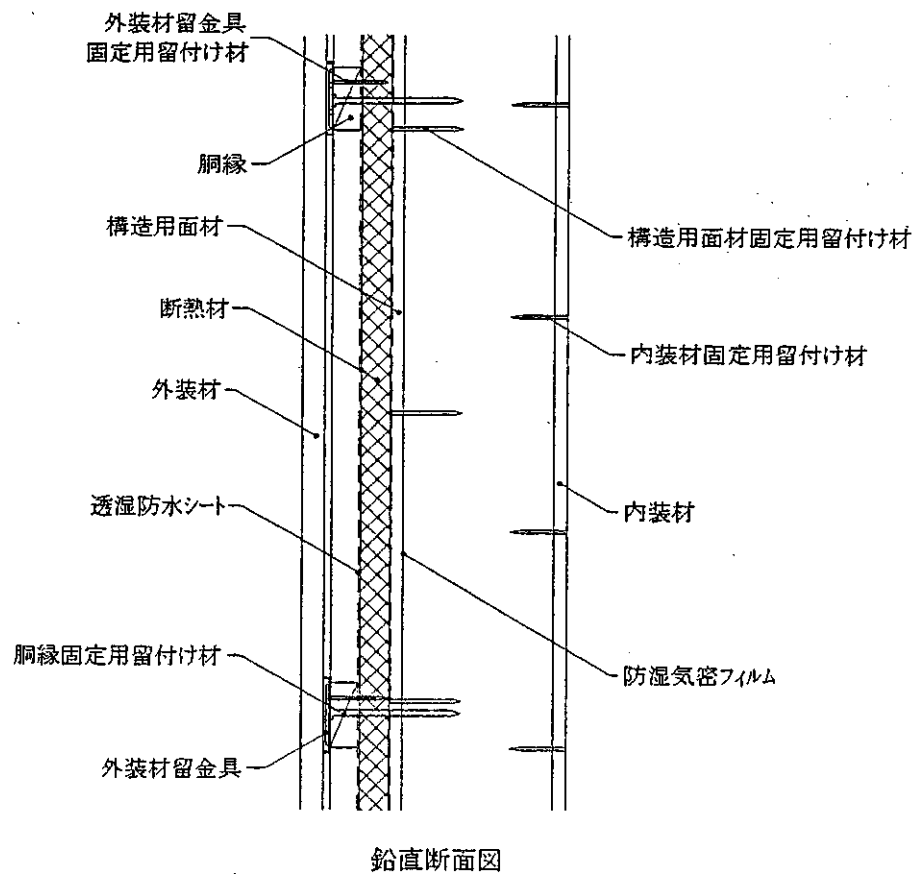
図 2 4 構造説明図
