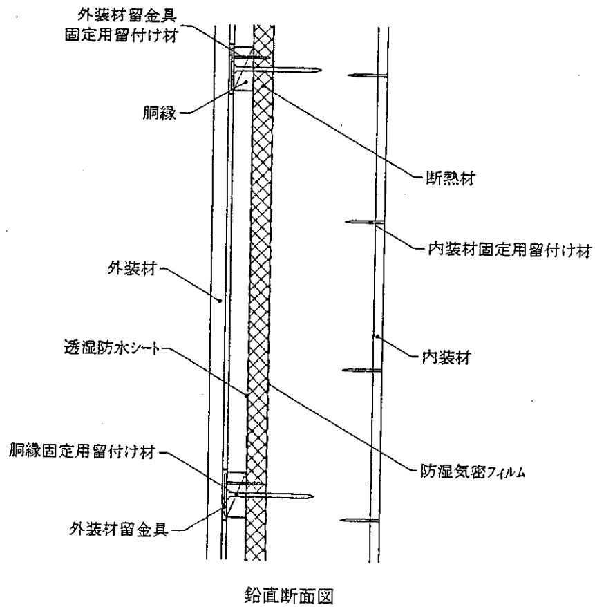
図 2 2 構造説明図
