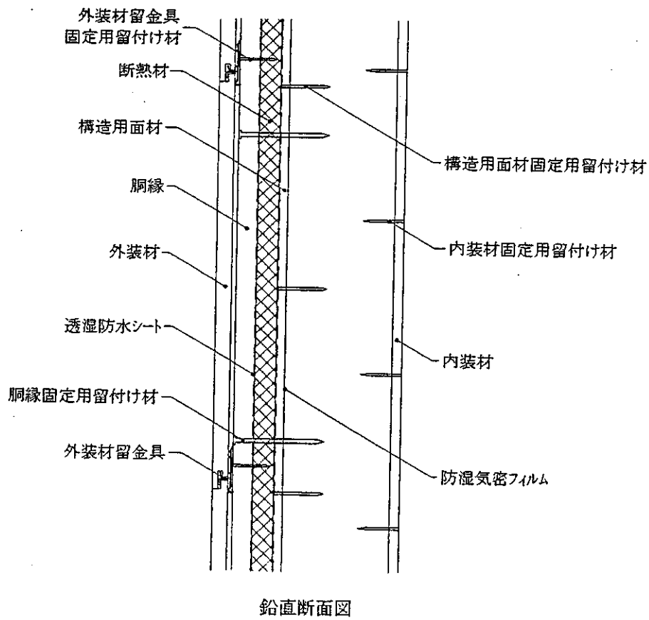
図 2 3 構造説明図
