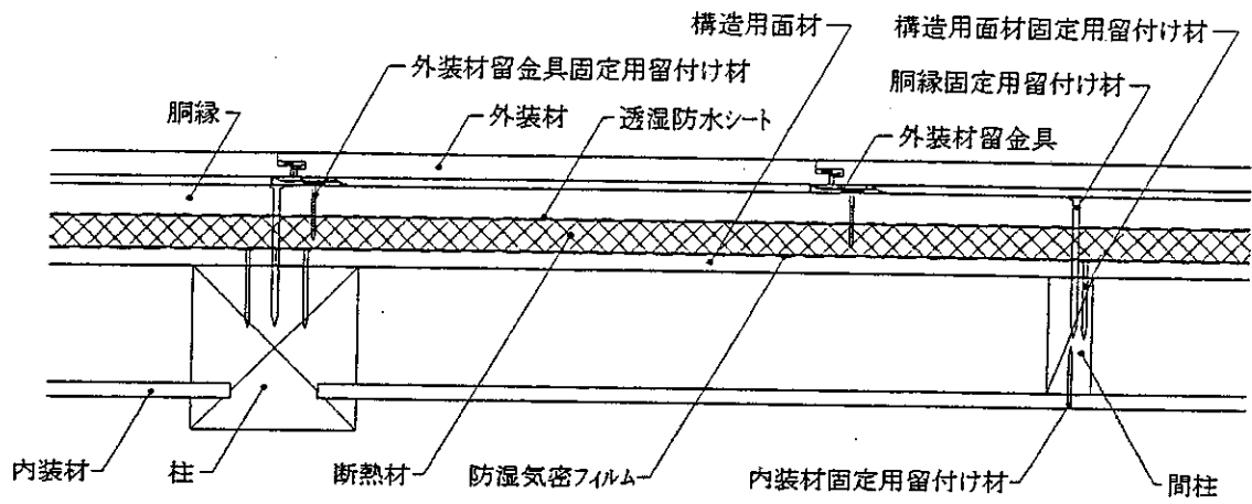
水平断面図
