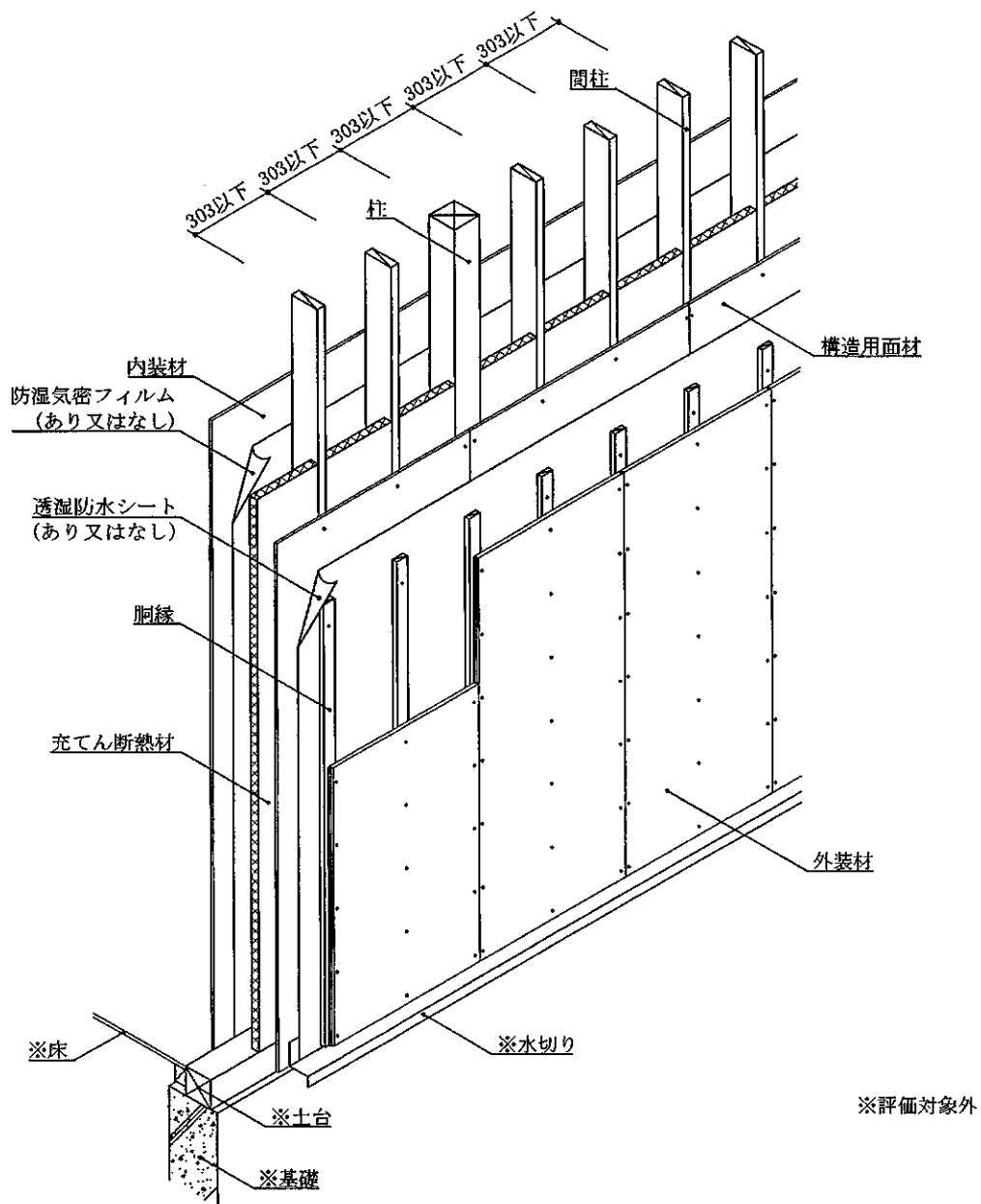
透視図 (外装材縦張・大壁造・構造用面材あり・下張材なし仕様)
