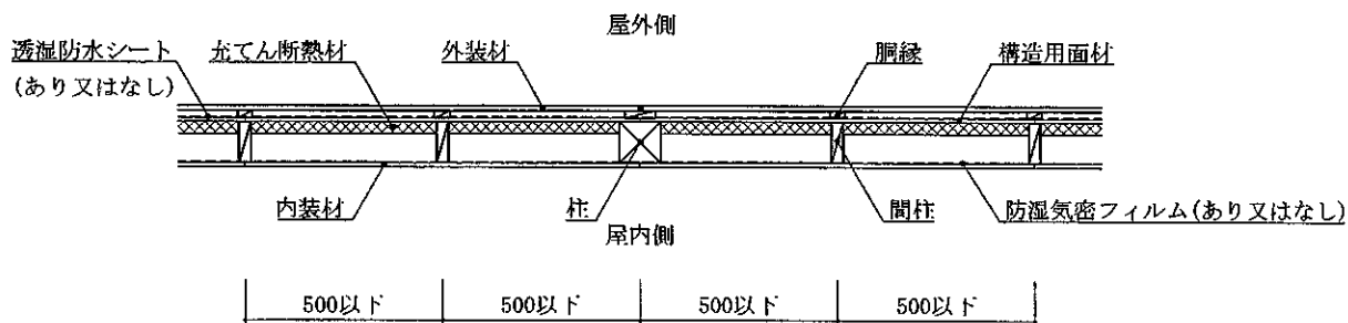
水平断面図 (外装材横張・大壁造・構造用面材あり・下張材なし仕様)
