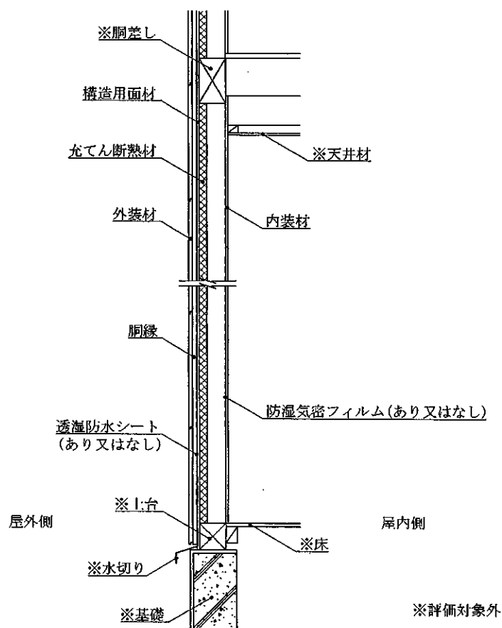
鉛直断面図 (外装材横張・大壁造・構造用面材あり・下張材なし仕様)
