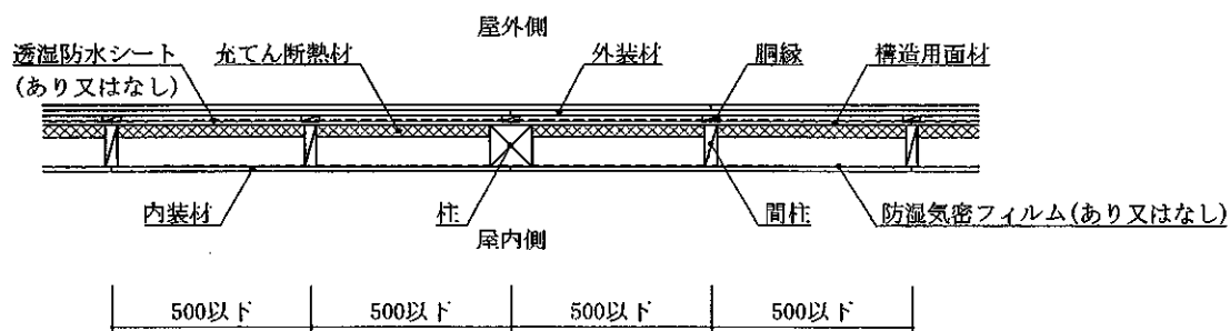
水平断面図 (外装材重張・大壁造・構造用面材あり・下張材なし仕様)
