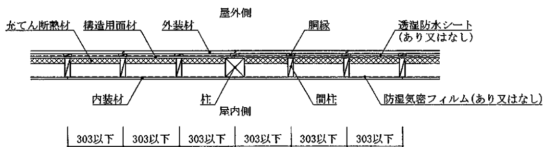
水平断面図 (外装材縦張・大壁造・構造用面材あり・下張材なし仕様)
