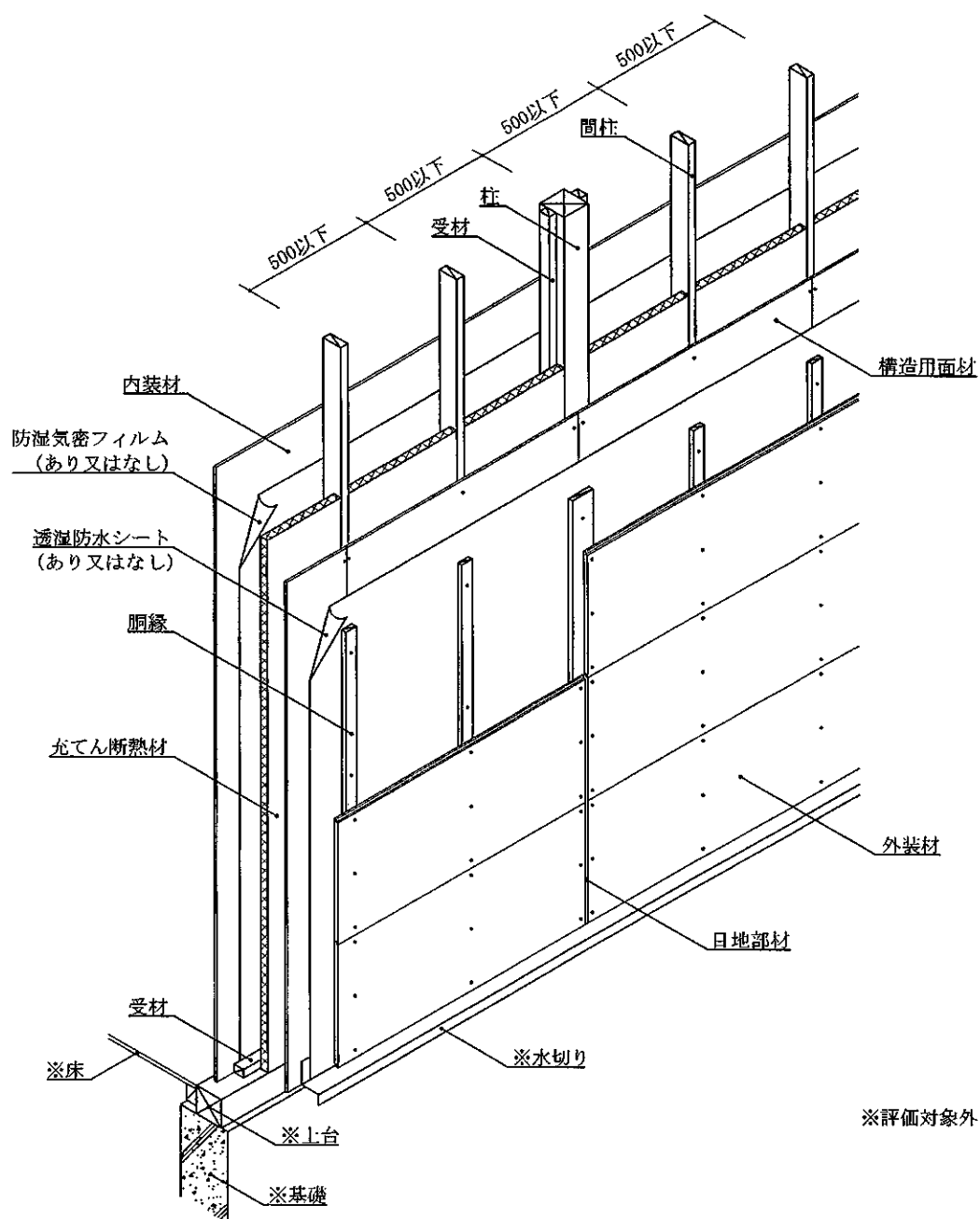
透視図 (外装材横張・受材真壁造・構造用面材あり・下張材なし仕様)
