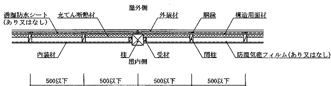
水平断面図 (外装材横張・受材真壁造・構造用面材あり・下張材なし仕様)
