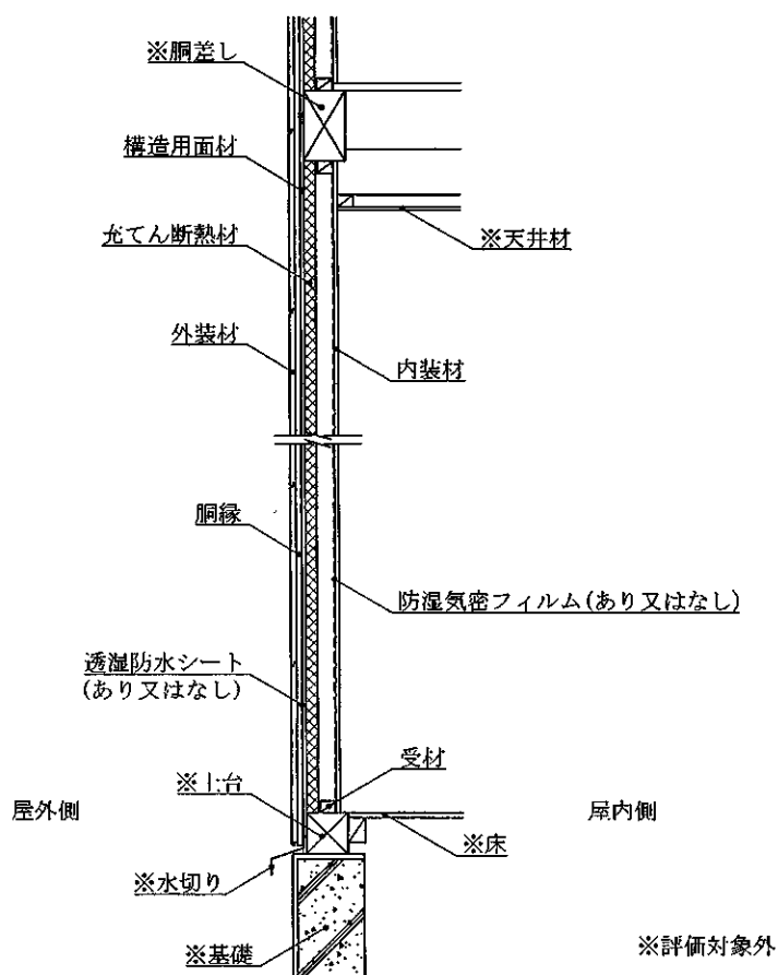
鉛直断面図 (外装材横張・欠き込み真壁造・構造用面材あり・下張材なし仕様)
