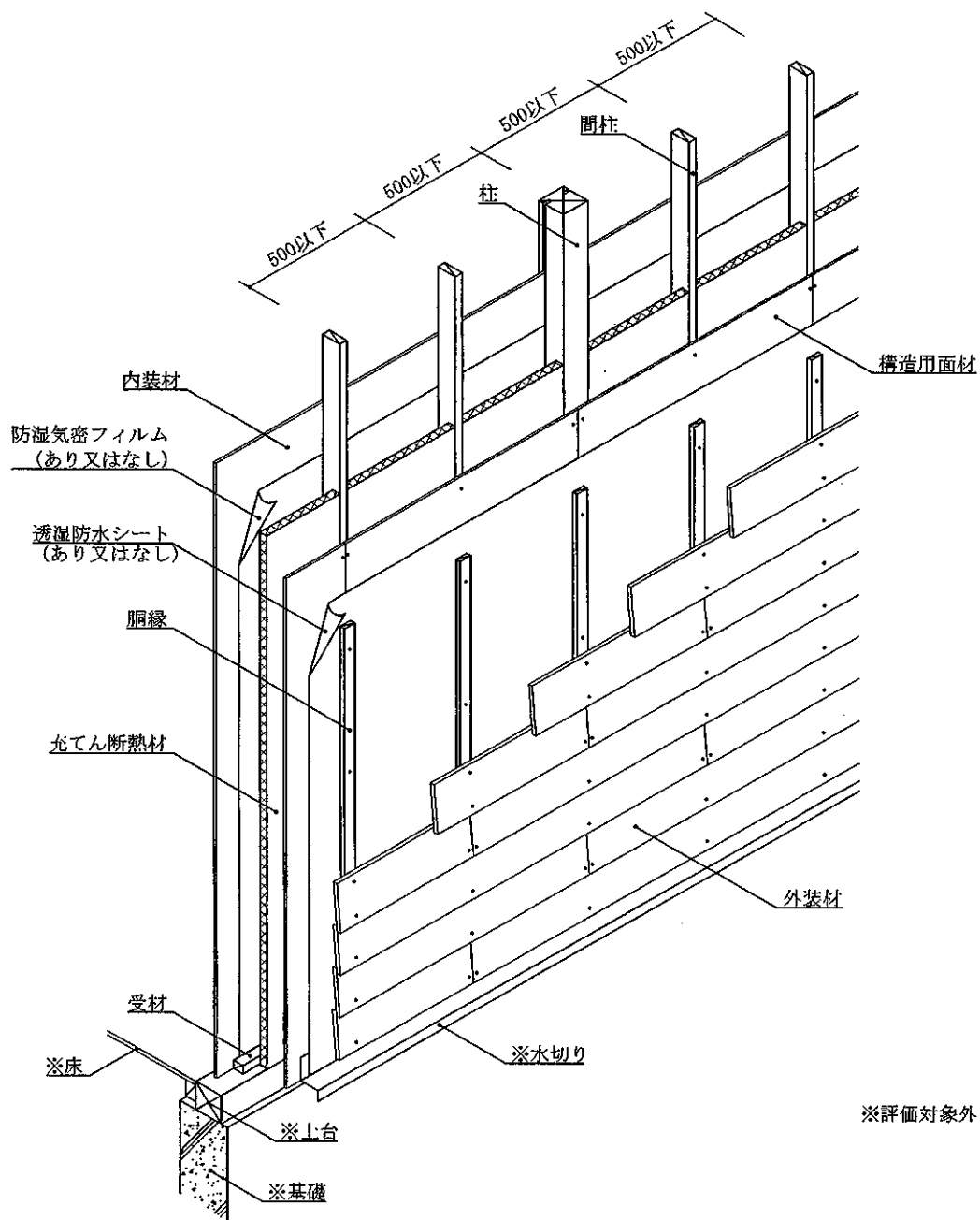
透視図 (外装材重張・欠き込み真壁造・構造用面材あり・下張材なし仕様)
