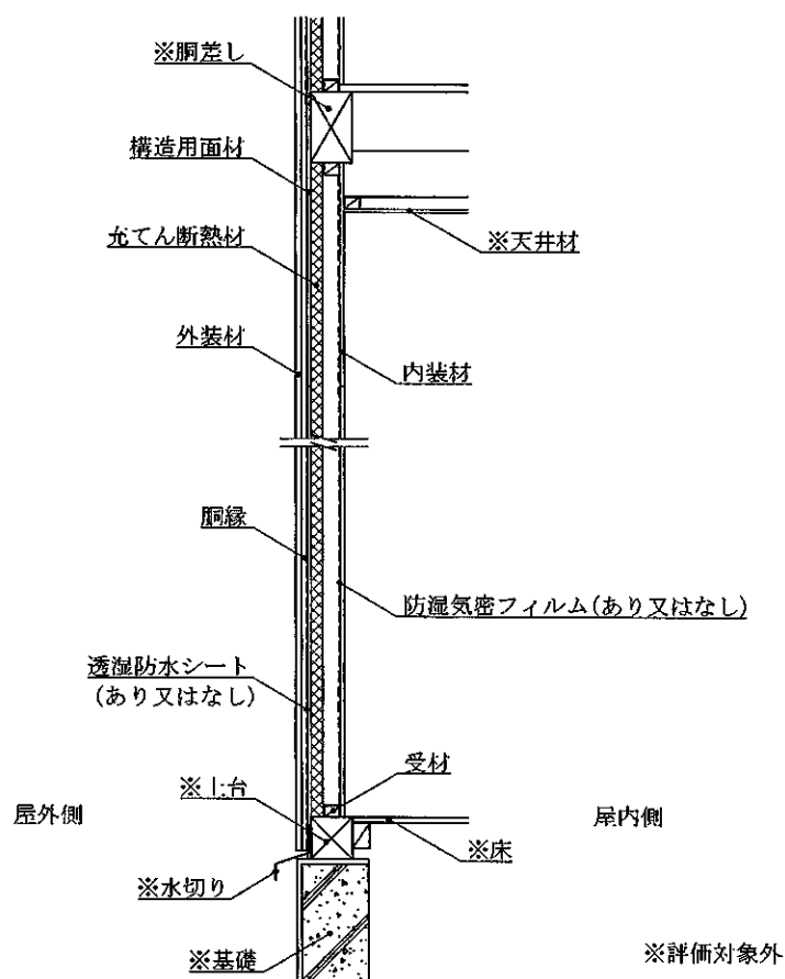
鉛直断面図 (外装材縦張・欠き込み真壁造・構造用面材あり・下張材なし仕様)
