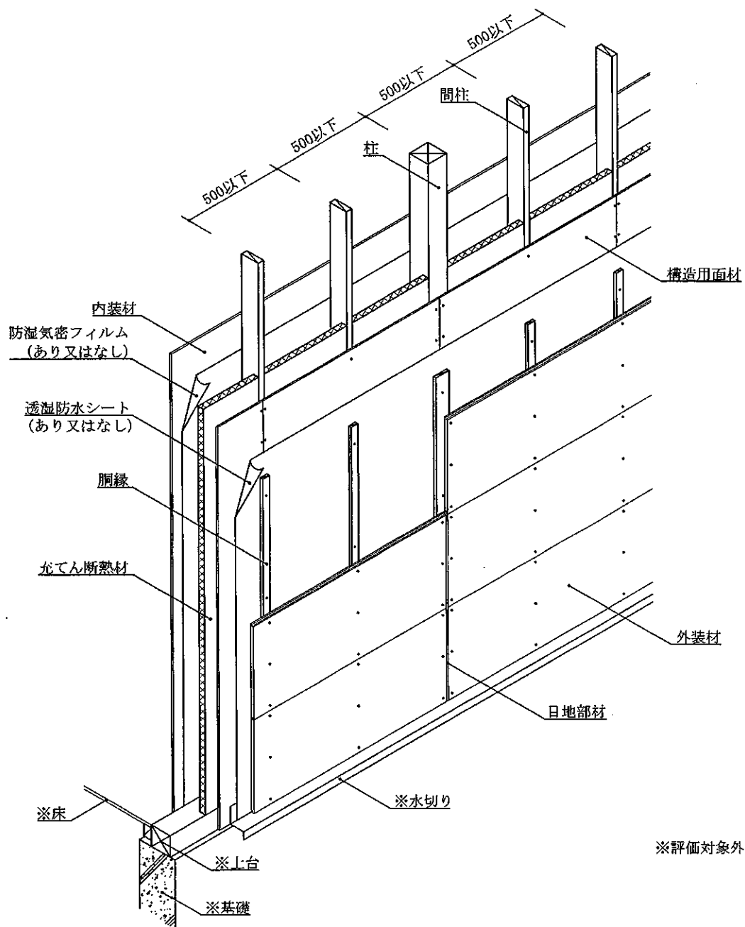
透視図 (外装材横張・大壁造・構造用面材あり・下張材なし仕様)
