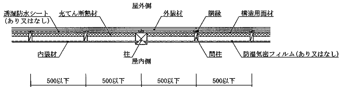
水平断面図 (外装材重張・欠き込み真壁造・構造用面材あり・下張材なし仕様)
