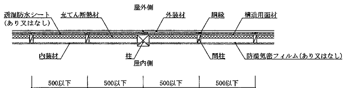
水平断面図 (外装材横張・欠き込み真壁造・構造用面材あり・下張材なし仕様)
