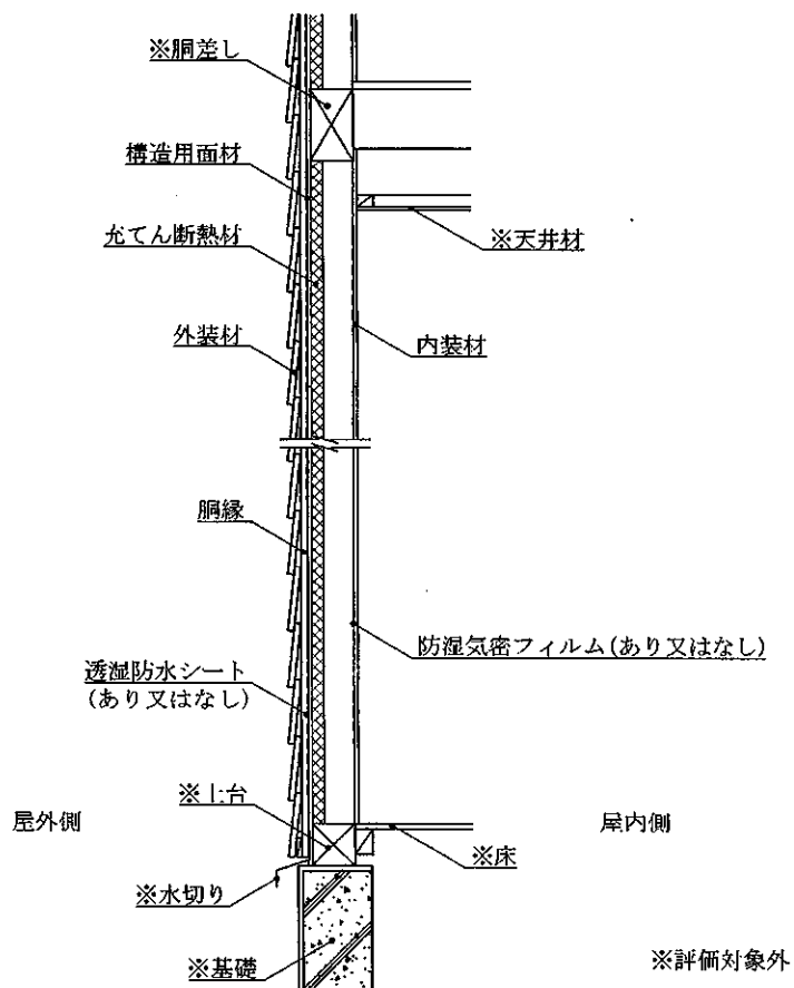
鉛直断面図 (外装材重張・大壁造・構造用面材あり・下張材なし仕様)
