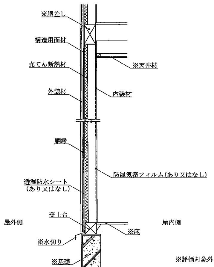
鉛直断面図 (外装材縦張・大壁造・構造用面材あり・下張材なし仕様)
