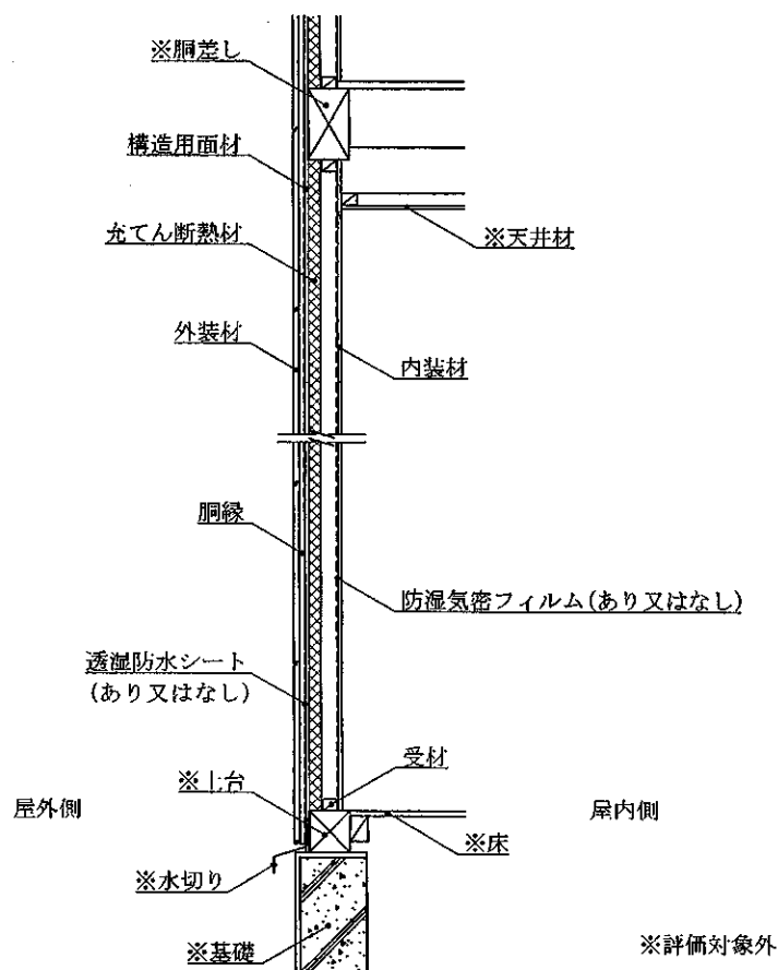
鉛直断面図 (外装材横張・受材真壁造・構造用面材あり・下張材なし仕様)
