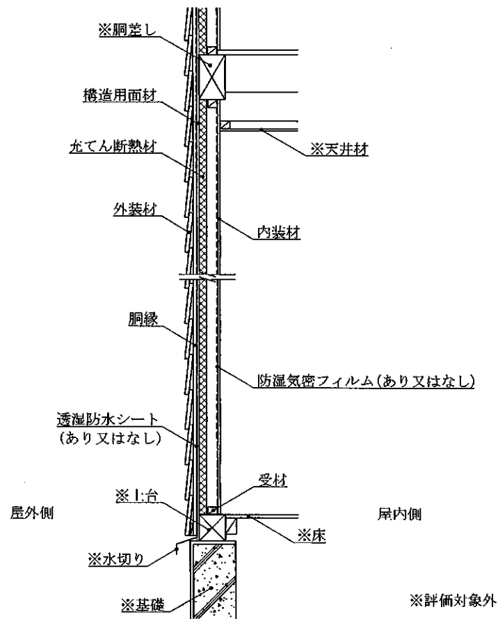
鉛直断面図 (外装材重張・欠き込み真壁造・構造用面材あり・下張材なし仕様)
