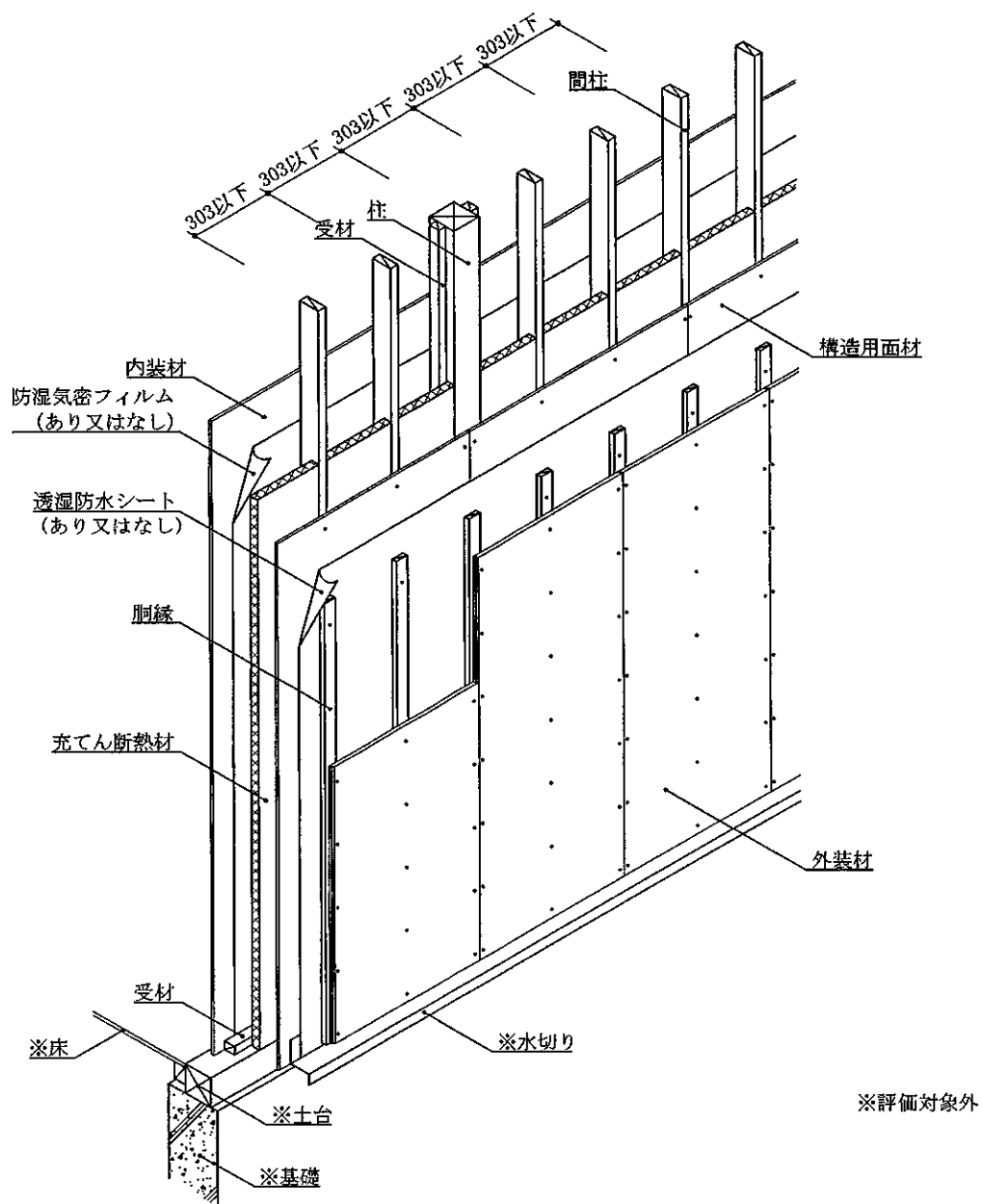
透視図 (外装材縦張・受材真壁造・構造用面材あり・下張材なし仕様)
