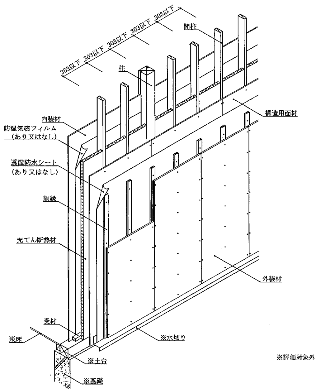
透視図 (外装材縦張・欠き込み真壁造・構造用面材あり・下張材なし仕様)
