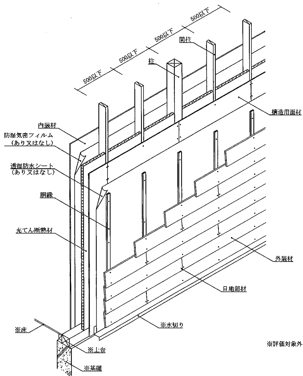
透視図 (外装材重張・大壁造・構造用面材あり・下張材なし仕様)
