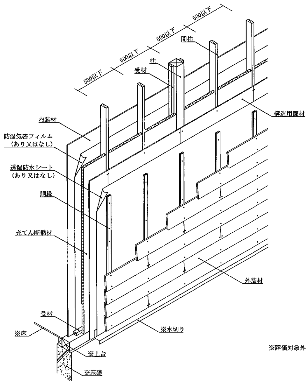
透視図 (外装材重張・受材真壁造・構造用面材あり・下張材なし仕様)
