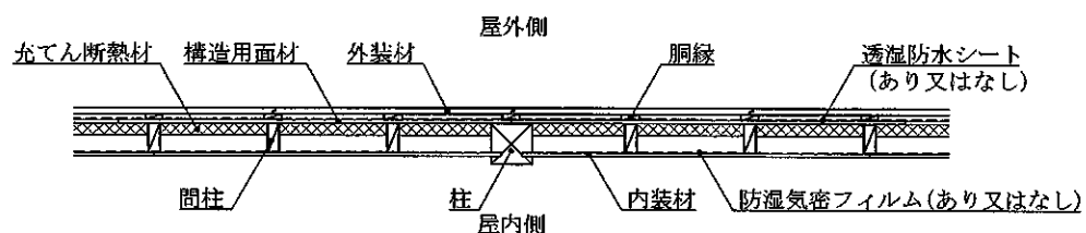
水平断面図 (外装材縦張・欠き込み真壁造・構造用面材あり・下張材なし仕様)
