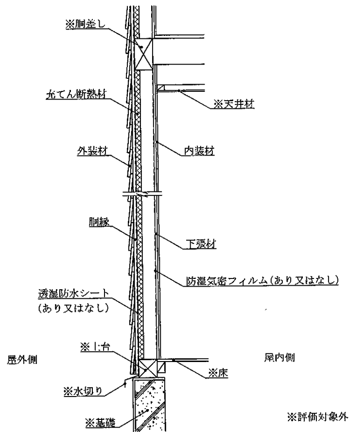
鉛直断面図 (外装材重張・大壁造・構造用面材なし・下張材あり仕様)
