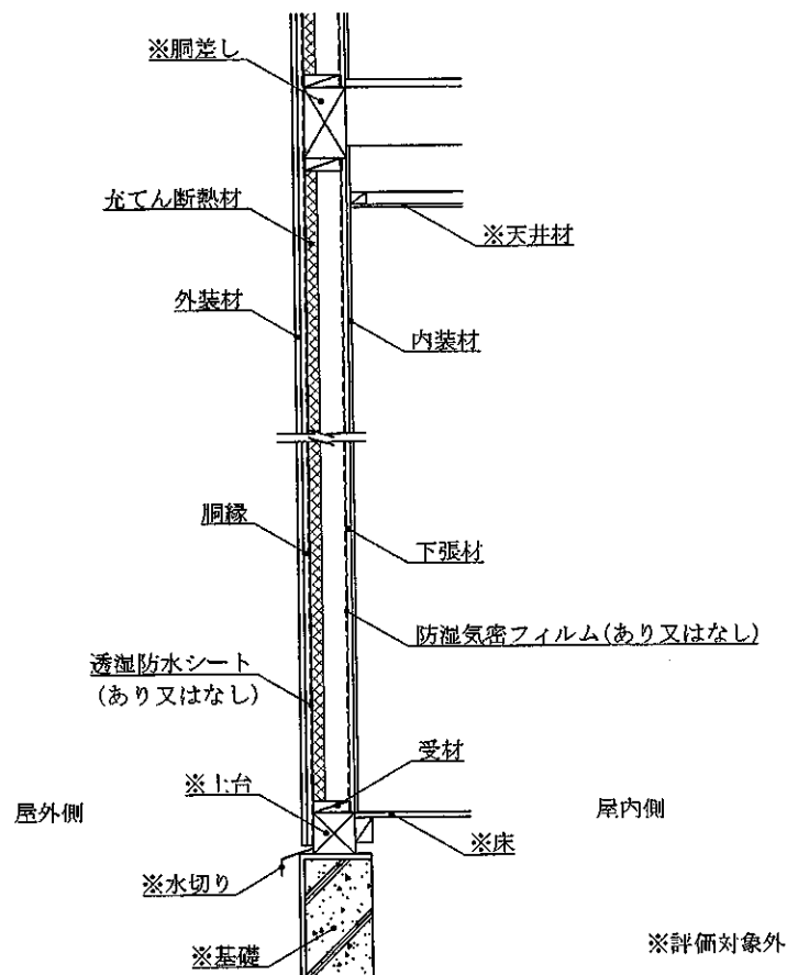
鉛直断面図 (外装材縦張・受材大壁造1・構造用面材なし・下張材あり仕様)
