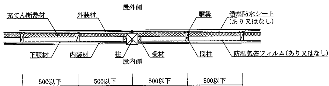
水平断面図 (外装材横張・受材真壁造・構造用面材なし・下張材あり仕様)
