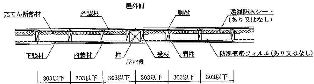
水平断面図 (外装材縦張・受材大壁造1・構造用面材なし・下張材あり仕様)
