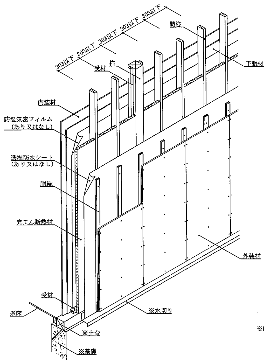
透視図 (外装材縦張・受材真壁造・構造用面材なし・下張材あり仕様)
