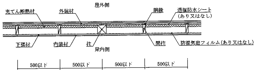
水平断面図 (外装材重張・大壁造・構造用面材なし・下張材あり仕様)
