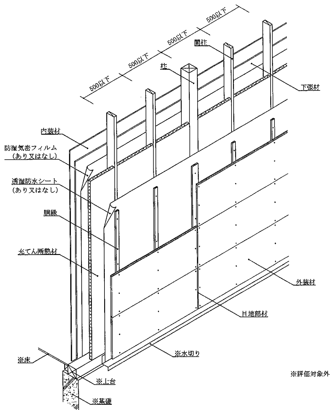
透視図 (外装材横張・大壁造・構造用面材なし・下張材あり仕様)
