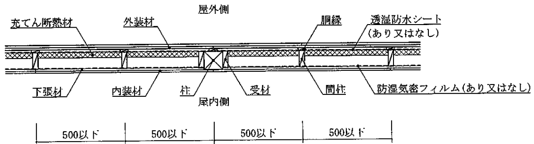
水平断面図 (外装材重張・受材大壁造1・構造用面材なし・下張材あり仕様)
