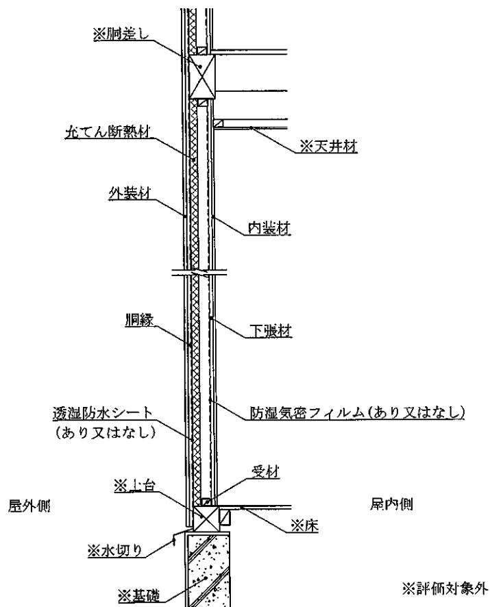
鉛直断面図
