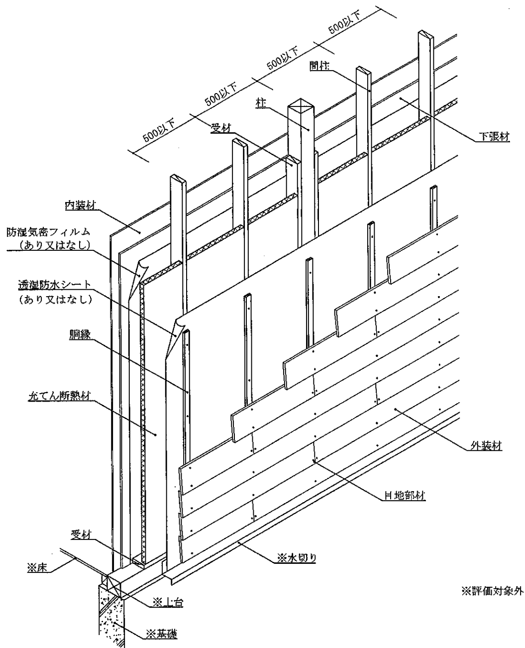
透視図 (外装材重張・受材大壁造1・構造用面材なし・下張材あり仕様)
