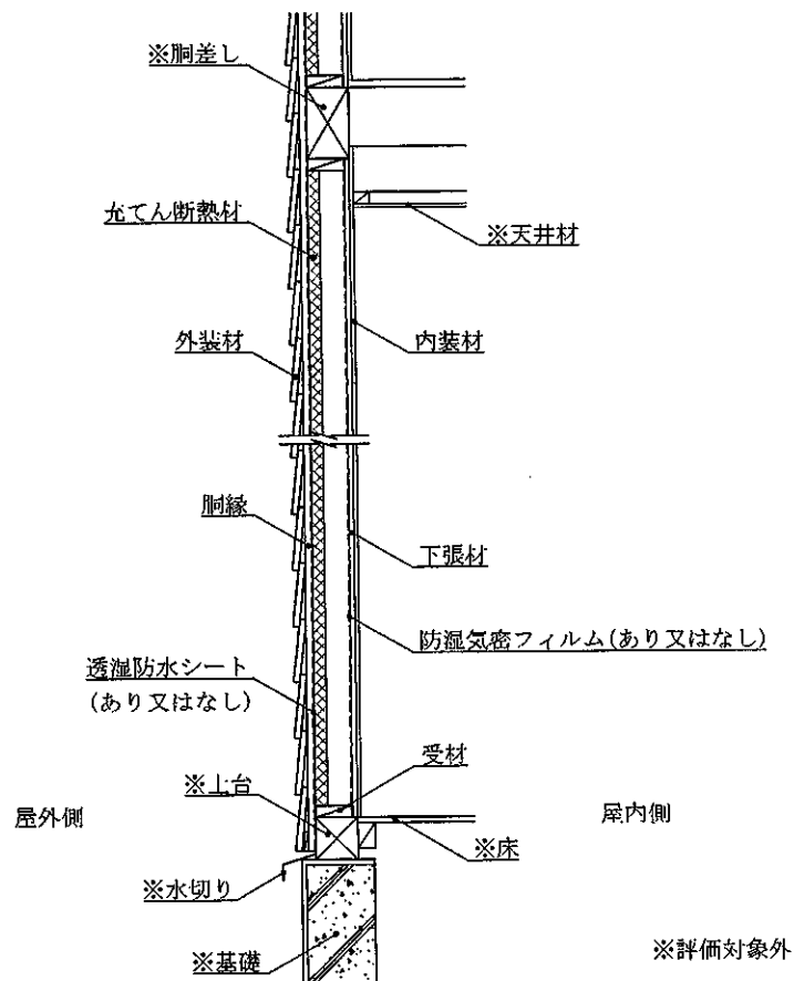
鉛直断面図 (外装材重張・受材大壁造1・構造用面材なし・下張材あり仕様)
