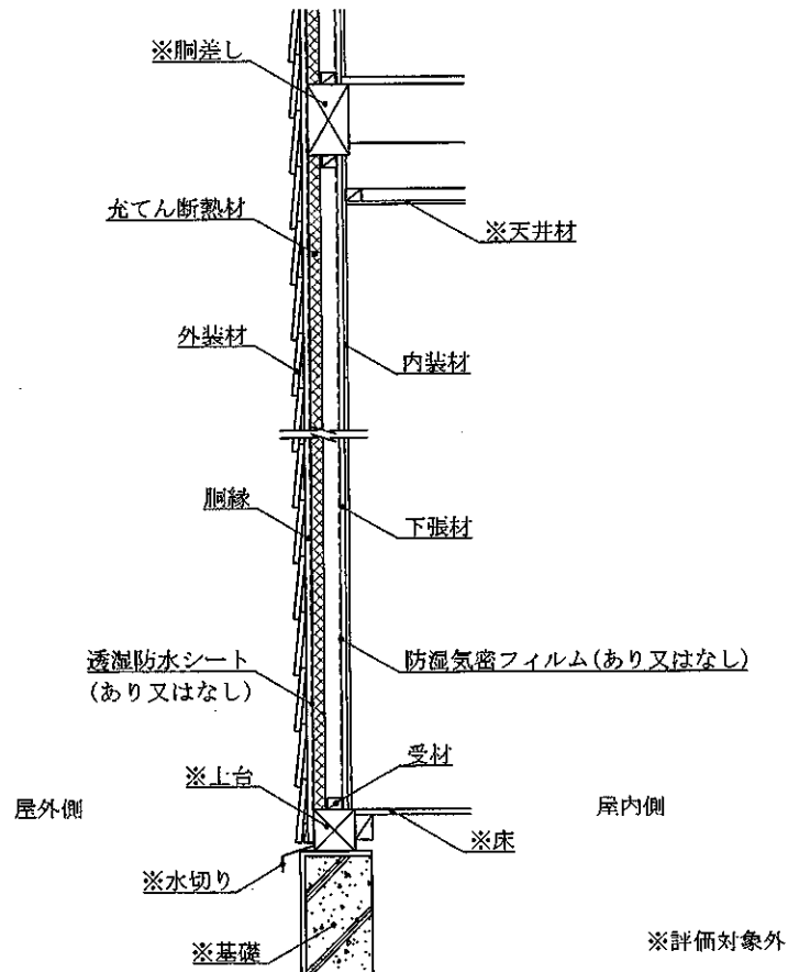
鉛直断面図 (外装材重張・受材真壁造・構造用面材なし・下張材あり仕様)
