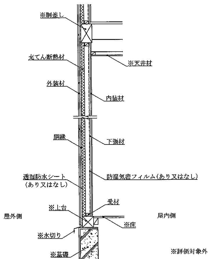
鉛直断面図 (外装材横張・受材真壁造・構造用面材なし・下張材あり仕様)
