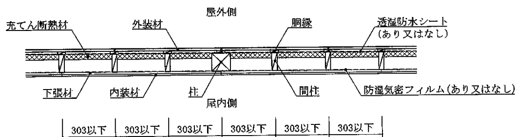
水平断面図 (外装材縦張・大壁造・構造用面材なし・下張材あり仕様)
