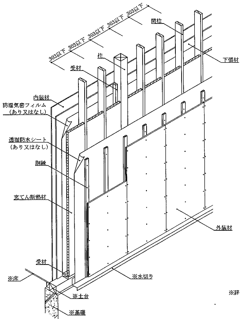
透視図 (外装材縦張・受材大壁造2・構造用面材なし・下張材あり仕様)
