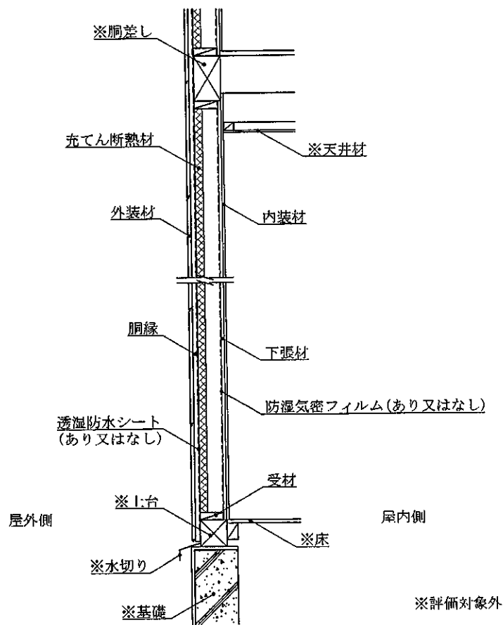
鉛直断面図 (外装材横張・受材人壁造1・構造用面材なし・下張材あり仕様)
