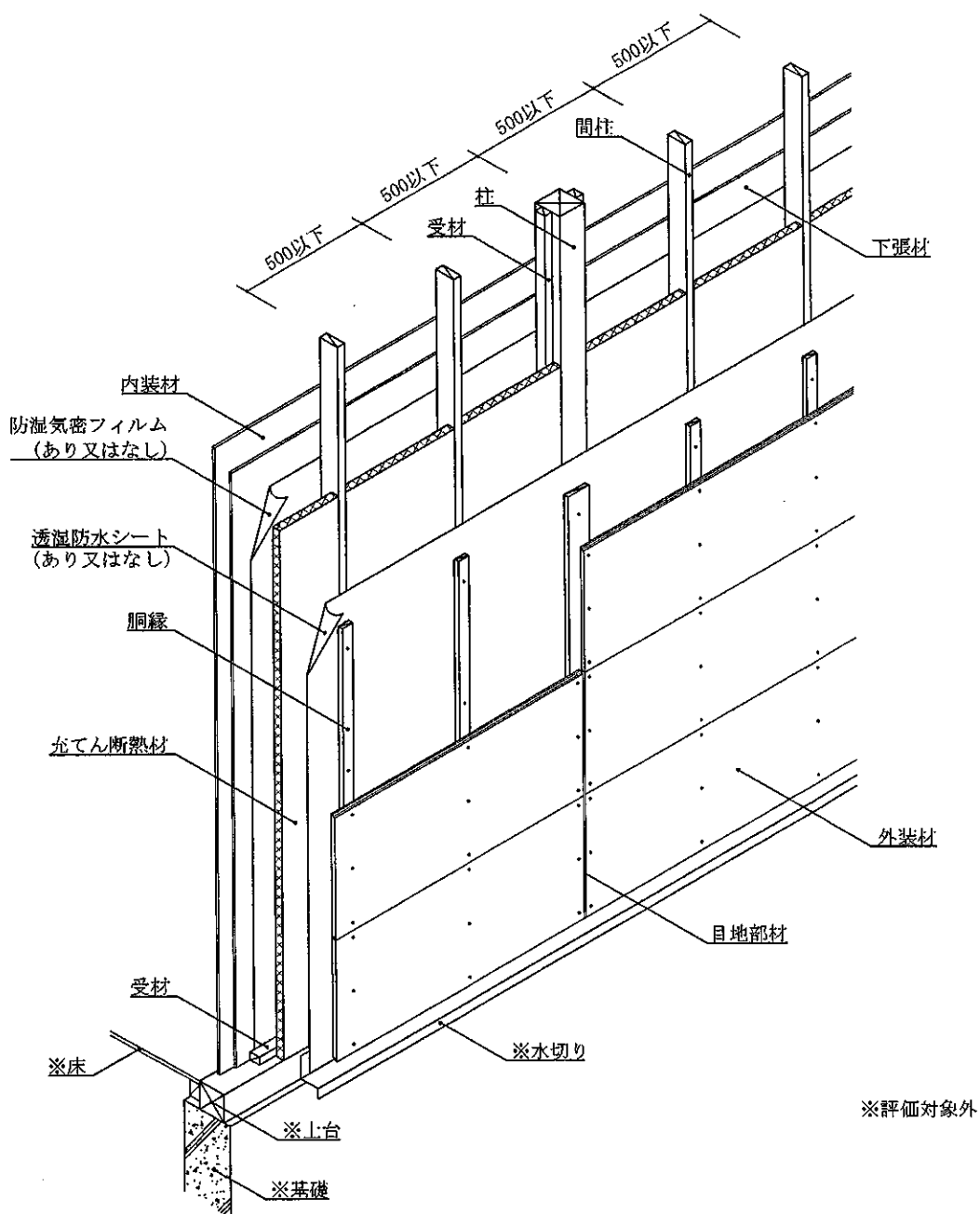
透視図 (外装材横張・受材真壁造・構造用面材なし・下張材あり仕様)
