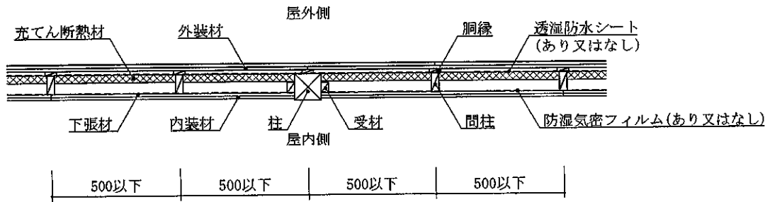
水平断面図 (外装材重張・受材真壁造・構造用面材なし・下張材あり仕様)
