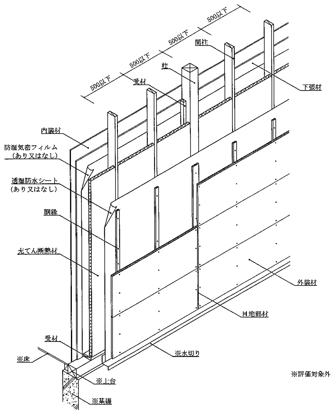
透視図 (外装材横張・受材大壁造2・構造用面材なし・下張材あり仕様)
