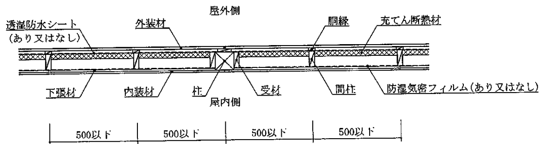
水平断面図 (外装材横張・受材人壁造1・構造用面材なし・下張材あり仕様)
