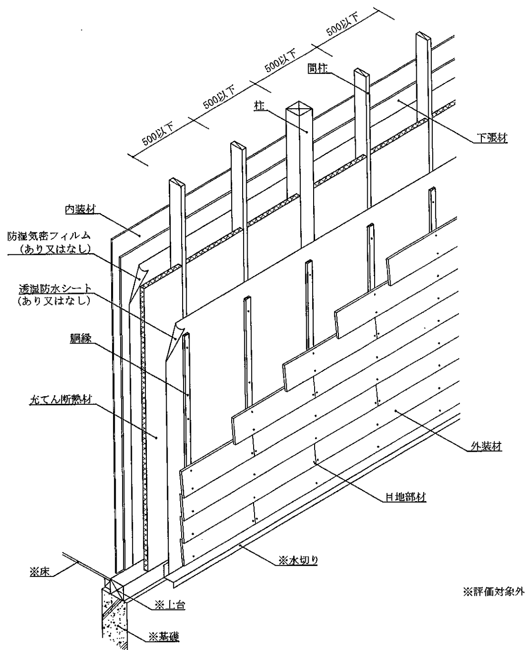
透視図 (外装材重張・大壁造・構造用面材なし・下張材あり仕様)
