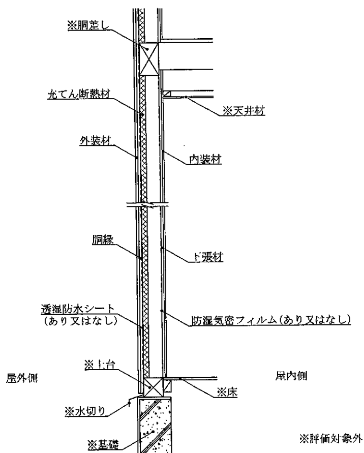
鉛直断面図 (外装材縦張・大壁造・構造用面材なし・下張材あり仕様)
