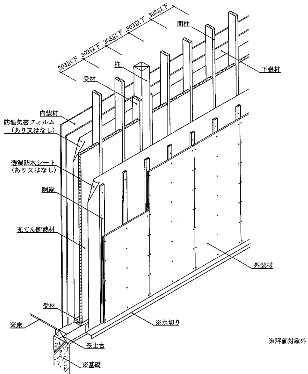
透視図 (外装材縦張・受材大壁造1・構造用面材なし・下張材あり仕様)
