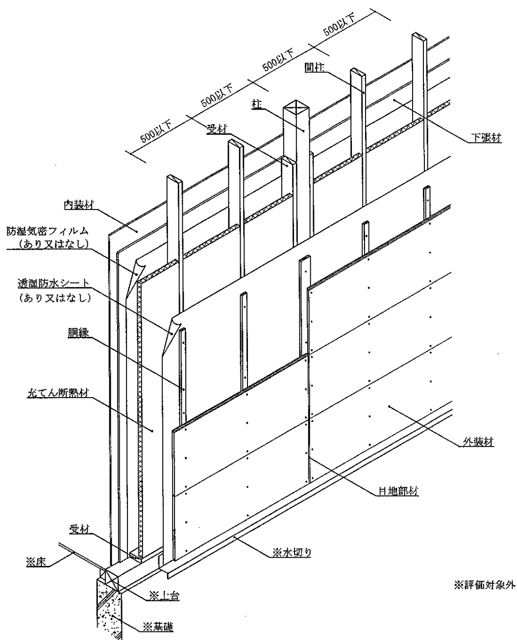
透視図 (外装材横張・受材大壁造1・構造用面材なし・下張材あり仕様)
