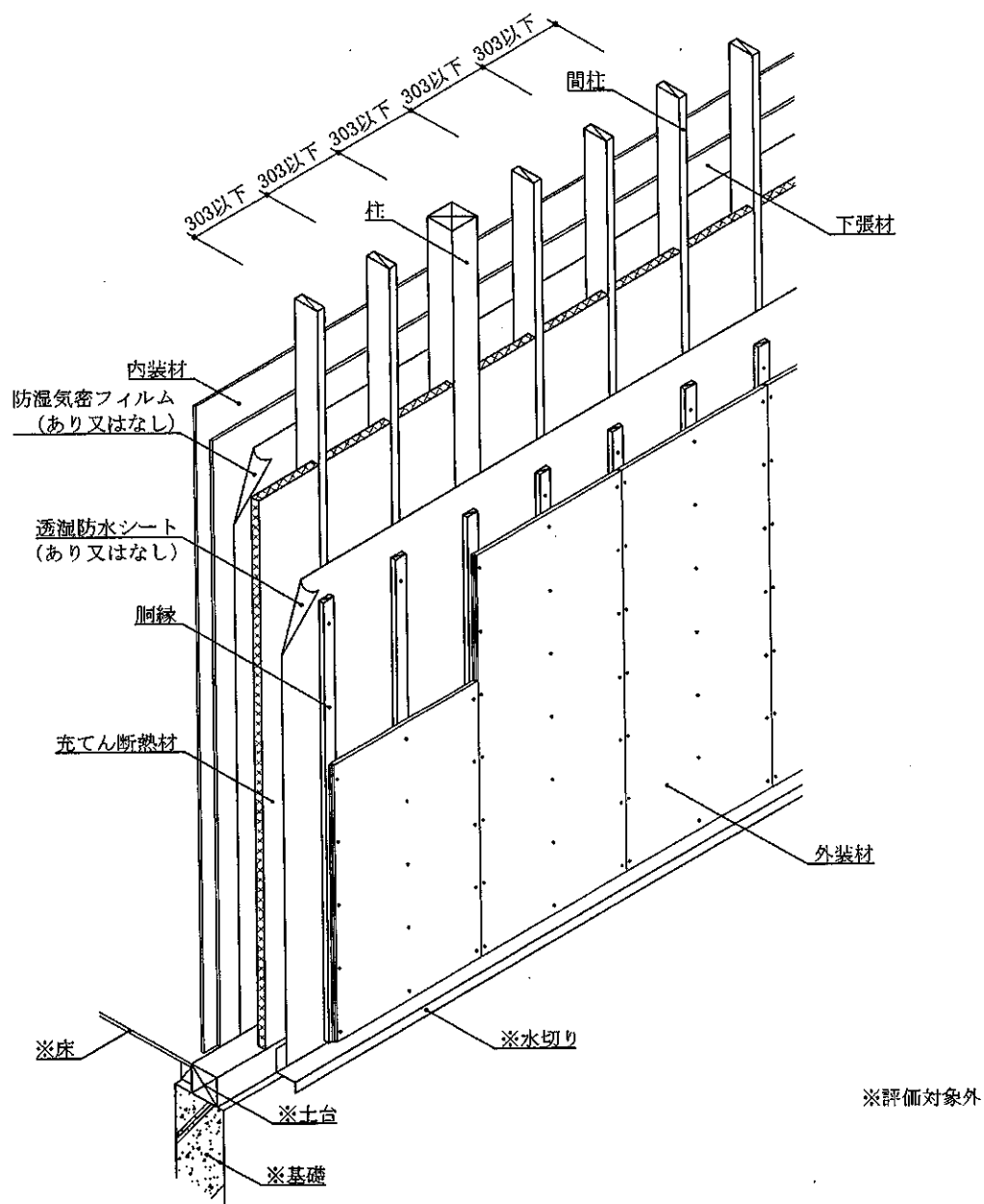
透視図 (外装材縦張・大壁造・構造用面材なし・下張材あり仕様)
