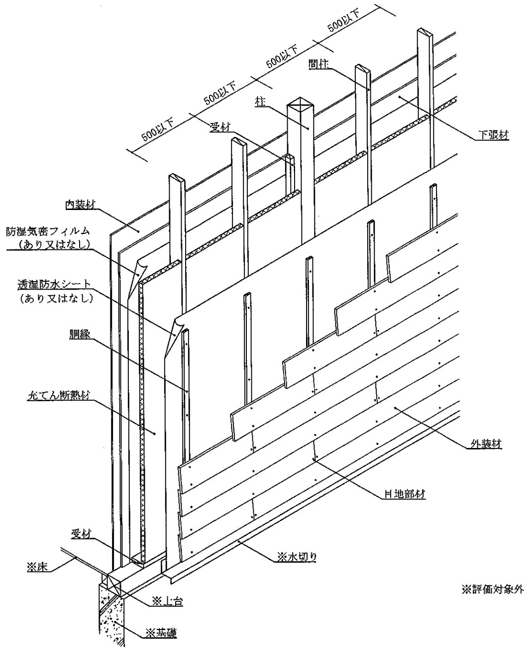
透視図 (外装材重張・受材大壁造2・構造用面材なし・下張材あり仕様)
