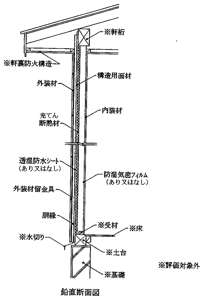
図12 施工図 (真壁造・受材仕様／構造用面材あり・下張材なし)
