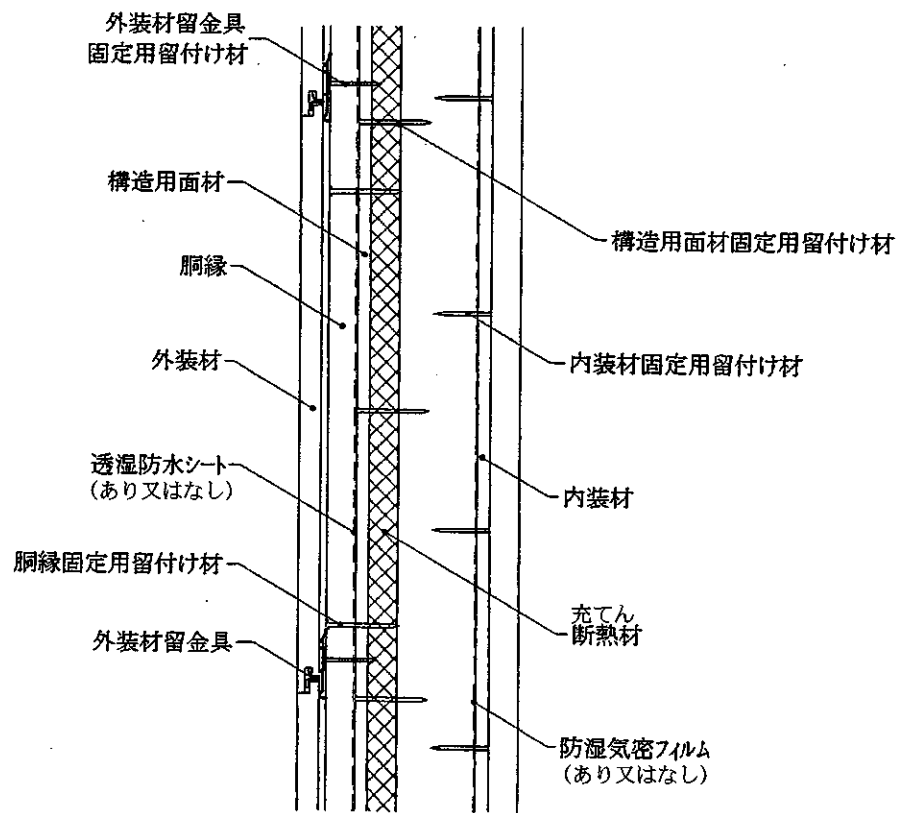
鉛直断面図
