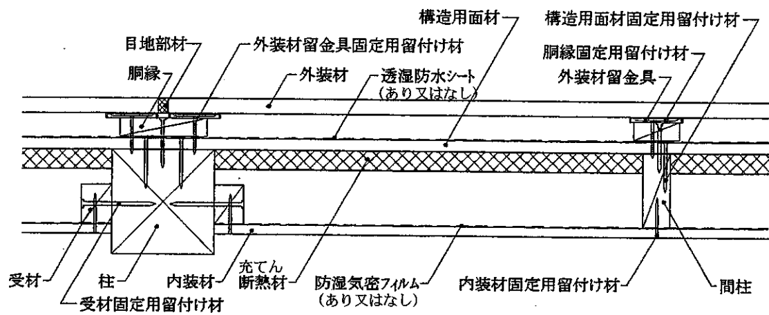
水平断面図
