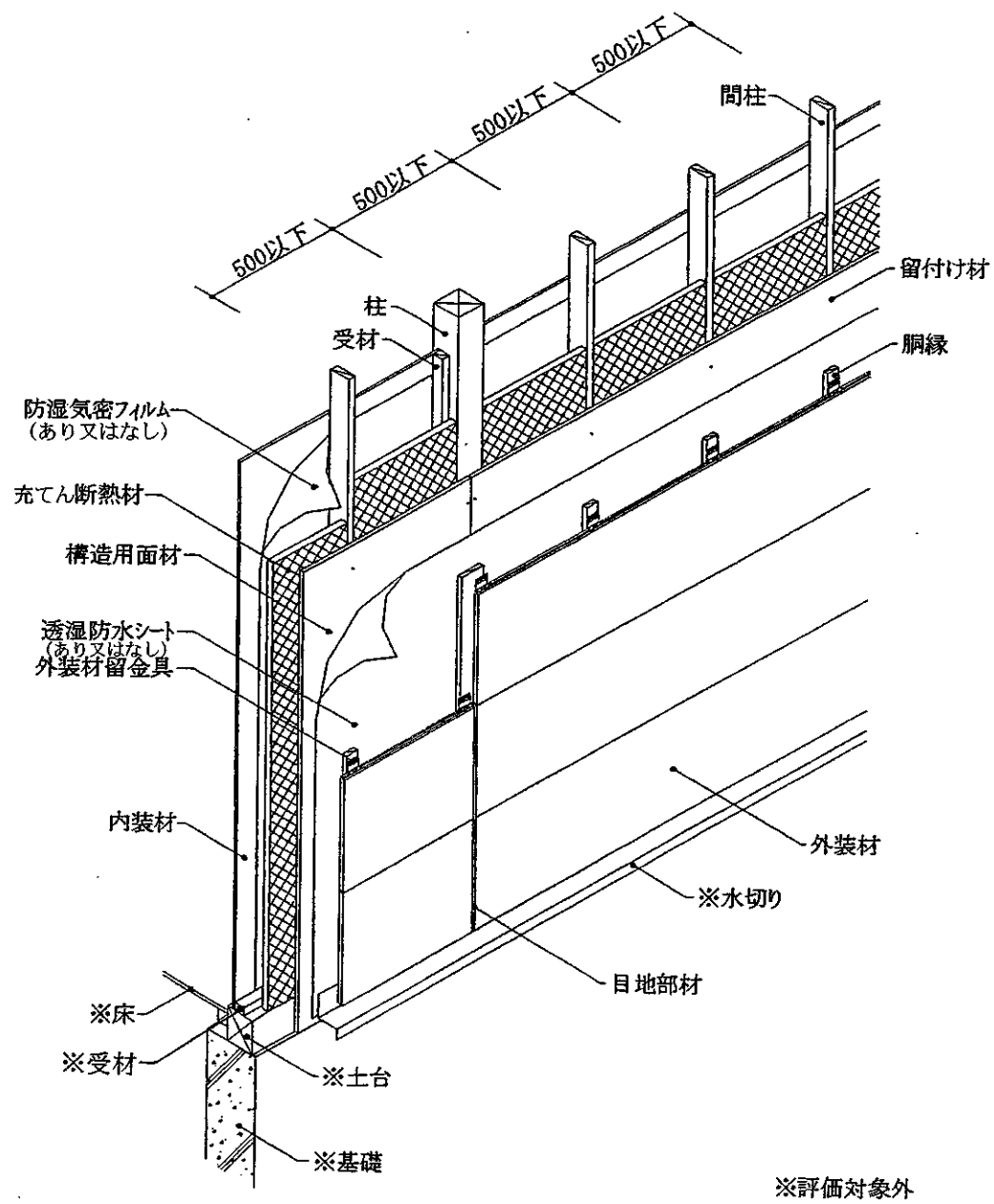
透視図
