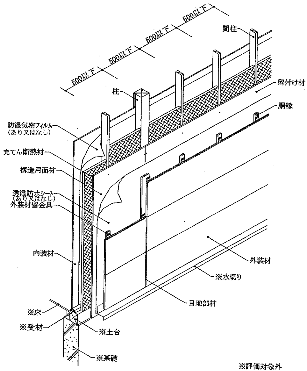
透視図
