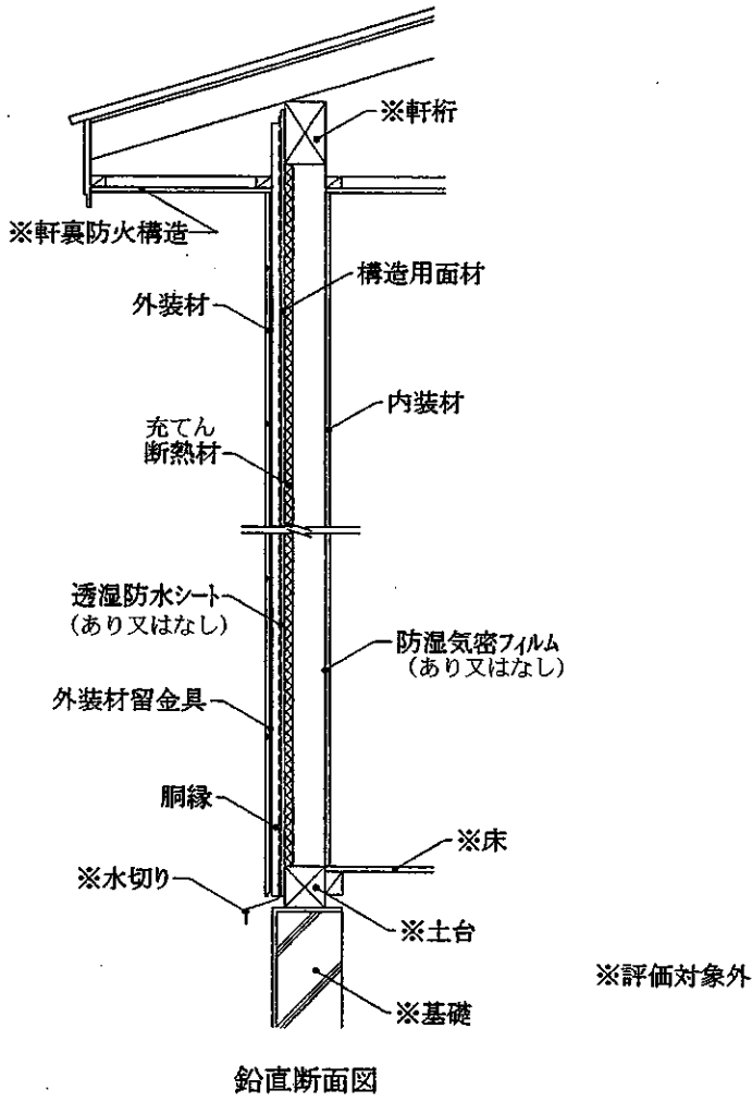
図13 施工図 (大壁造／構造用面材あり・下張材なし)
