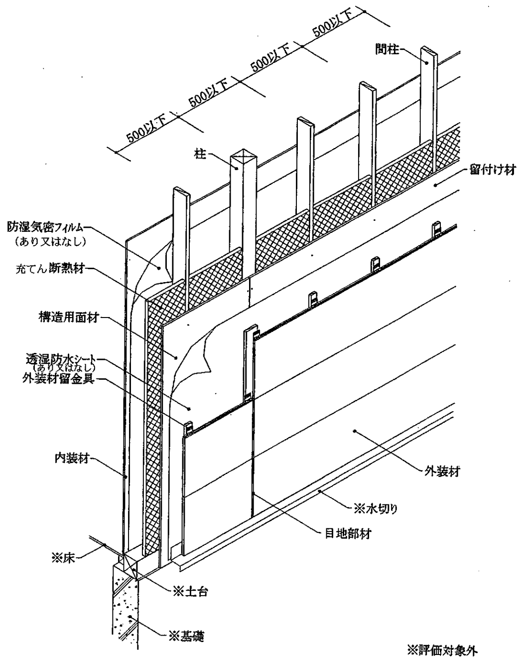
透視図
