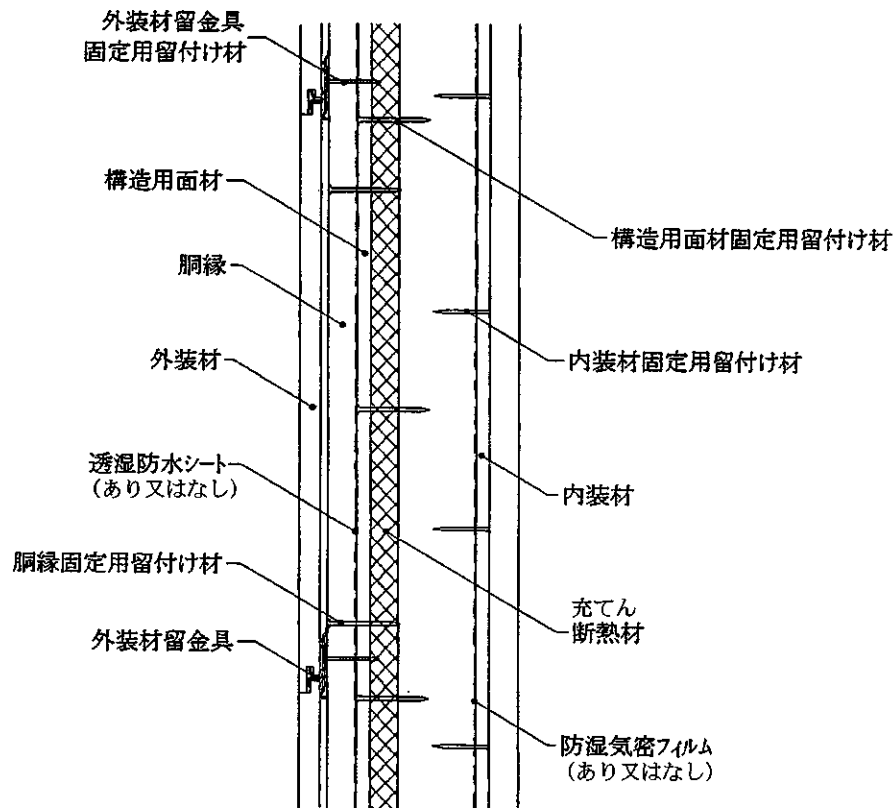
鉛直断面図
