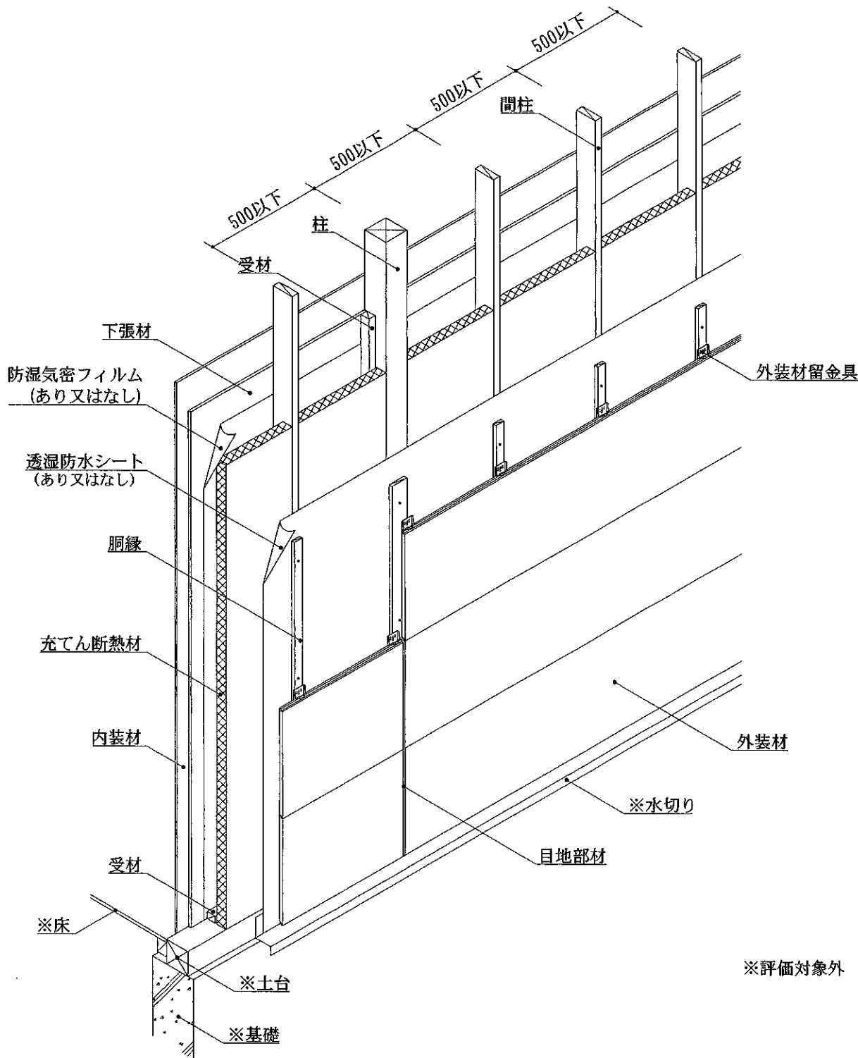
透視図
