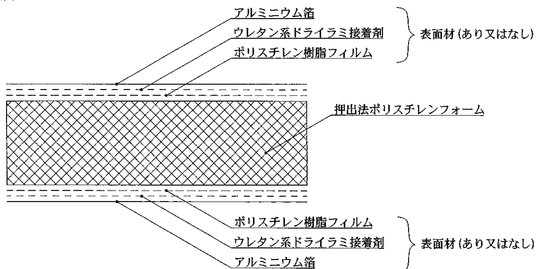
図5 構造説明図
