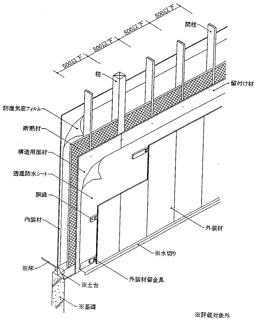
透視図
