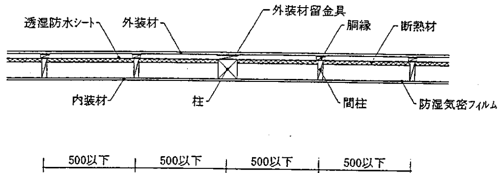
水平断面図
