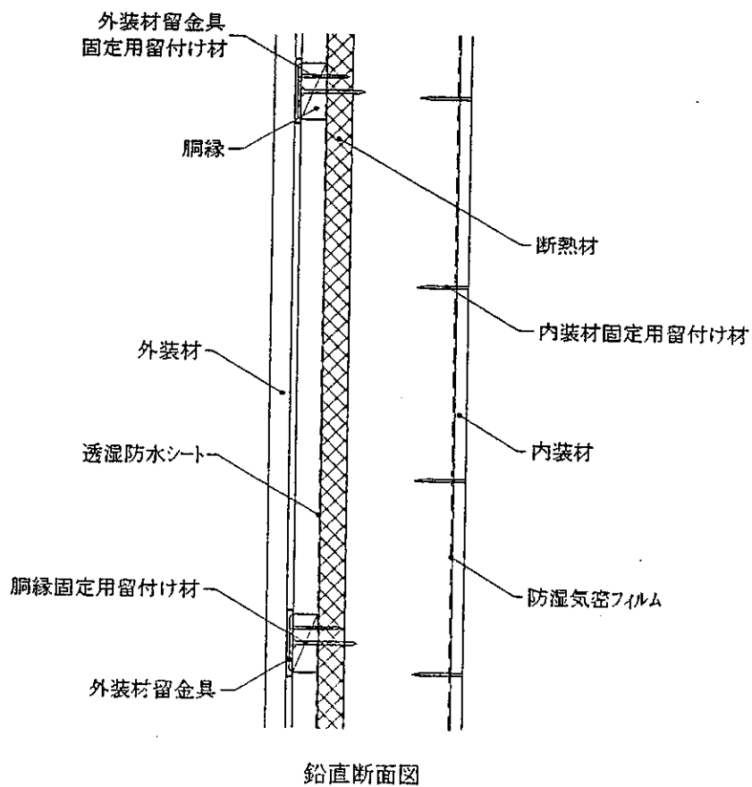
図 2 2 構造説明図
