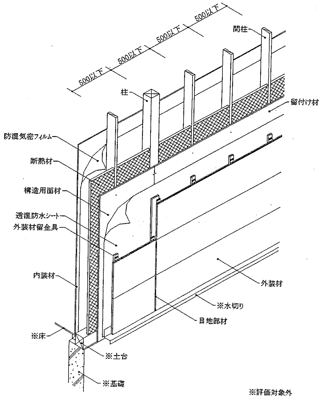
透視図
