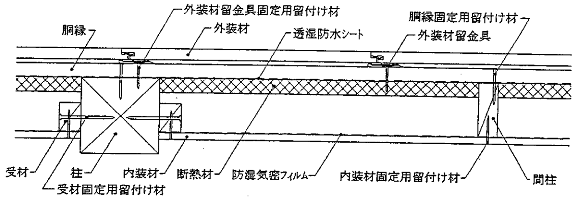
水平断面図
