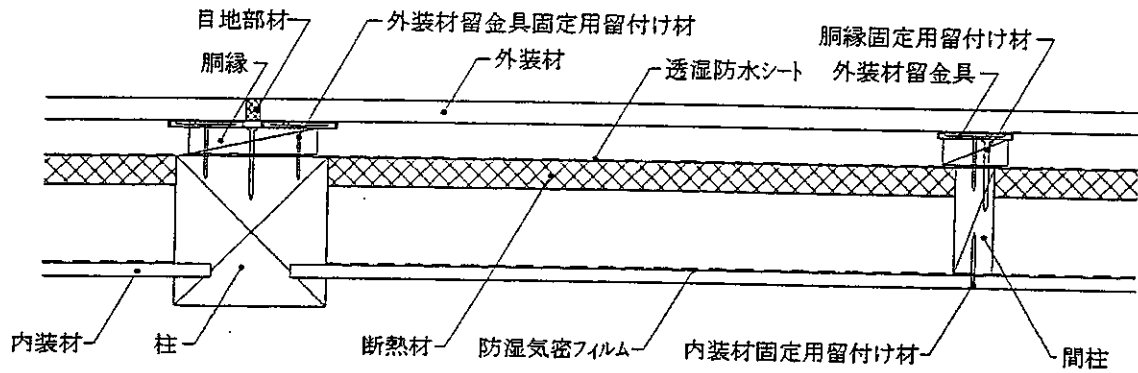
水平断面図
