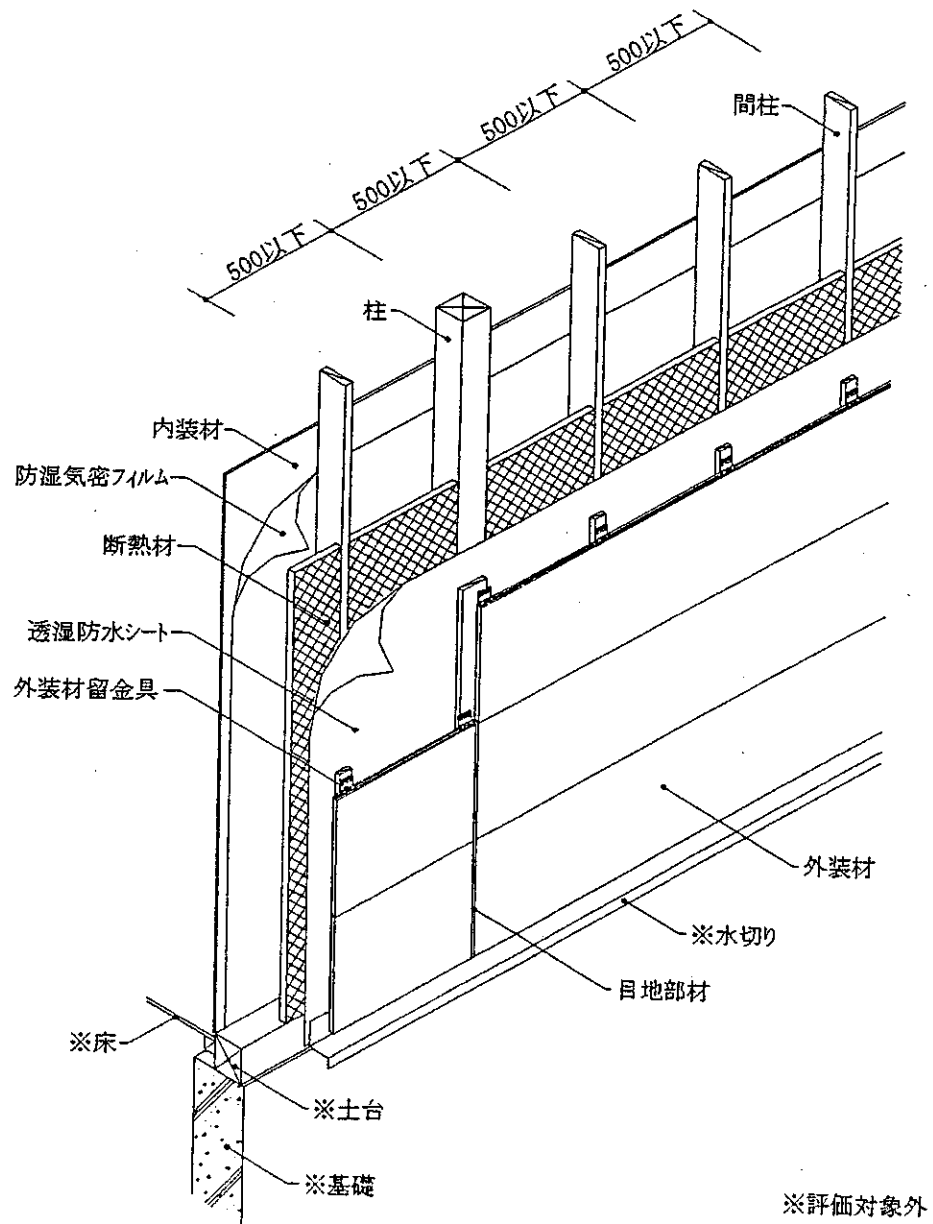
透視図
