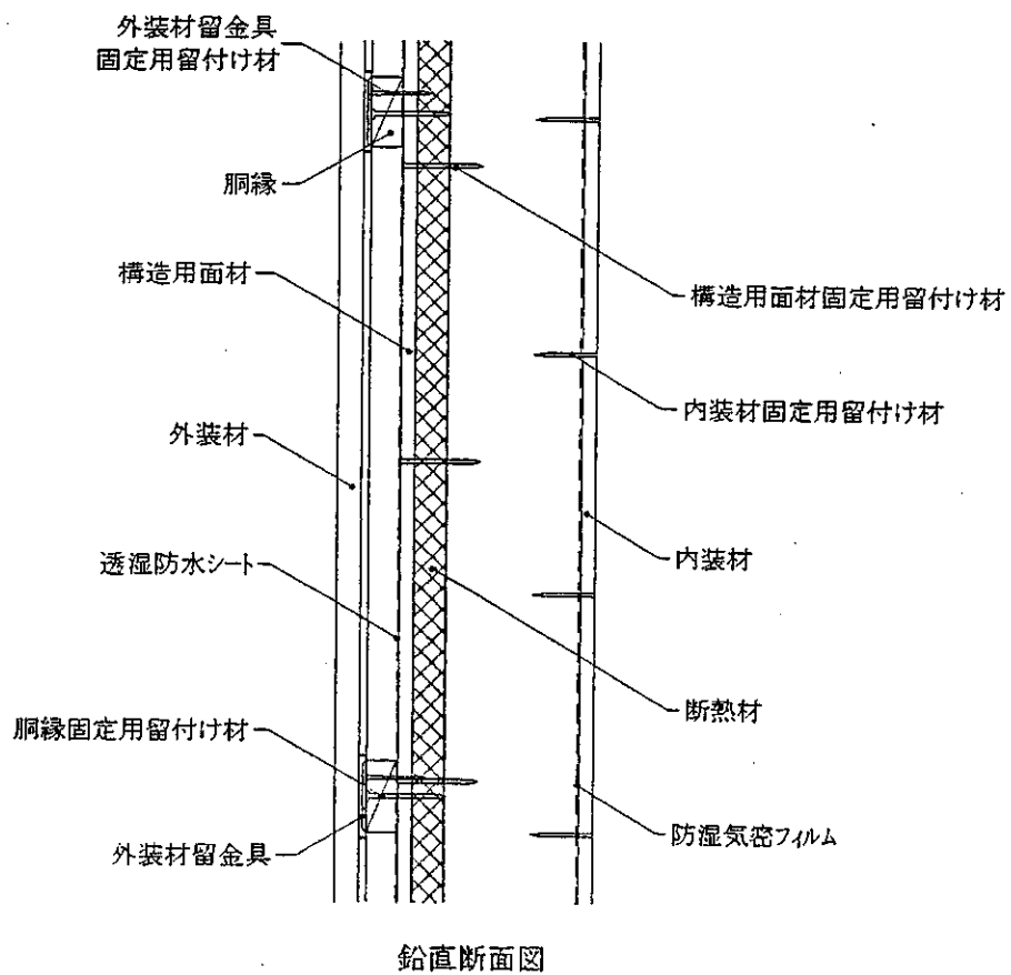
図 2 4 構造説明図
