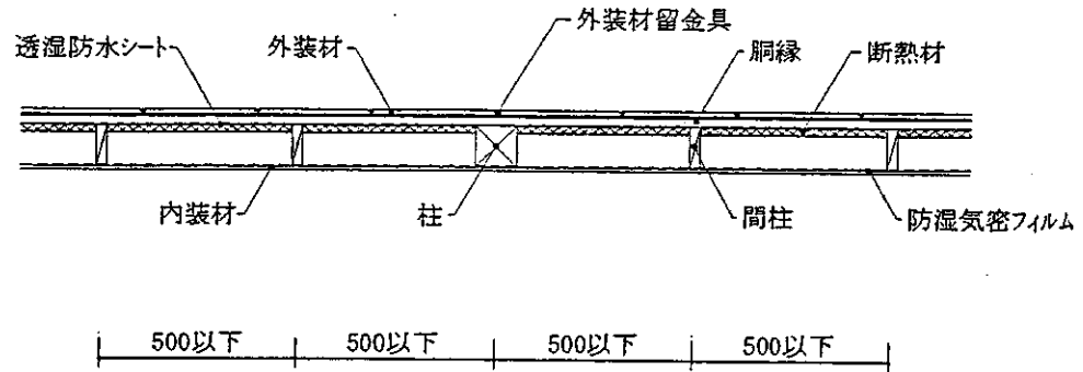
水平断面図
