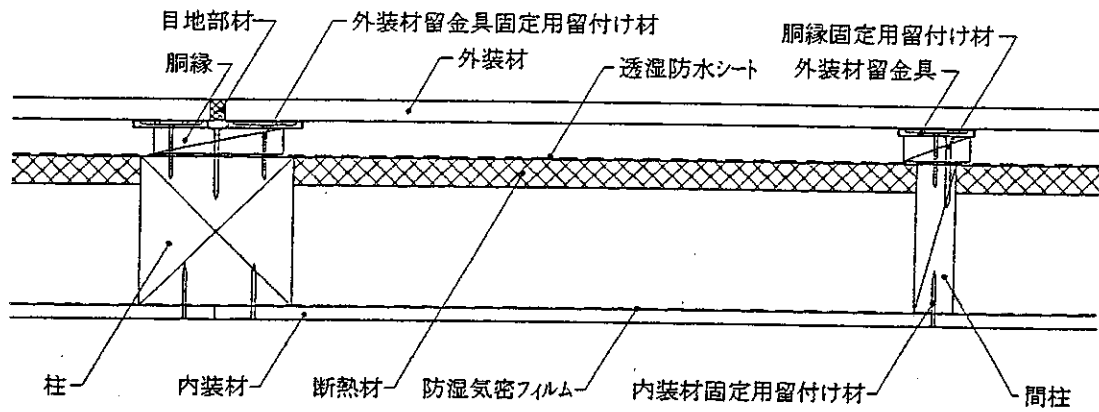
水平断面図
