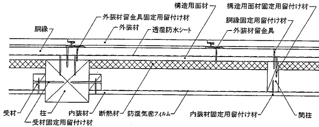
水平断面図
