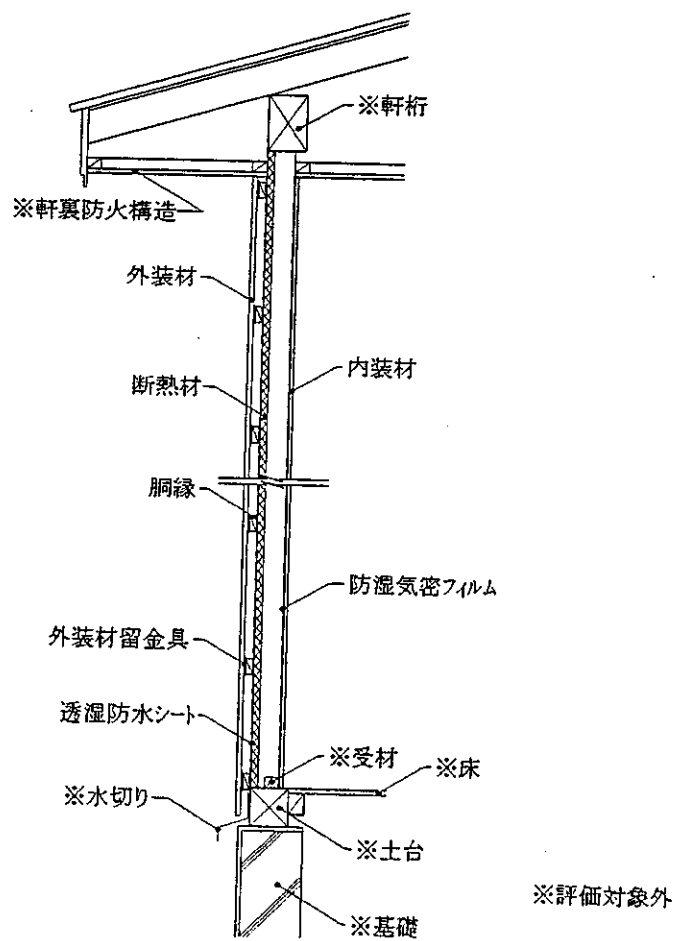
鉛直断面図
