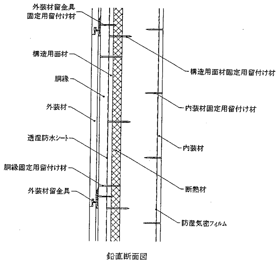
図 2 3 構造説明図
