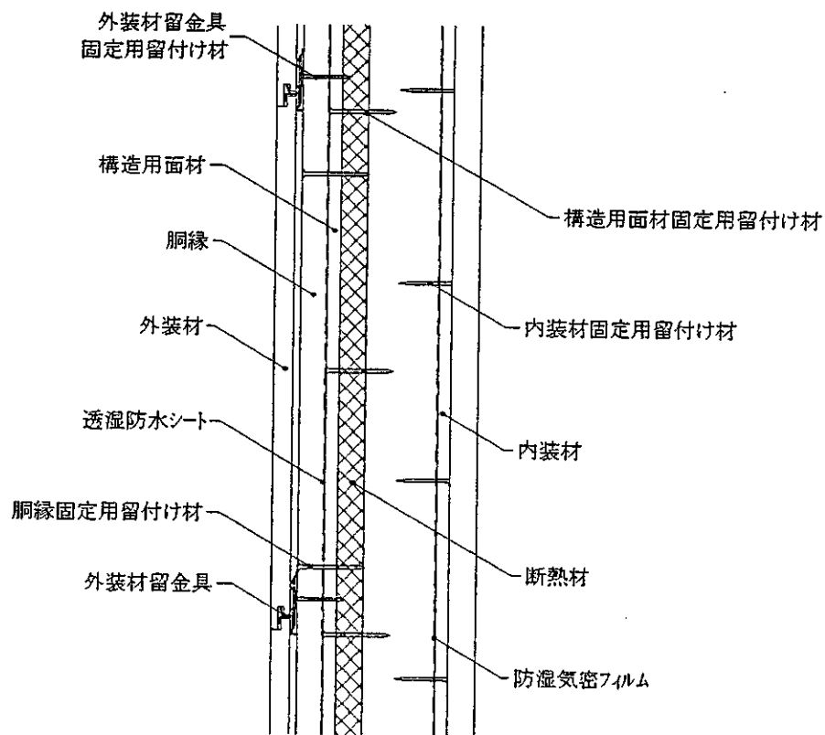
鉛直断面図
