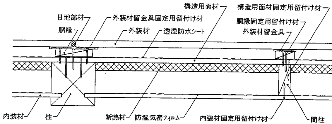
水平断面図
