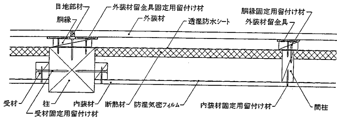
水平断面図
