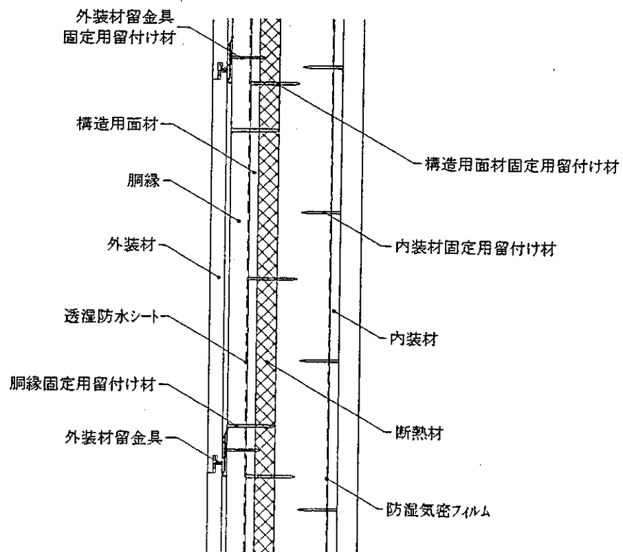
鉛直断面図
