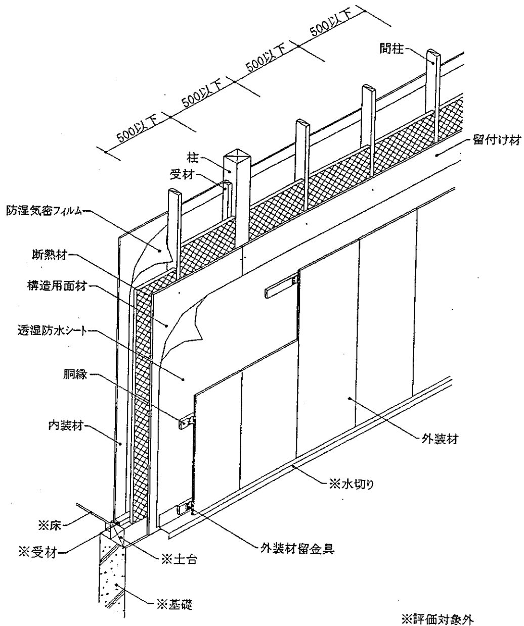
透視図
