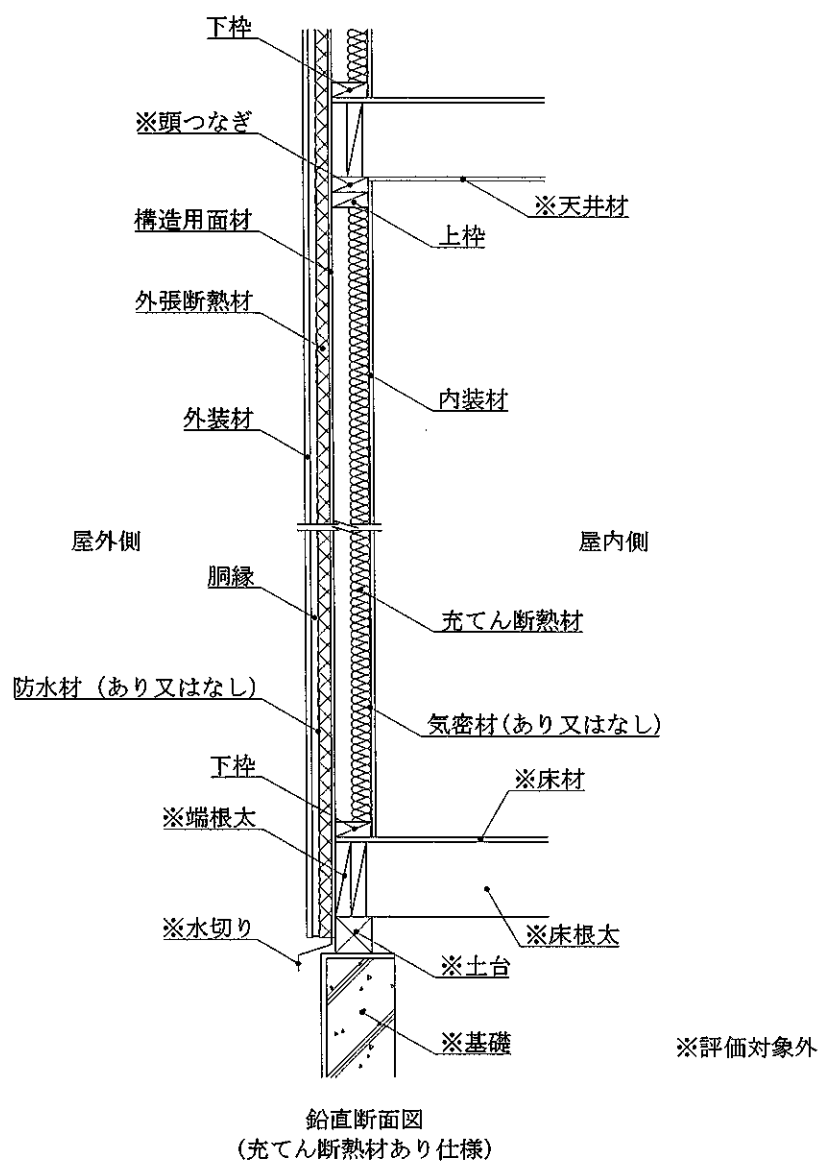
図12 施工図 (外装材縦張／充てん断熱材あり)
