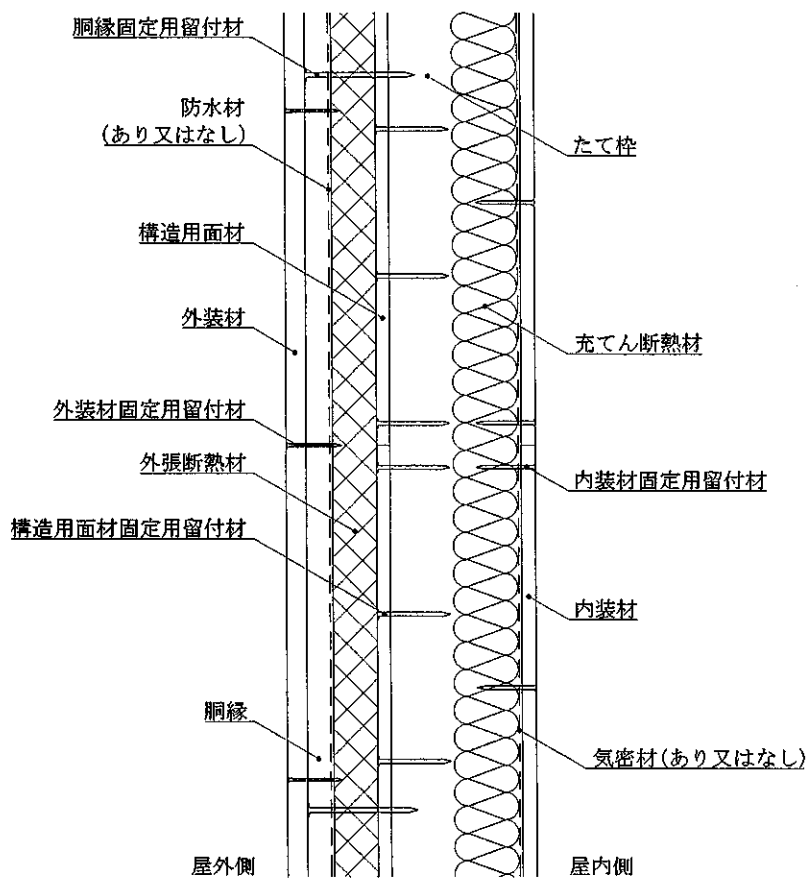
鉛直断面図 (充てん断熱材あり仕様)
