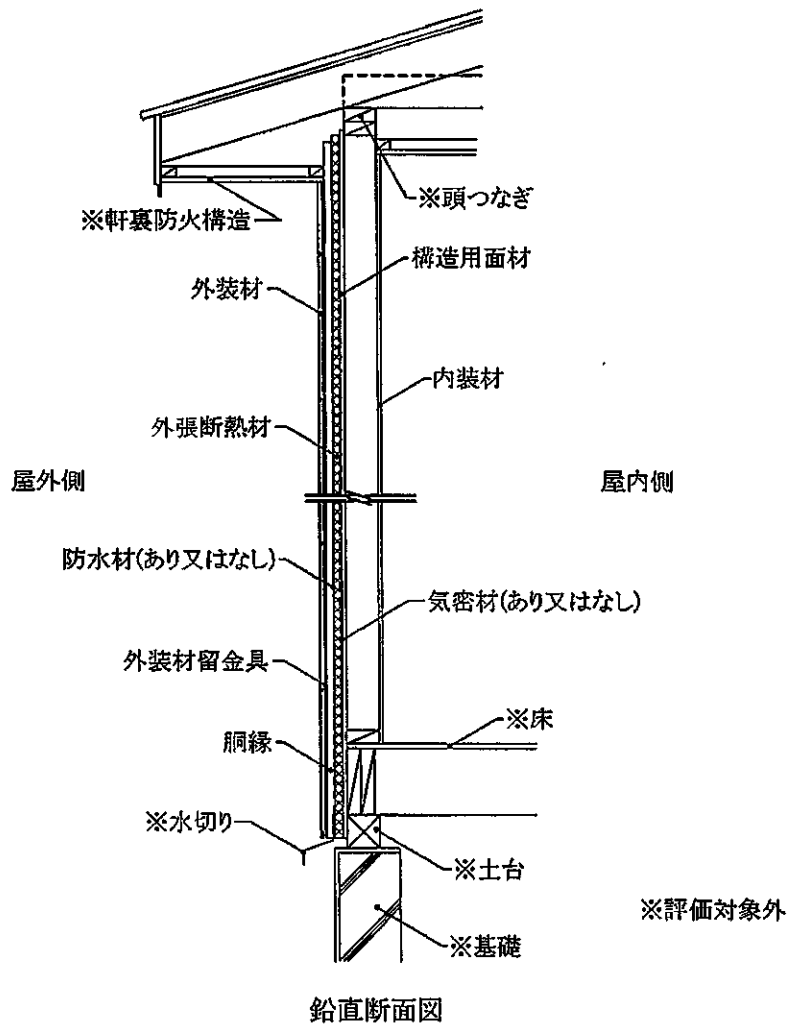
図6 施工図 (外装材横張/充てん断熱材なし)
