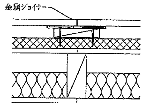
④金属ジョイナー目地
