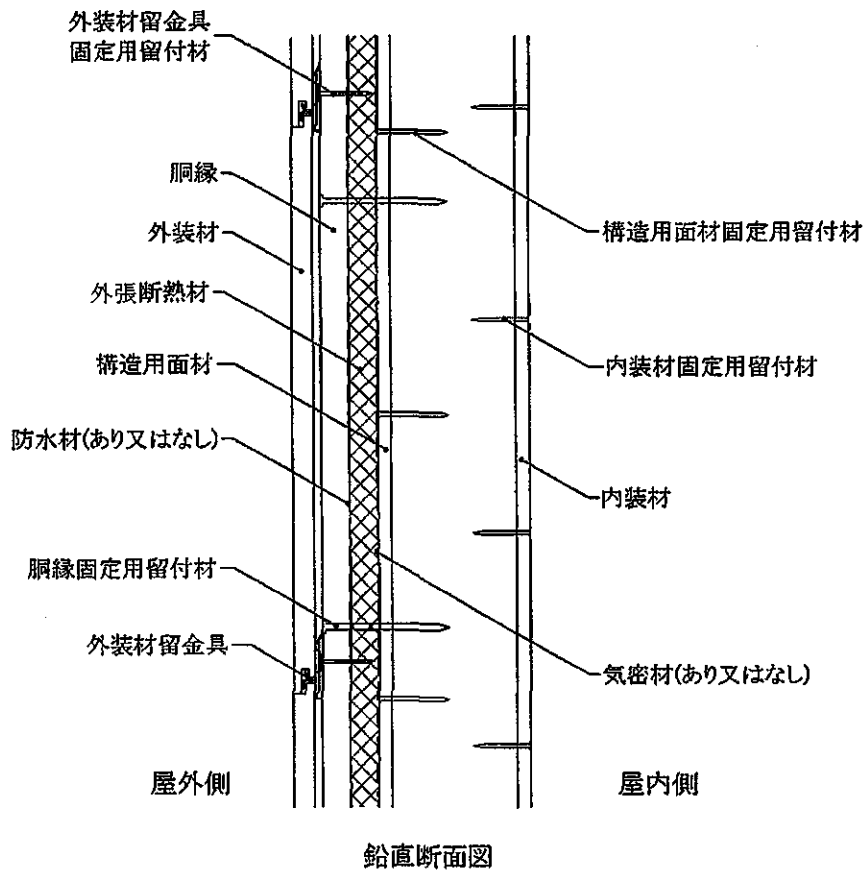
図2 構造説明図 (外装材横張/充てん断熱材なし)
