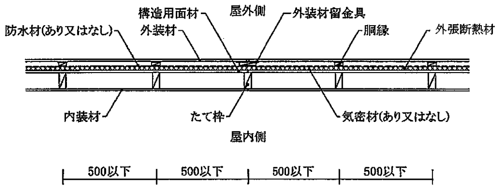
水平断面図
