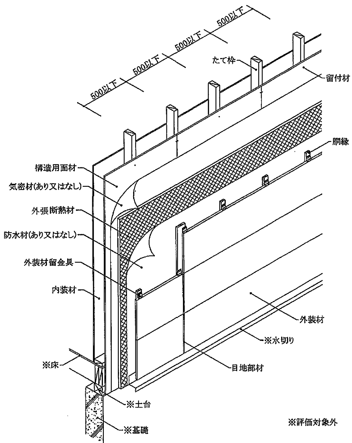
透視図
