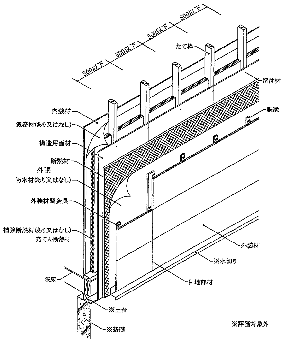
透視図
