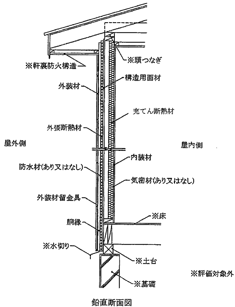
図6 施工図 (外装材横張／充てん断熱材あり)
