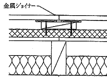
④金属ジョイナー目地
