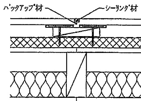
③バックアップ材+シーリング目地
