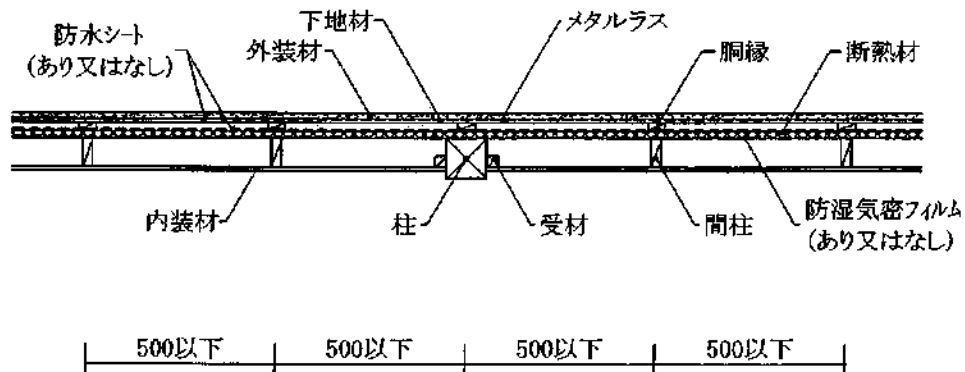
水平断面図
