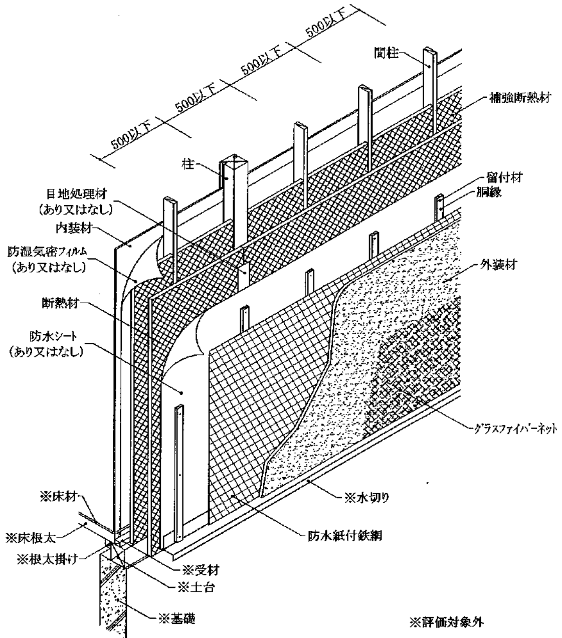
透視図
