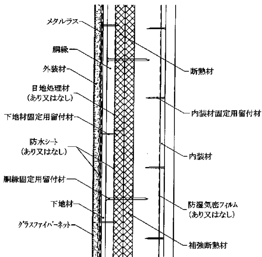
鉛直断面図
