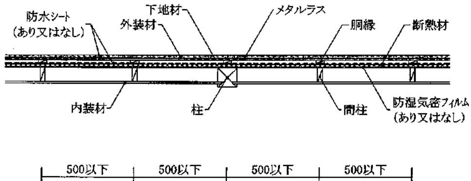
水平断面図
