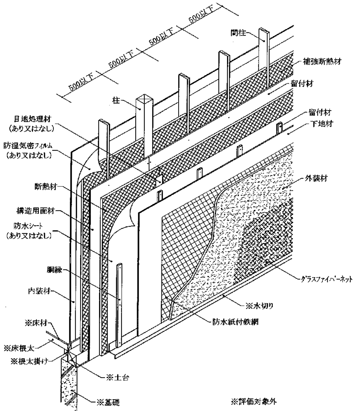
透視図
