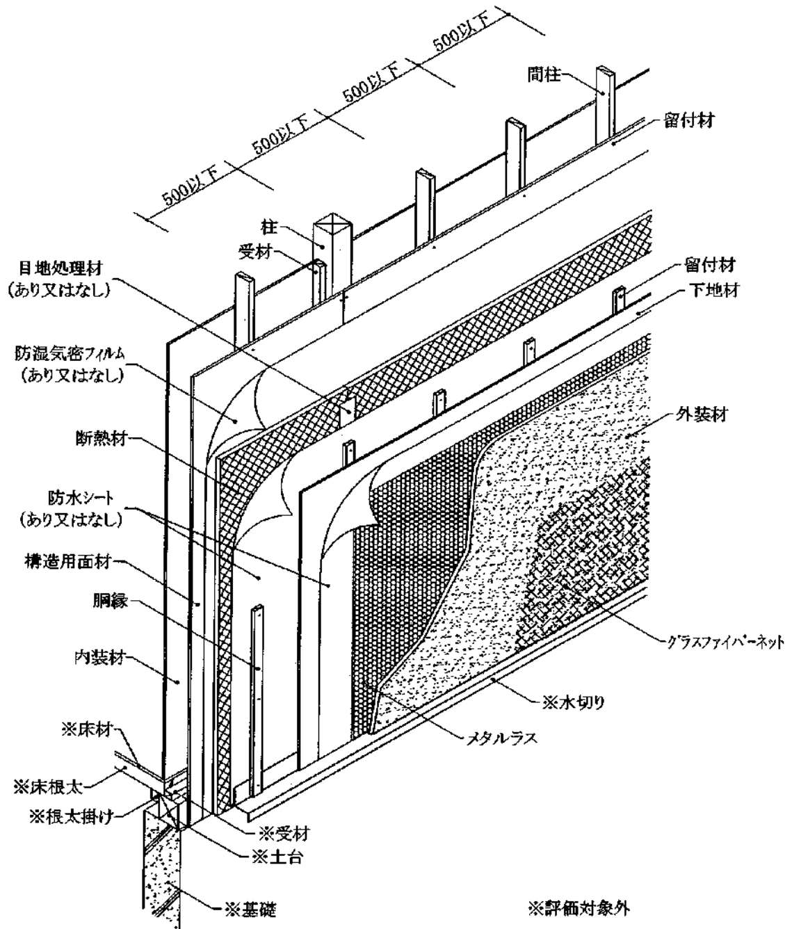
透視図
