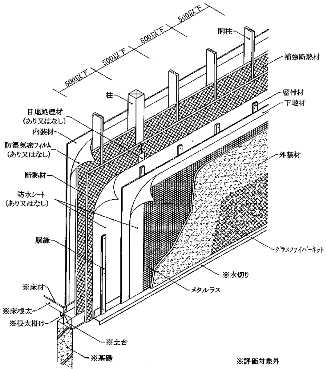
透視図
