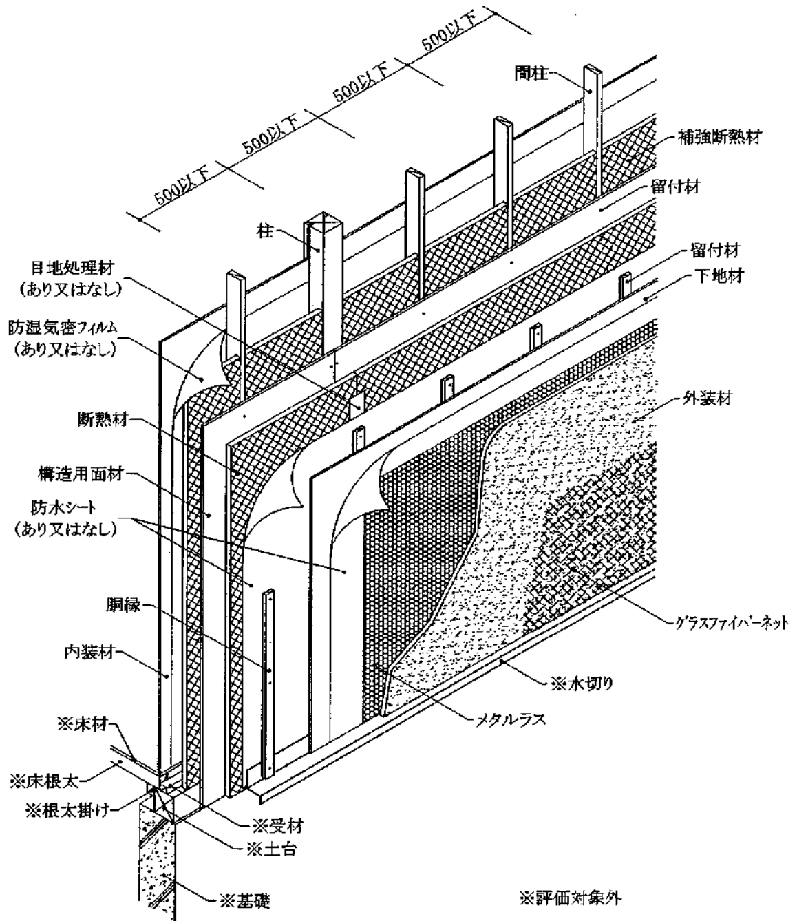
透視図
