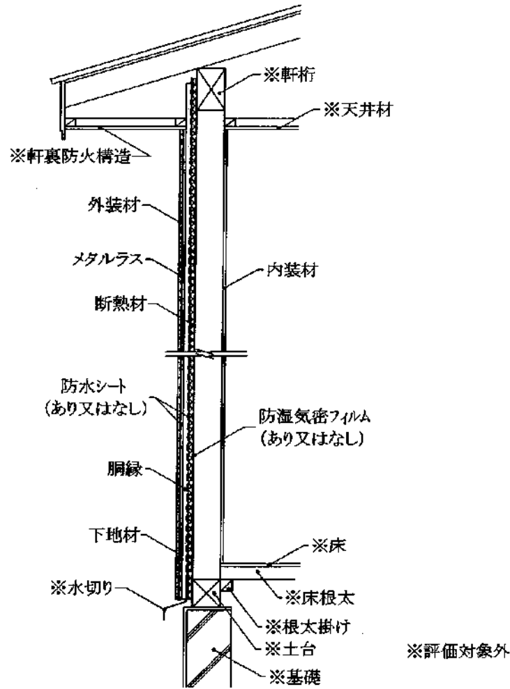
鉛直断面図
