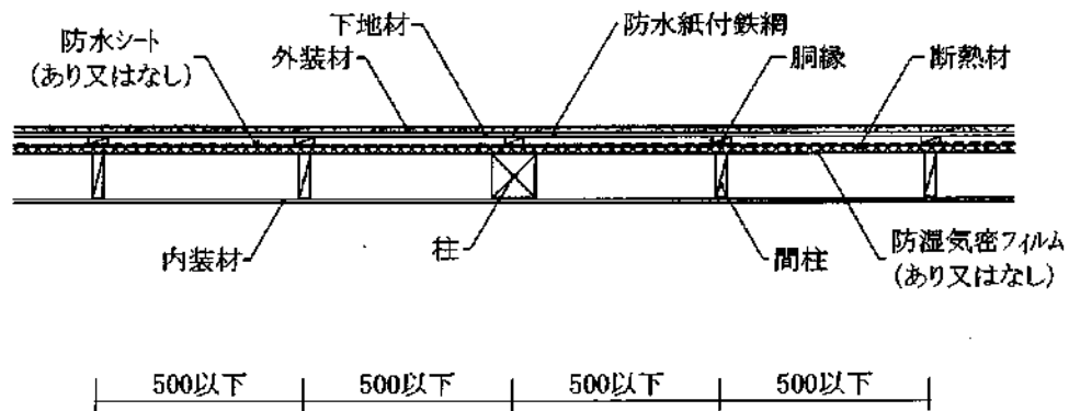
水平断面図
