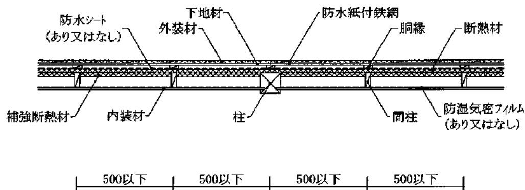
水平断面図
