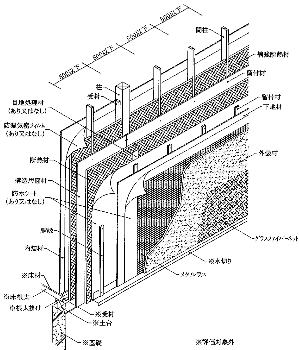
透視図
