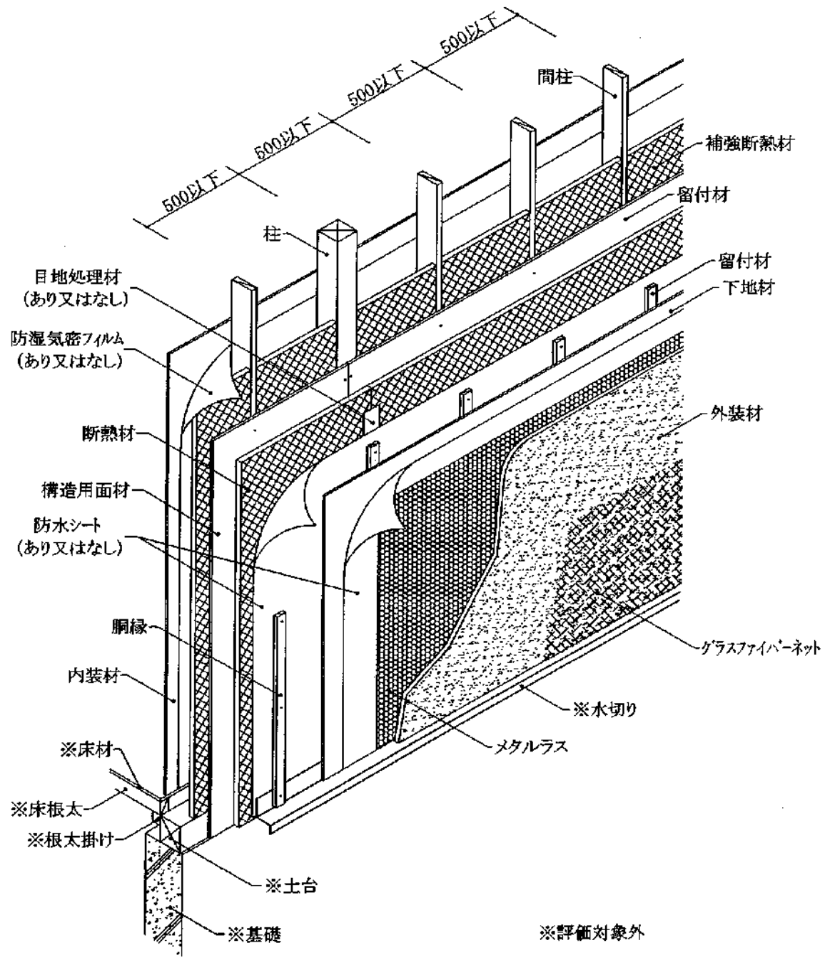
透視図
