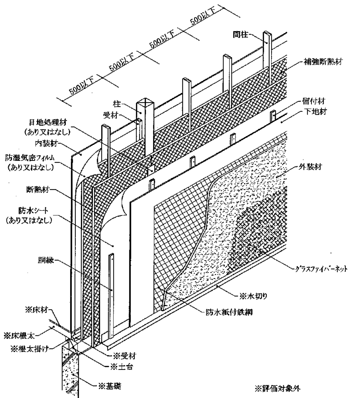
透視図
