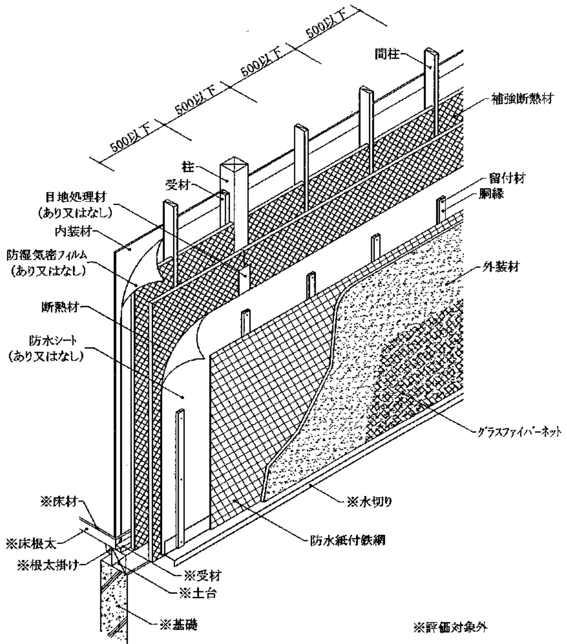
透視図
