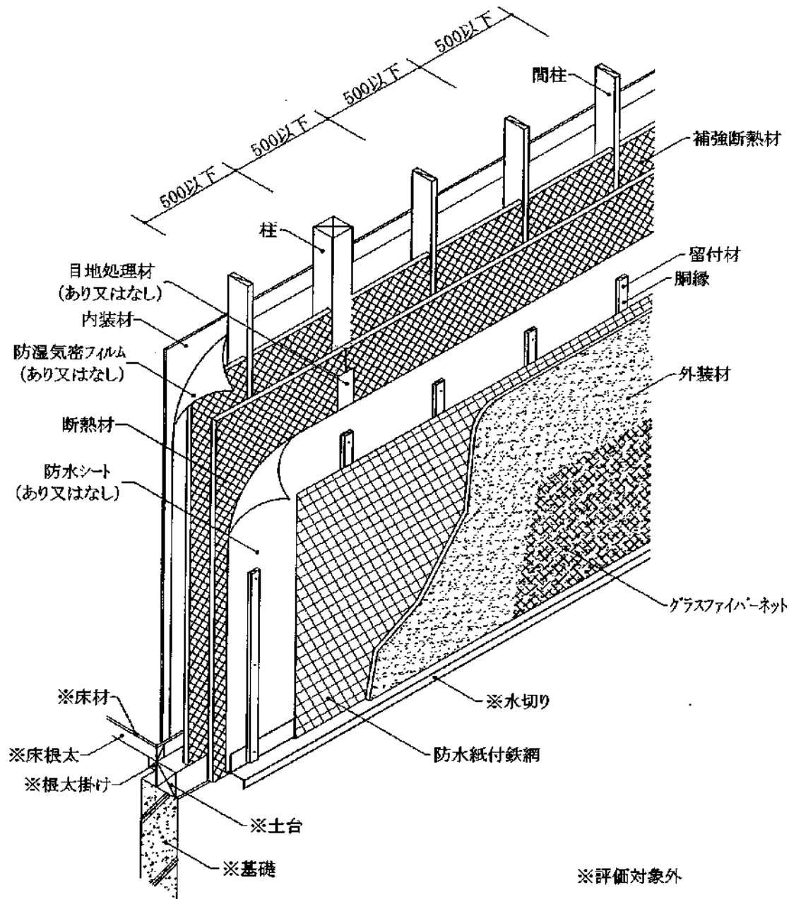
透視図
