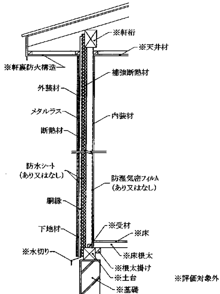
鉛直断面図
