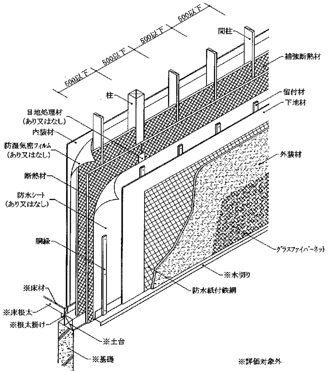
透視図
