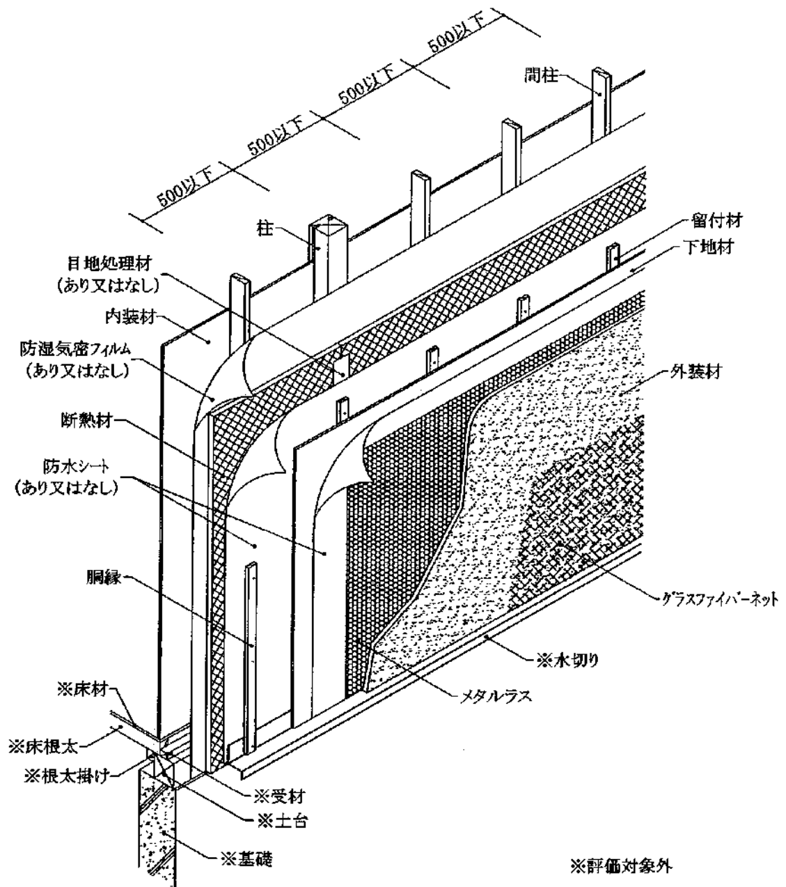
透視圖
