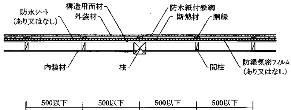
水平断面図
