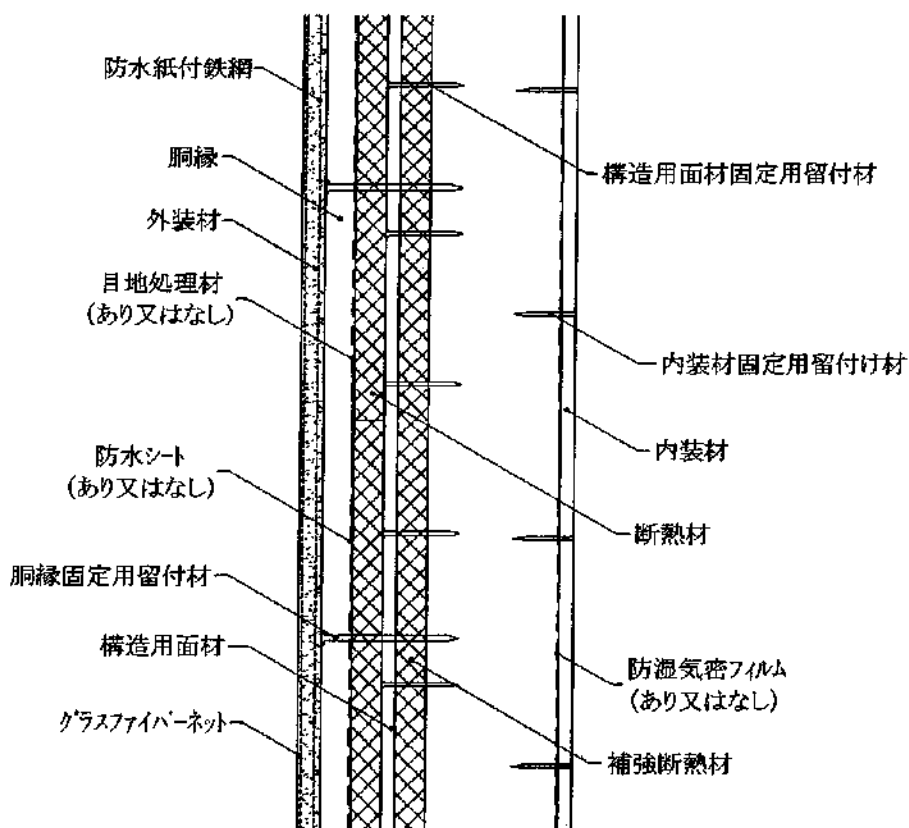
鉛直断面図
