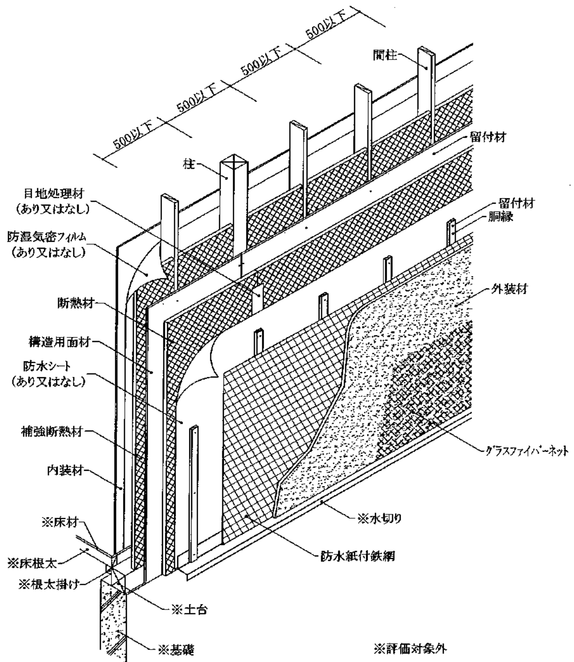
透視図
