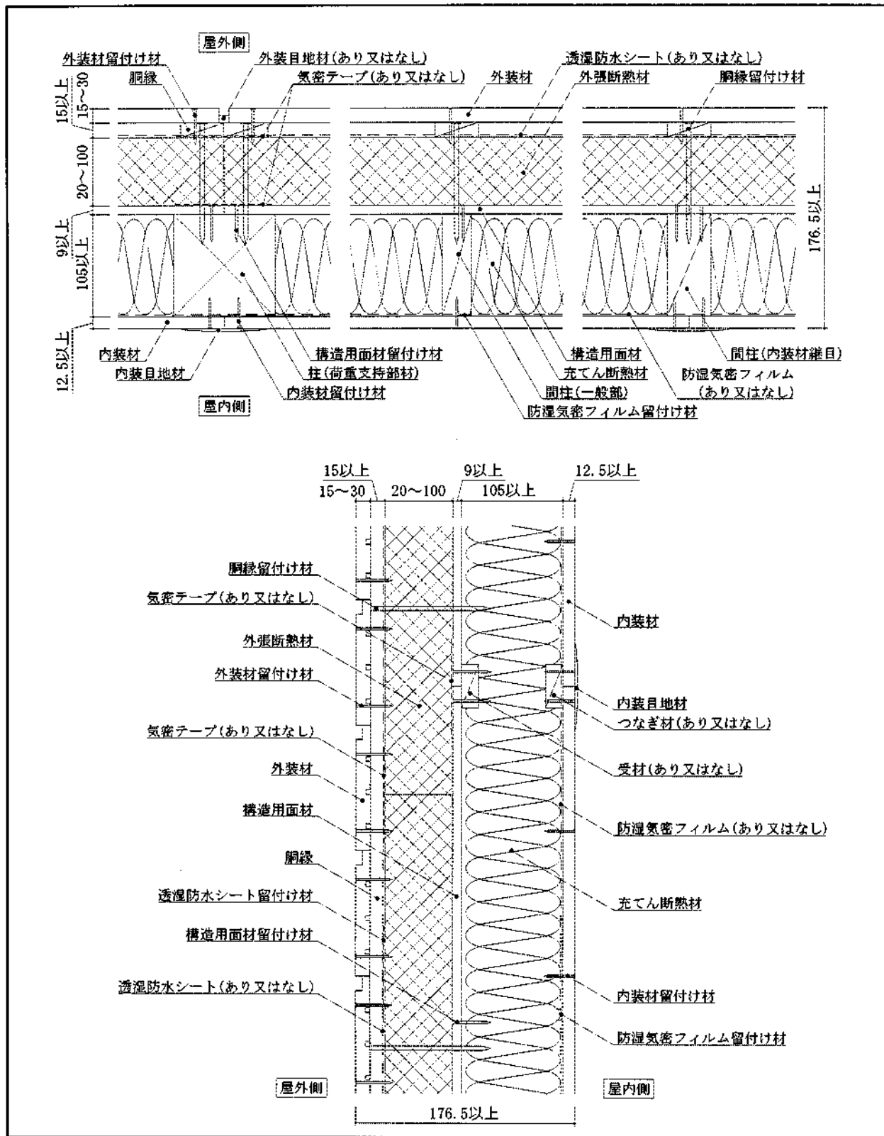
図2 構造説明図
