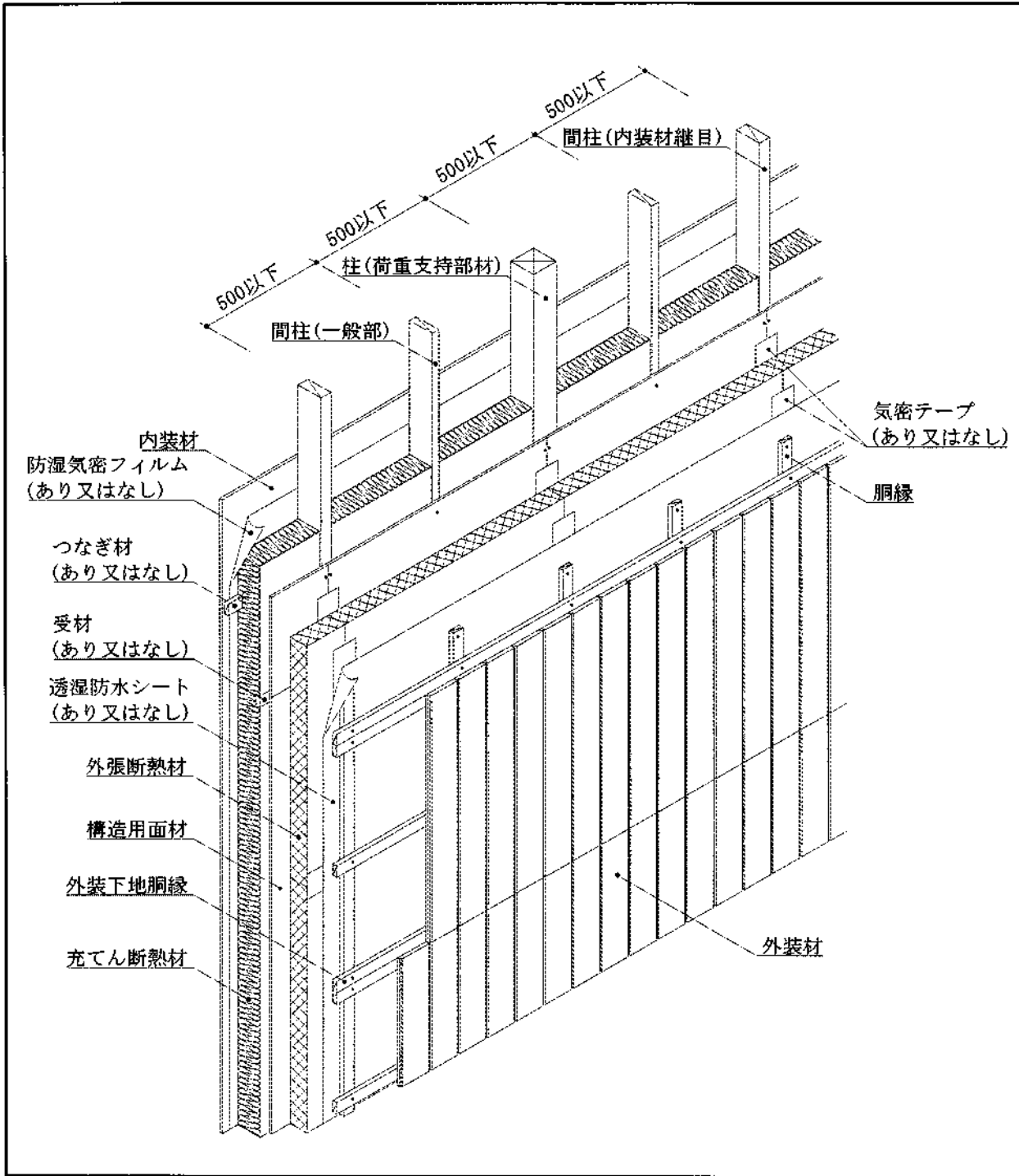
外装材：縦張りの場合（外装下地胴縁あり）
