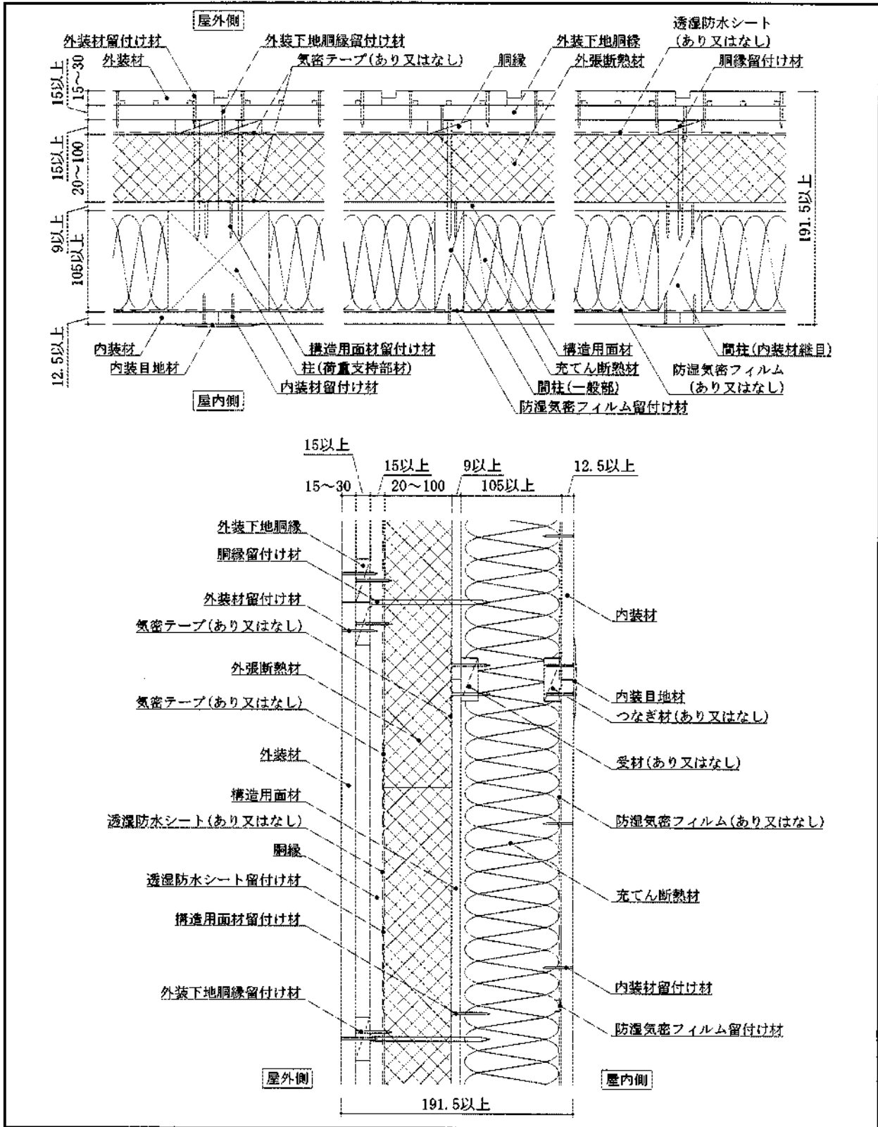
図6 構造説明図
