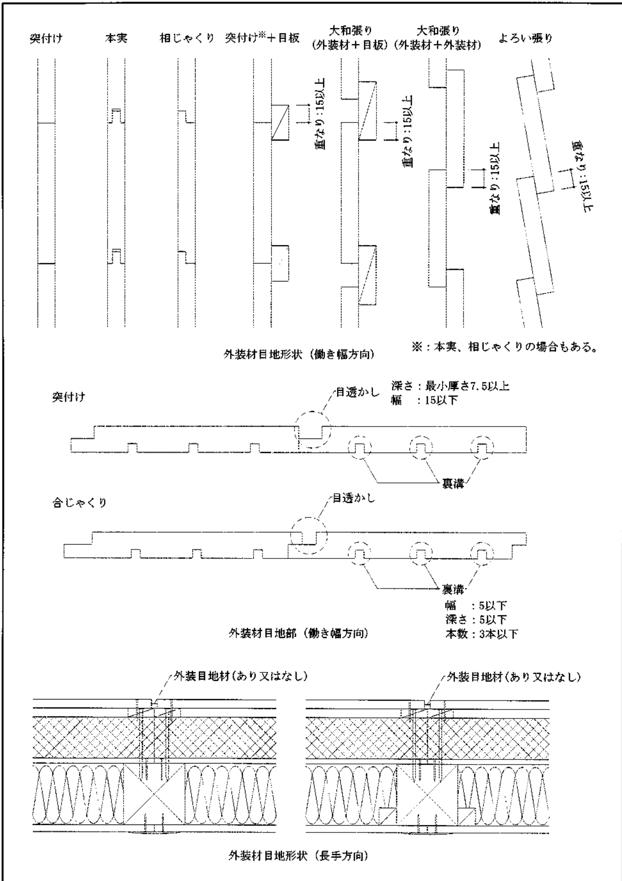
図7 構造説明図
