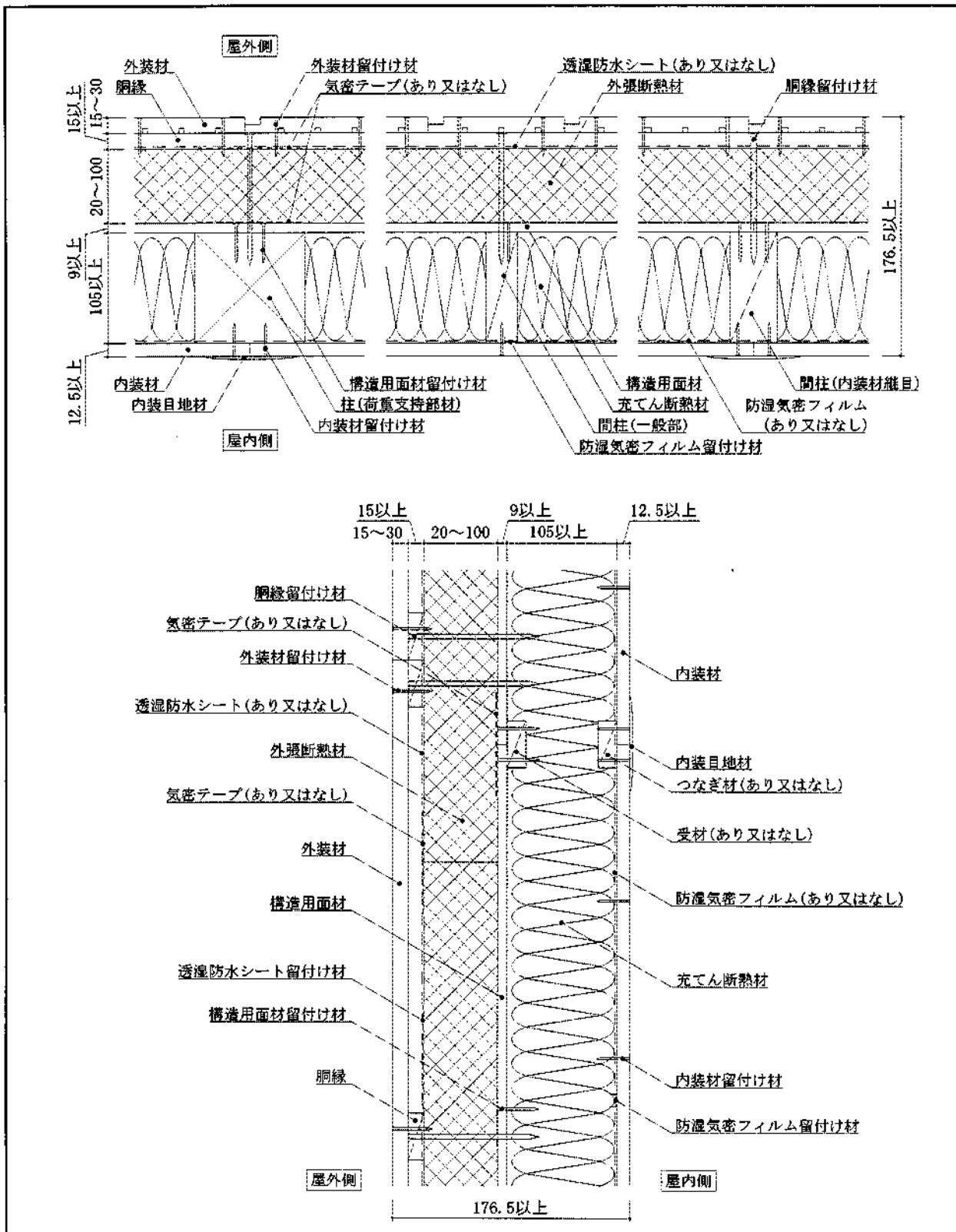
図4 構造説明図
