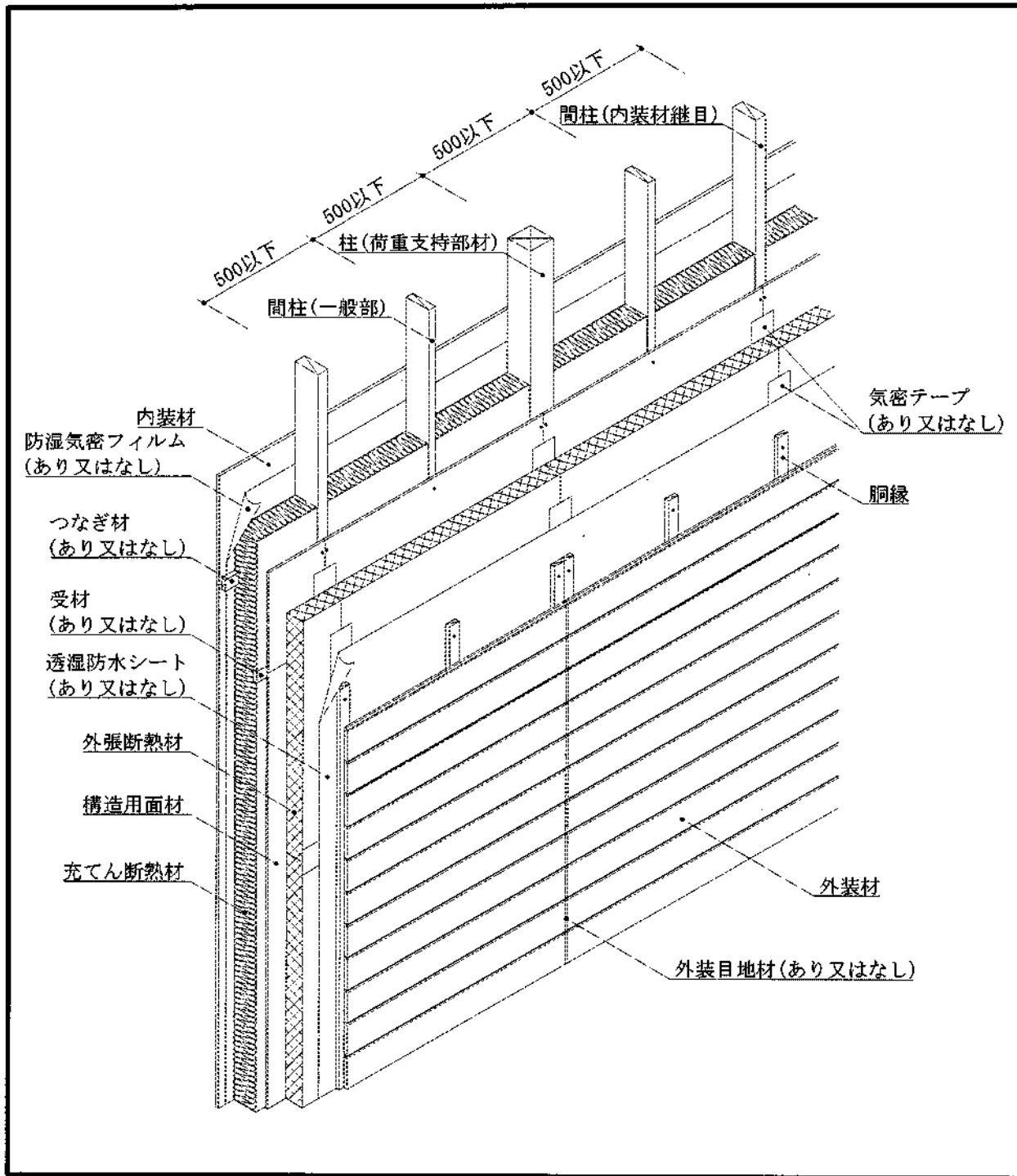
図1 構造説明図
