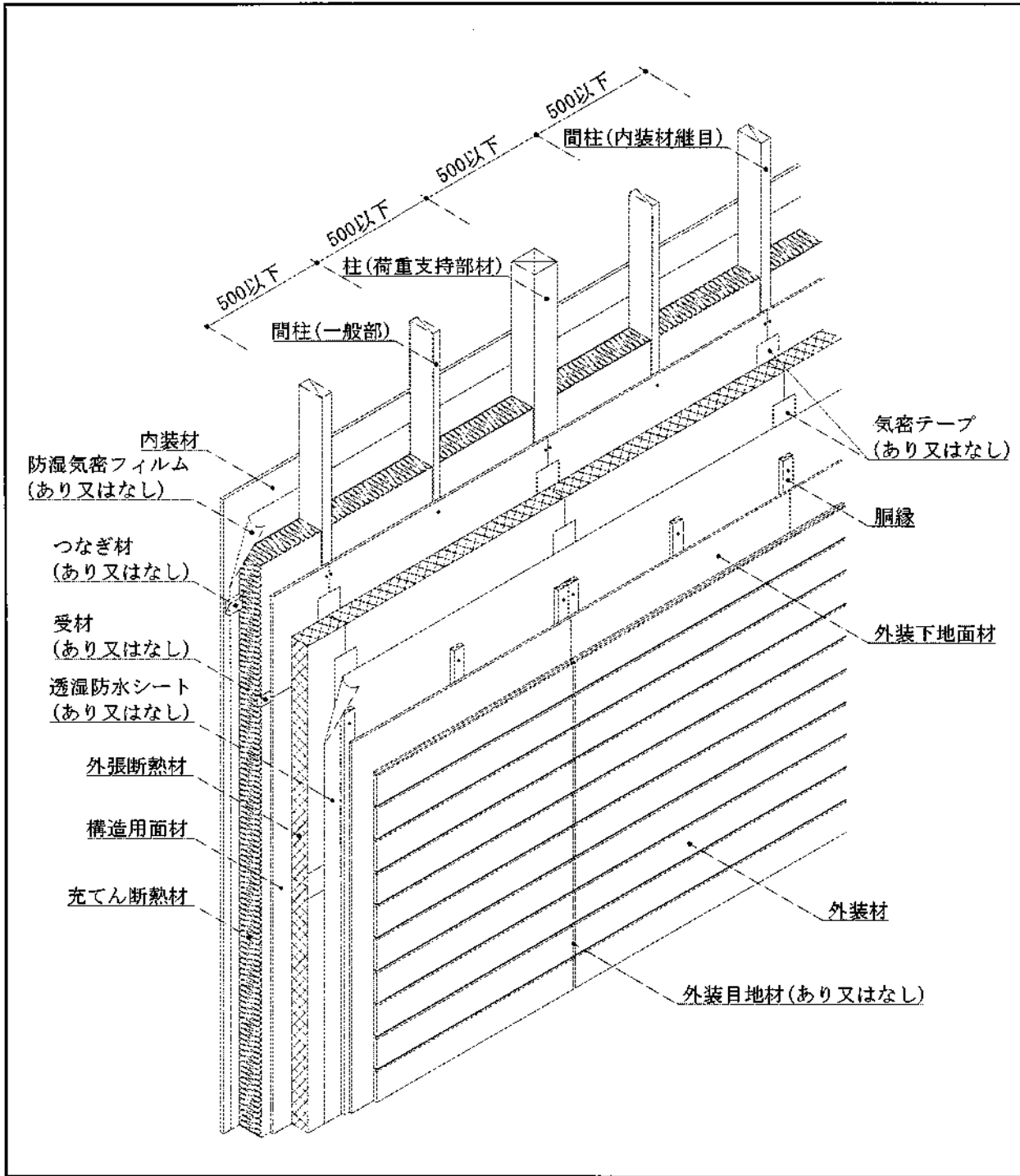
図1 構造説明図
