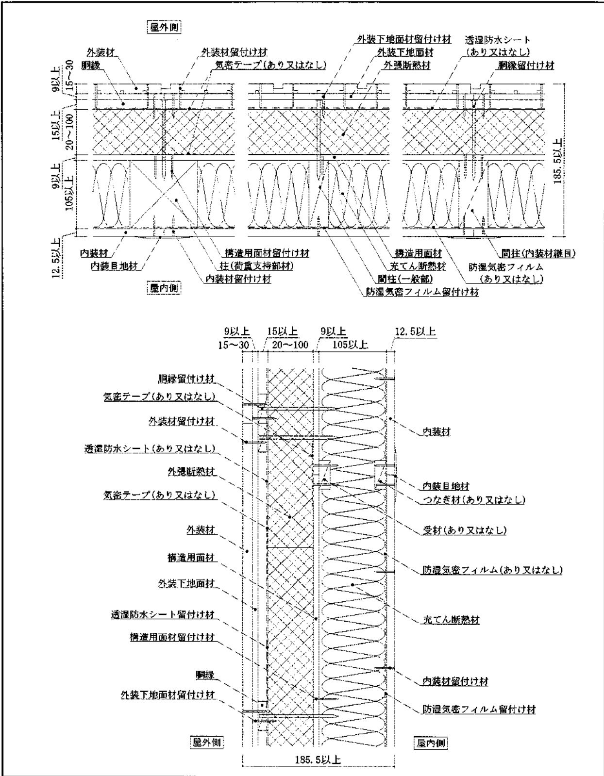
図4 構造説明図
