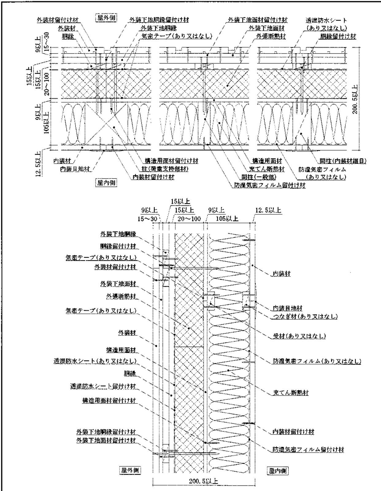
図6 構造説明図
