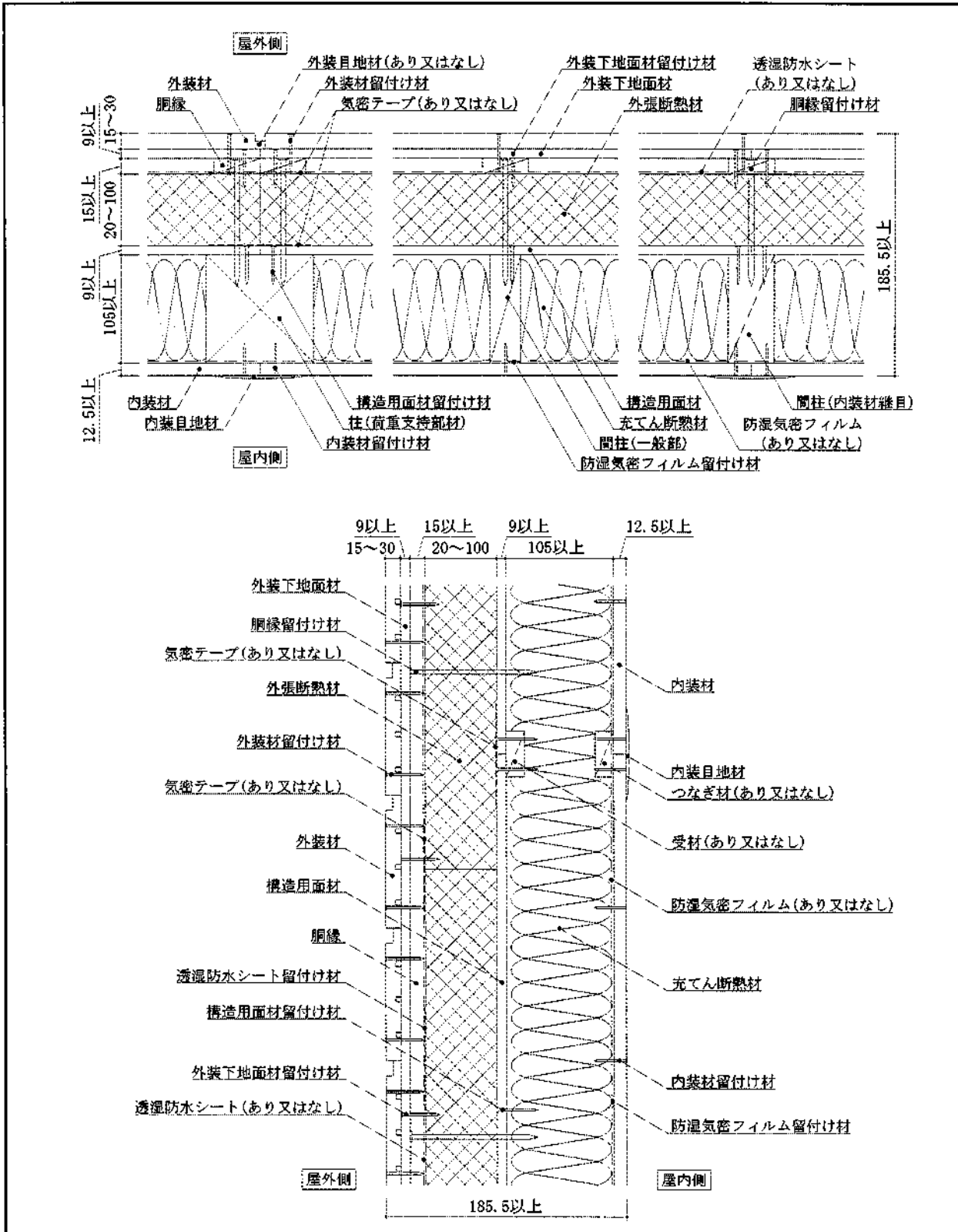
図2 構造説明図
