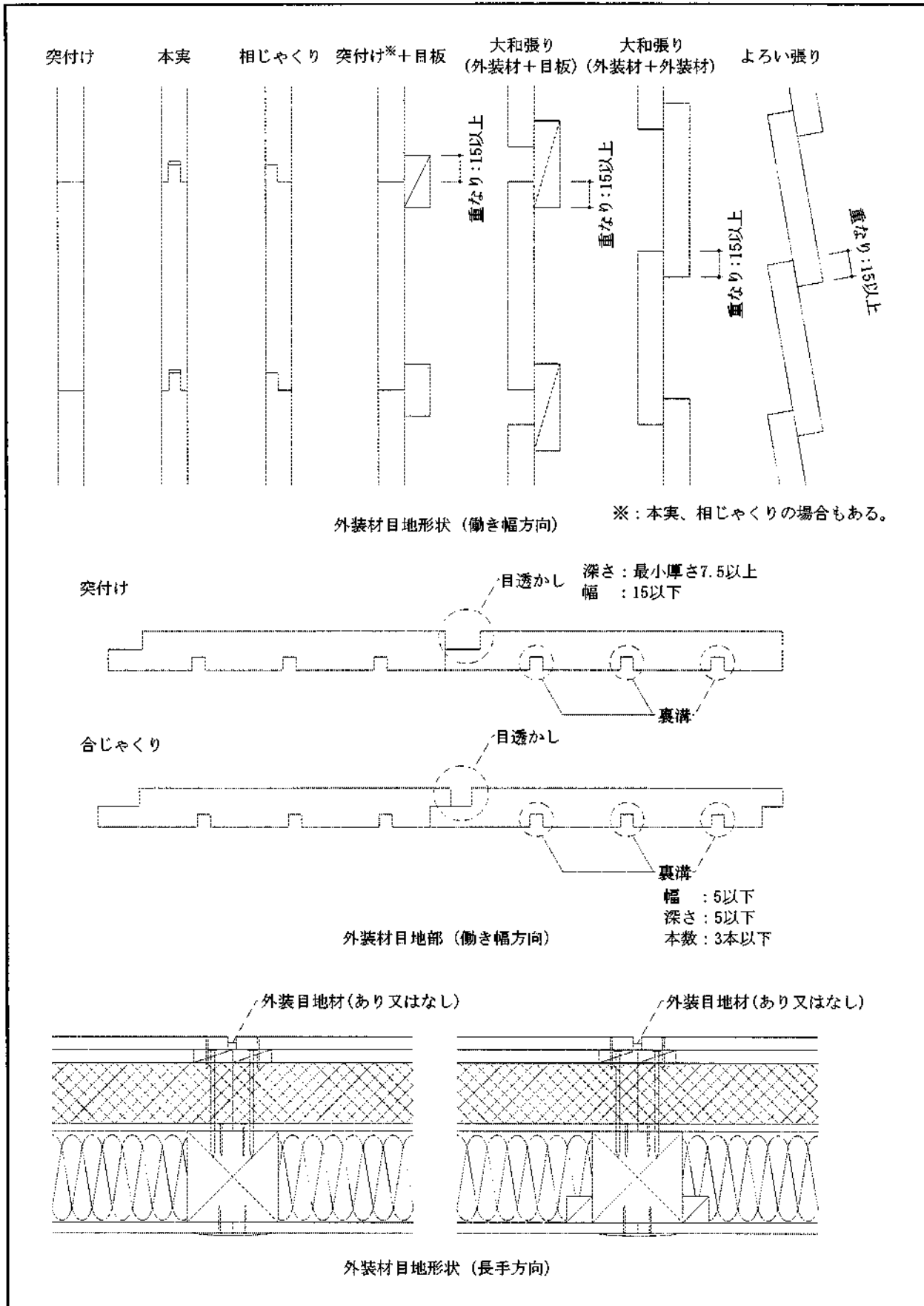
図7 構造説明図
